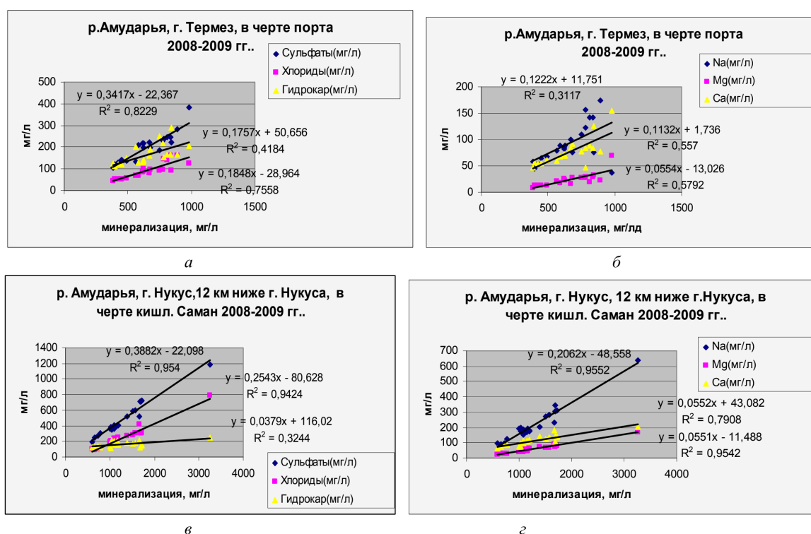
Рисунок 3 – Графики зависимости содержания главных ионов ( \text{Ca}^{2+} , \text{Mg}^{2+} , \text{Na}^+ , \text{HCO}_3^- , \text{Cl}^- , \text{SO}_4^{2-} ) от величины минерализации на различных створах р. Амударья
