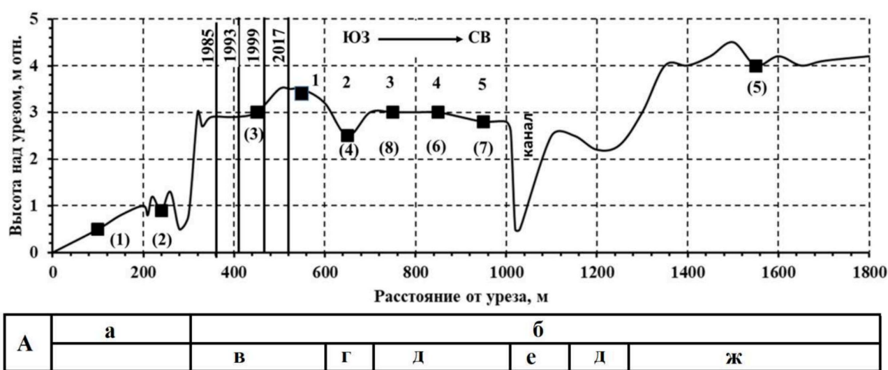
Рис. 2. Топо-экологический профиль близ возвышенности Порлытау. Условные обозначения. Точки в скобках заложены: (1)-(5) – в 1979 г., (6)-(7) – в 1993 г., (8) – в 2017 г.; 1-4 – номера точек в таблице 2 и на рисунке 3; вертикальные линии и год – положение берегового обрыва реки в конкретном году. А – рельеф: а – современная прирусловая пойма р. Амударьи; б – исторический прирусловой вал р. Амударьи; в – современный прирусловой вал; г – наложенное современное русло протоки на пологом склоне прируслового вала; д – пологий склон современного прируслового вала; е – антропогенный с/х канал на обсохшем склоне прируслового вала; ж – мелкогребистая поверхность, сформированная системой более поздних наложенных проток на погребенном выположенном склоне исторического прируслового вала.
