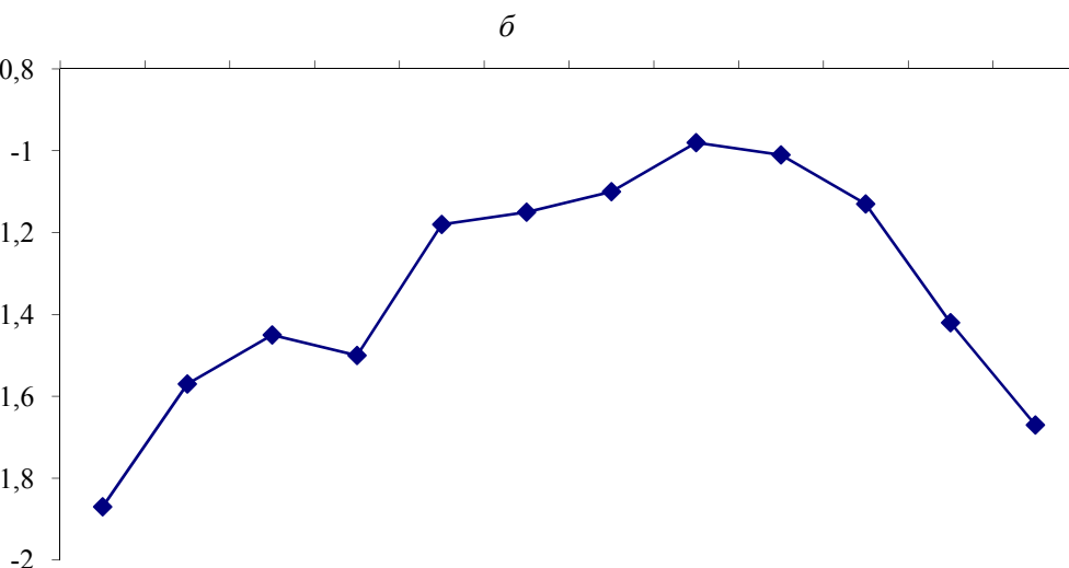
Внутригодовые изменения уровней подземных вод в режимной скважине: a – за 2001–2006 гг.; б – средних за 2005–2014 гг.
