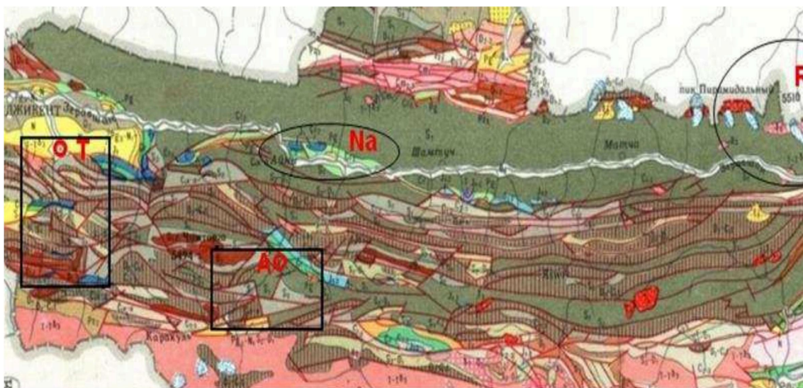
Рис. 1. Геологическая позиция главных источников образования аномальных концентраций макро- и микроэлементов в бассейне реки Зеравшан. Техногенные источники показаны
