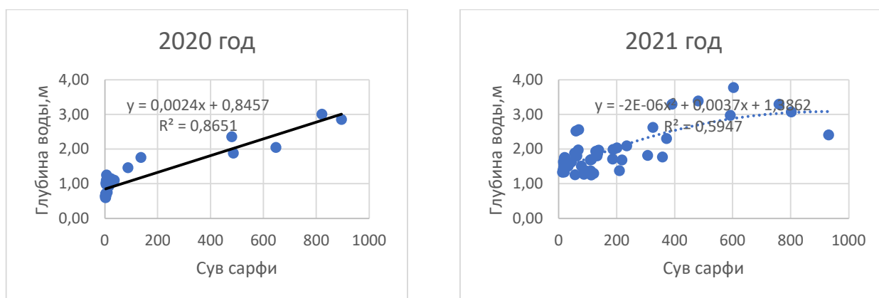
Рисунок 4. Динамика зависимости расхода воды Амударьи от глубины на бесплотинном водозаборе КМК
