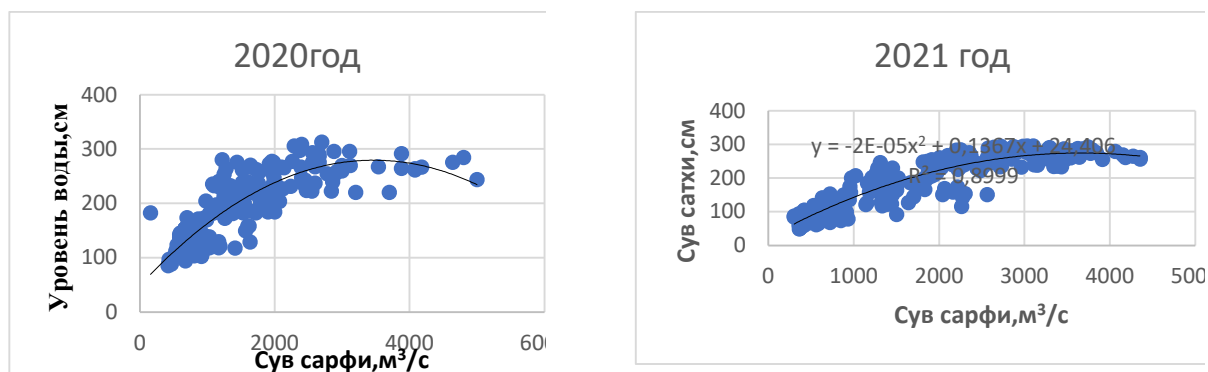
Рисунок 3. Динамика зависимости уровня воды Амударьи от расхода на бесплотинном водозаборе КМК
