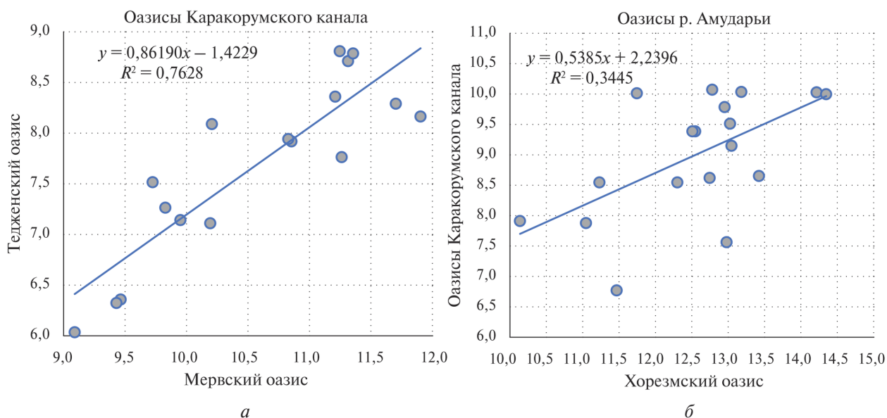
Рис. 4. Взаимосвязь между значениями ICE оазисов р. Амударьи в период 2003–2020 гг.: a — оазисы среднего течения реки: Мервский против Тедженского; б — оазисы нижнего и среднего течения: Хорезмский против Мервского с Тедженским. Построено на основе данных LST FEWS NET
