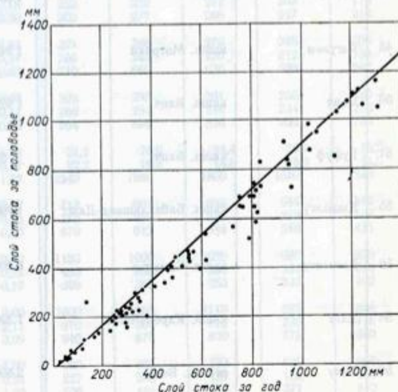
Рис. 59. Связь между нормой стока за половодье и нормой стока за год.
