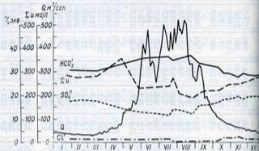
Рис. 114. Внутригодовое изменение расходов воды, минерализации и содержания главных ионов в воде р. Зарафшан у моста Дупули за 1954 г.
