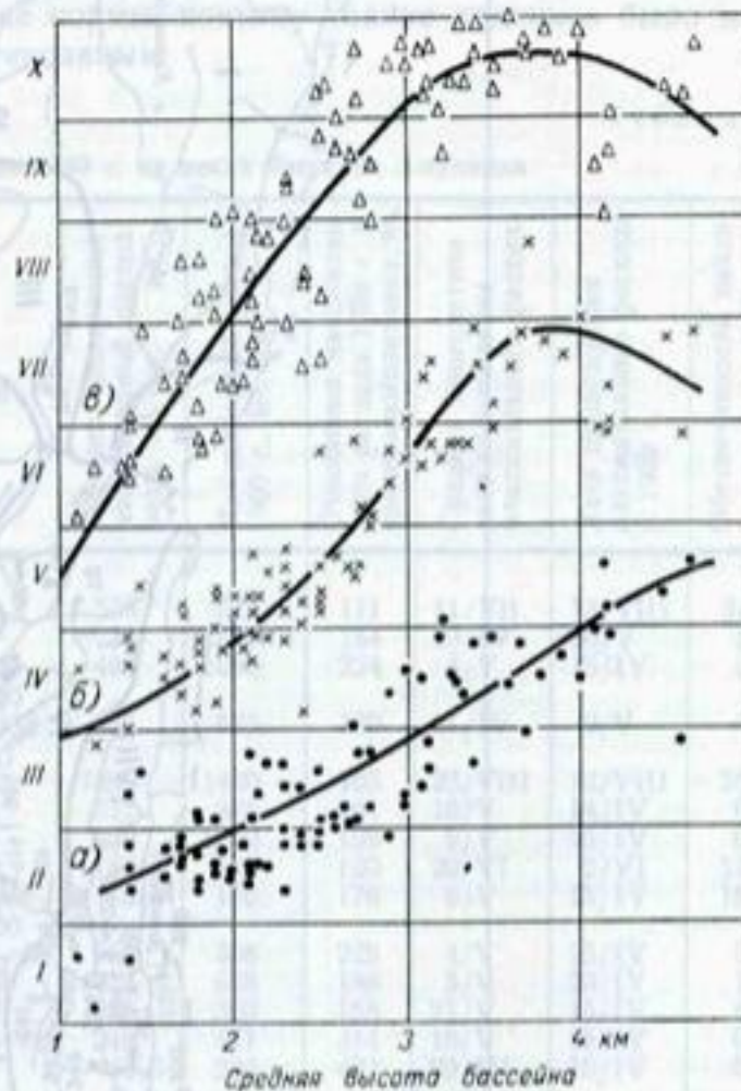
Рис. 55. Зависимость времени прохождения половодья от средней высоты бассейнов.
