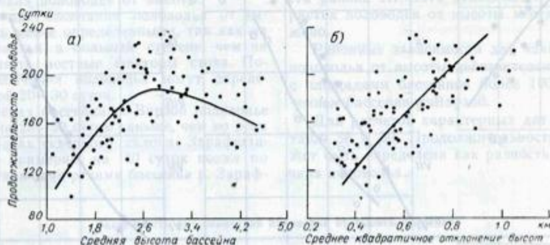
Рис. 56. Зависимость продолжительности половодья от средней высоты бассейнов (а) и среднего квадратичного отклонения высот в бассейне (б).
