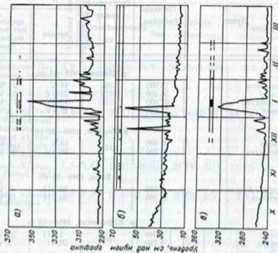
Рис. 38. Ход уровня на реках в период осенне-зимней межени 1955—56 гг., искаженный ледовыми явлениями.
