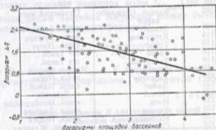
Рис. 64. Зависимость величины дождевой надбавки к максимальным расходам талых вод от площади бассейна.
