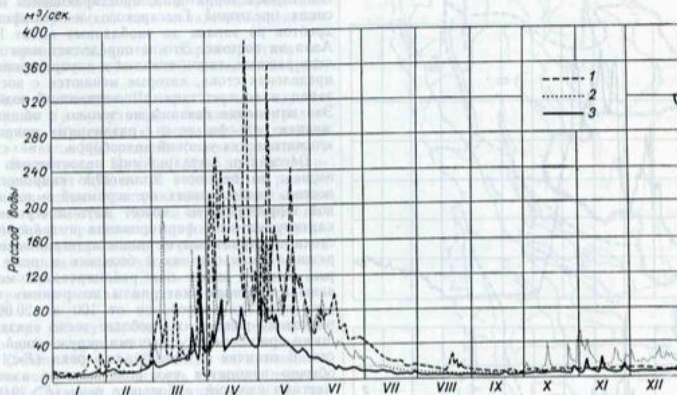
Рис. 33. Гидрограф стока р. Яхсу у кишла. Карбостонак за характерные по водности годы. 1 — многоводный (1949), 2 — средний (1953), 3 — маловодный (1947).
