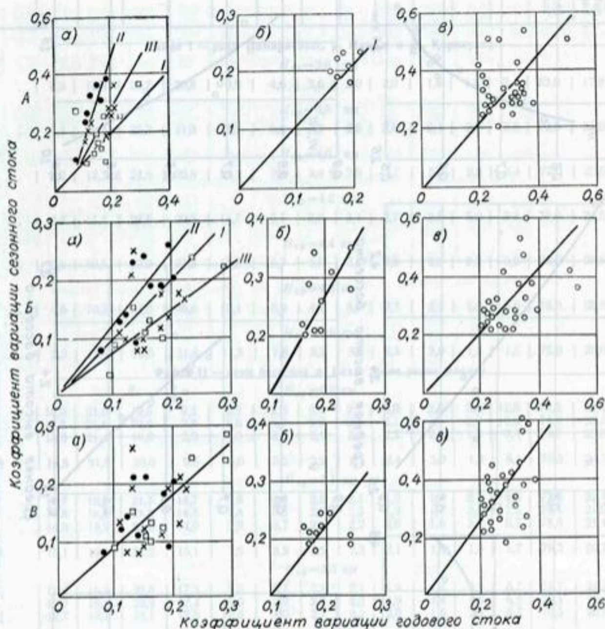
Рис. 51. Связь коэффициентов вариации годового и сезонного стока для рек бассейна Амударьи.
