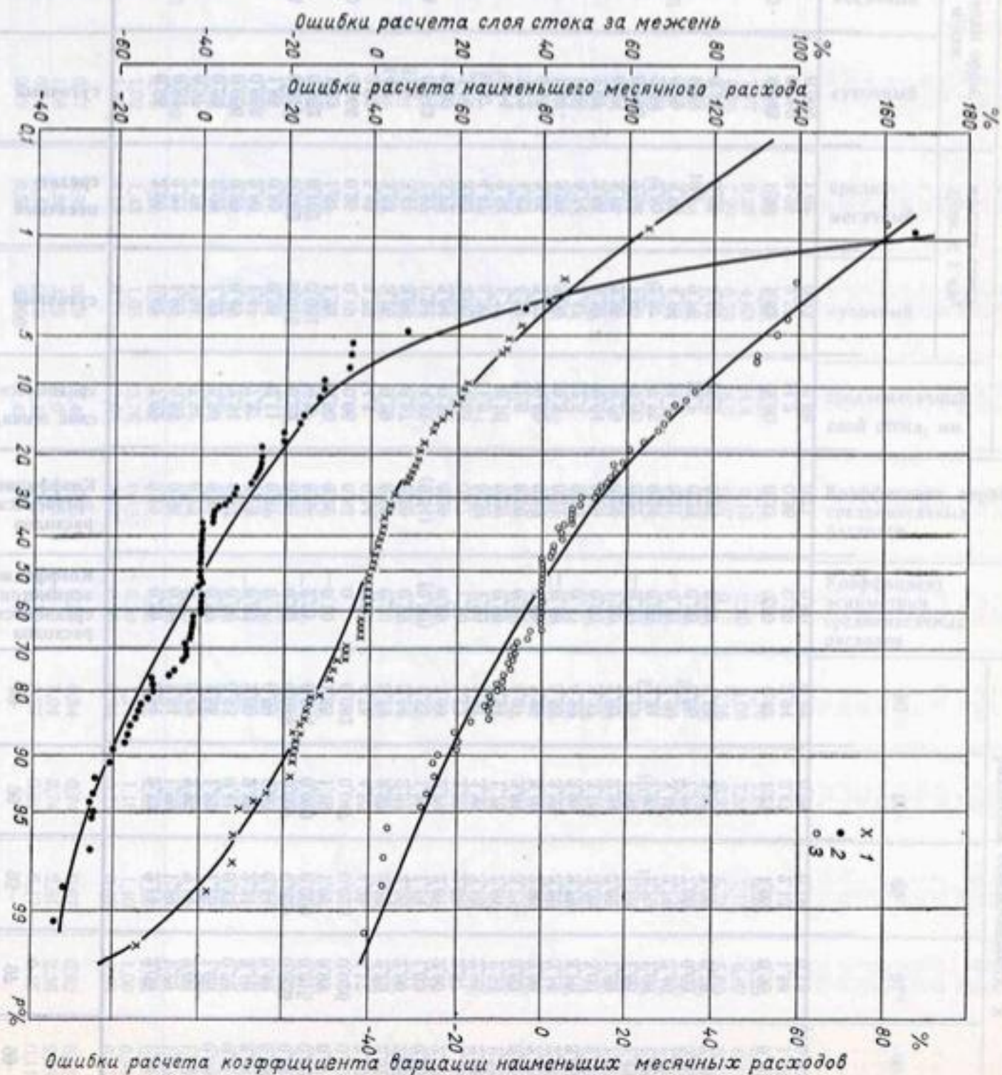
Рис. 76. Обеспеченность относительных ошибок расчета слоев стока за межень (1), минимального месячного стока (2) и коэффициентов вариации минимального месячного стока (3).
