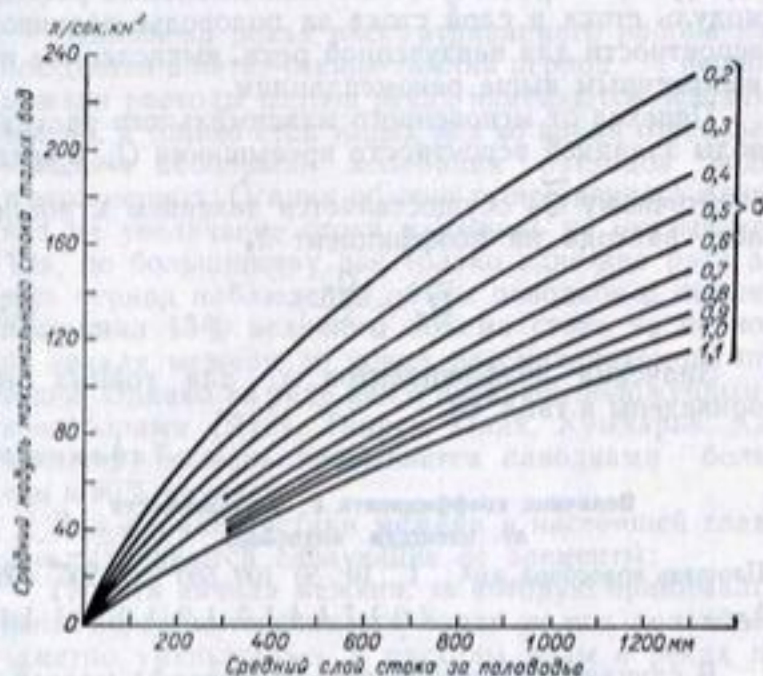
Рис. 68. Номограмма для определения среднего модуля максимального стока талых вод.
