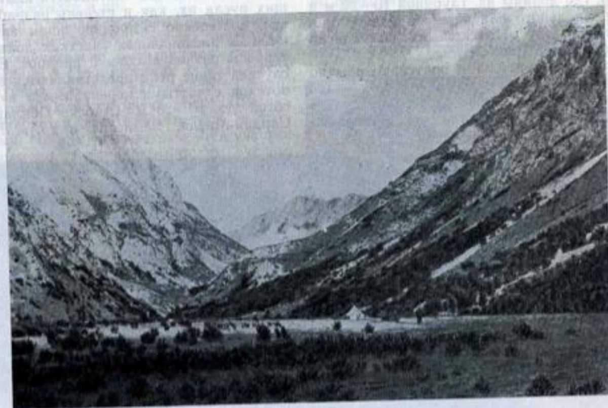
Рис. 23. Долина р. Кокеу (правый приток р. Кызылсу северная).
