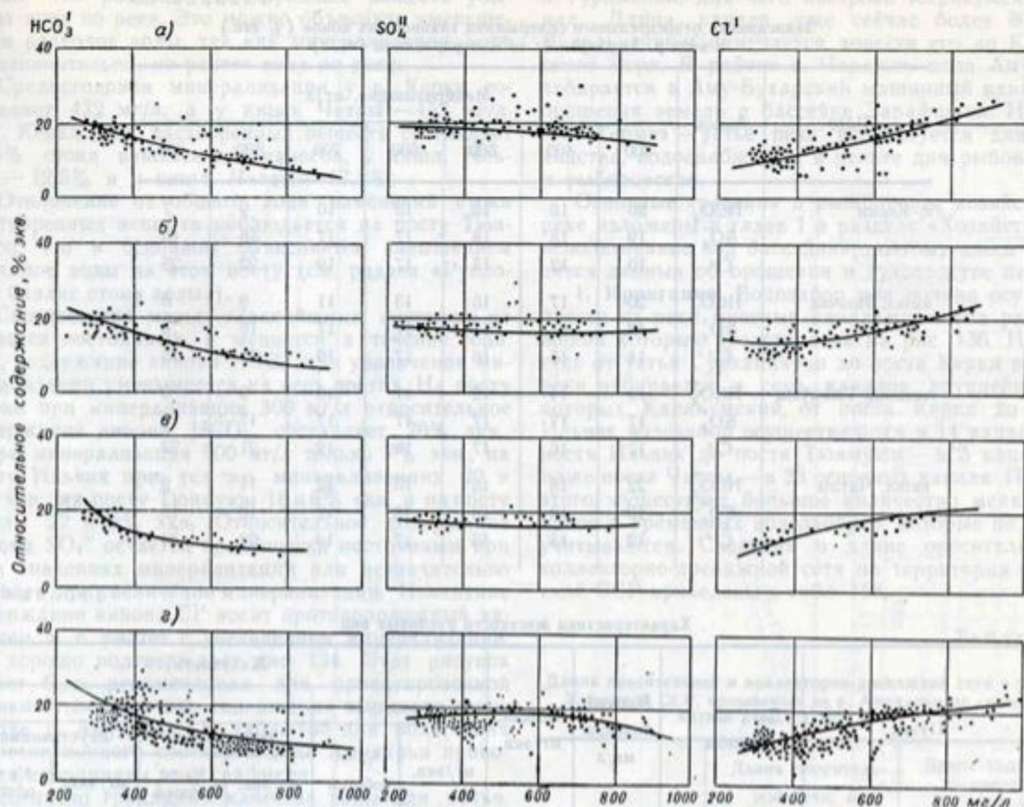
Рис. 134. Зависимость содержания главнейших ионов (в % экв.) в воде р. Амударьи от минерализации (мг/л). а — г. Керки, б — кишла. Ильячик, в — теснина Тюямурун, г — кишла. Чатам.
