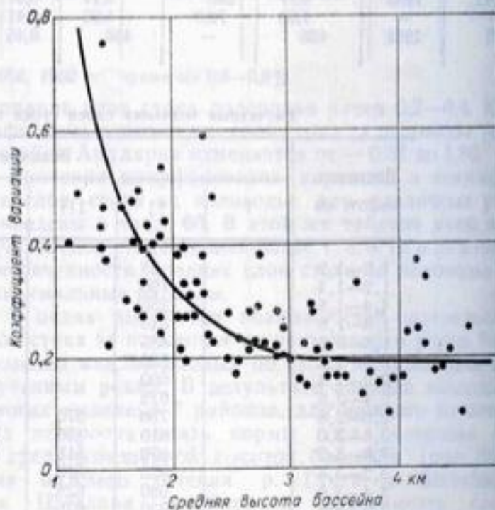
Рис. 61. Зависимость коэффициента вариации слоя половодья от средней высоты бассейнов.
