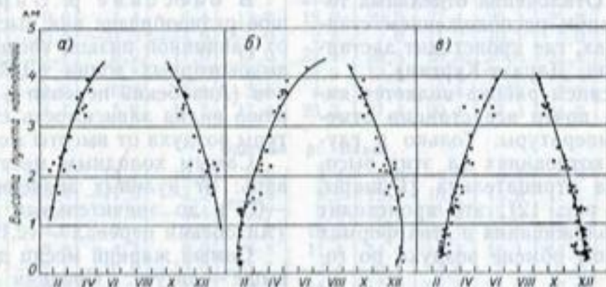
Рис. 13. Зависимость времени перехода температуры воздуха через +5^{\circ} (а), 0^{\circ} (б) и -5^{\circ} (в) от высоты места весной и осенью.
