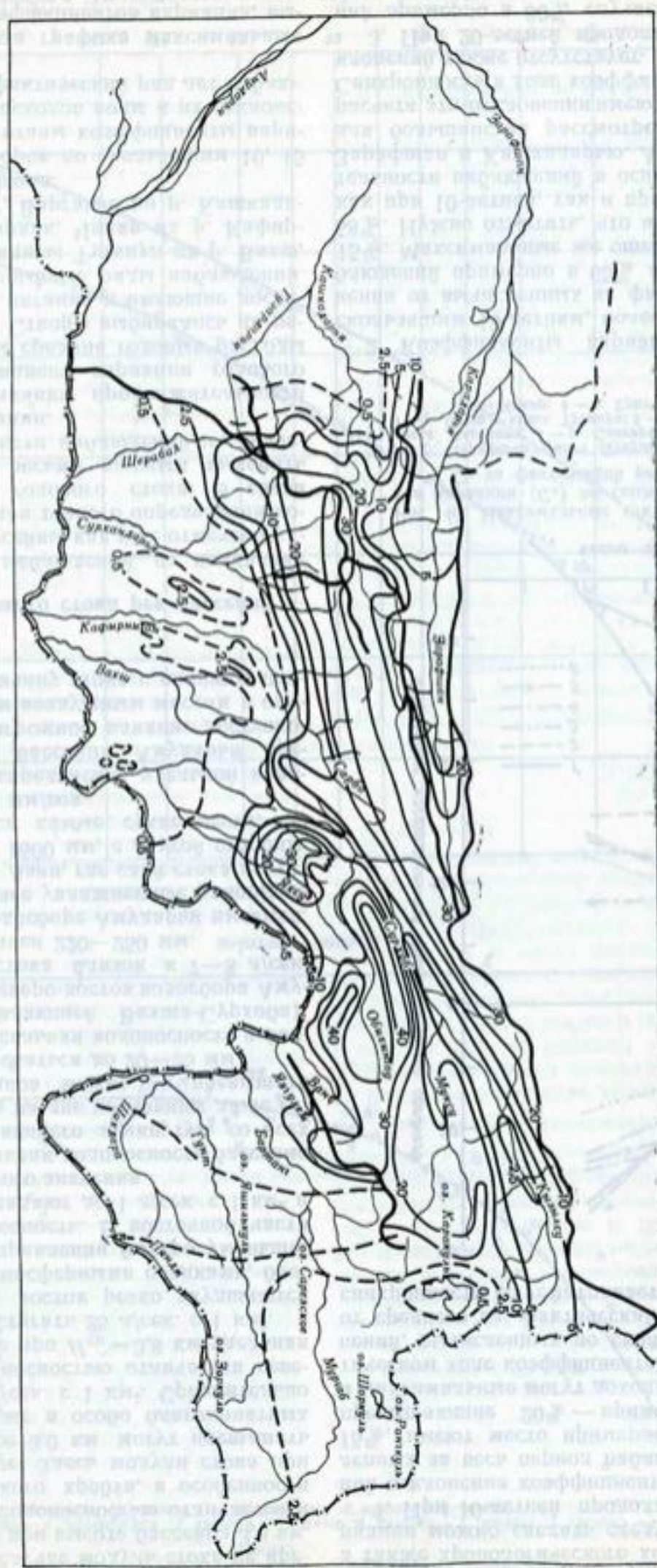
Рис. 45. Схематическая карта среднего многолетнего годового стока воды (д/сек. с 1 км 2 ) рек бассейна Амударьи.
