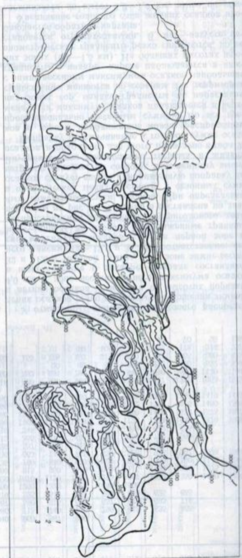
Рис. 17. Сverdловская карта средних многолетних сумм атмосферных осадков.
