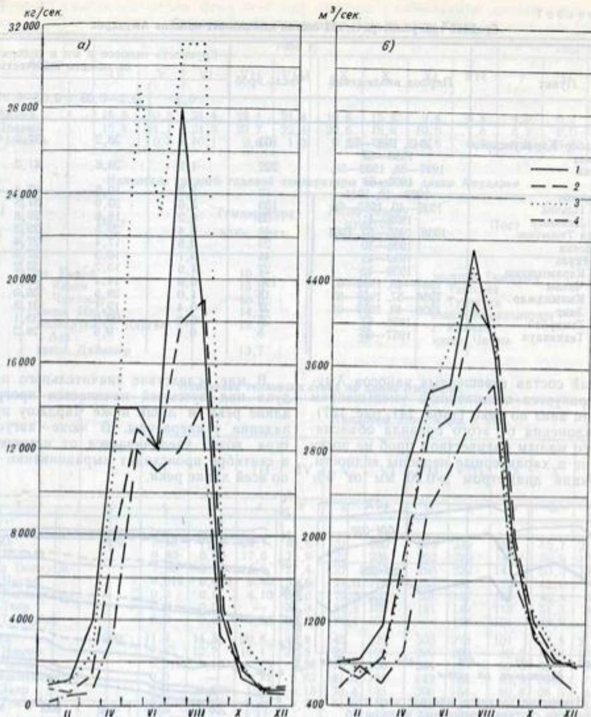
Рис 126. График колебания расходов взвешенных наносов (а) и расходов воды (б) на постах р. Амударьи за 1956 г.
