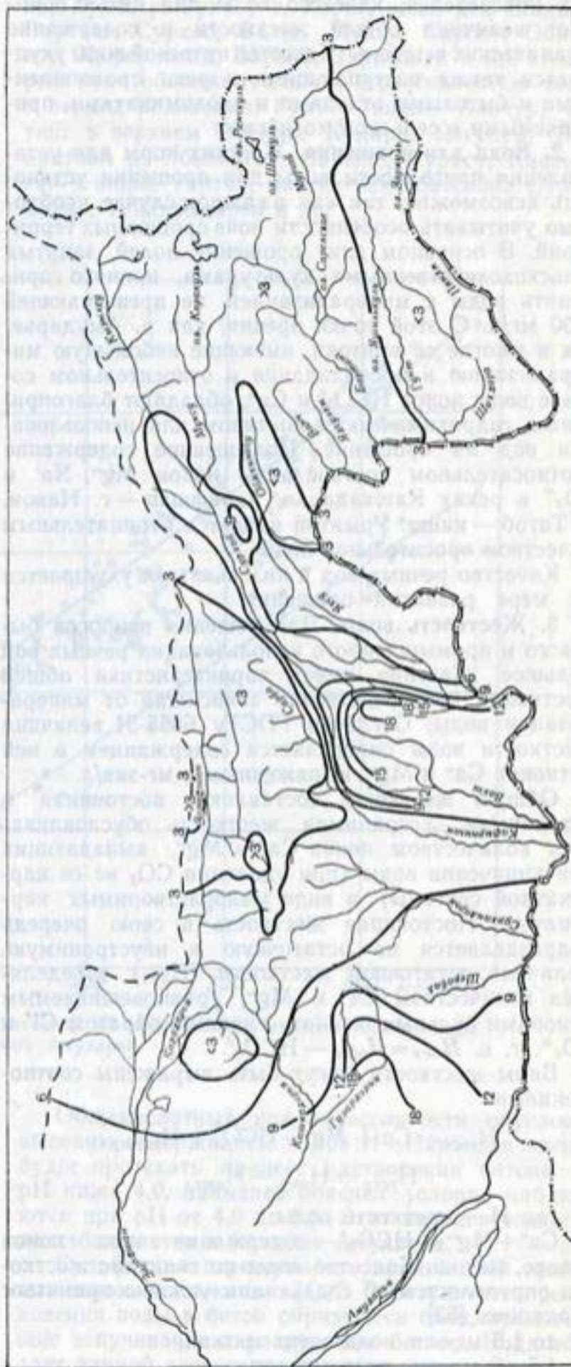
Рис. 116. Величина общей жесткости речной воды (мг-экв/л) в бассейне Амударьи в период межени.
