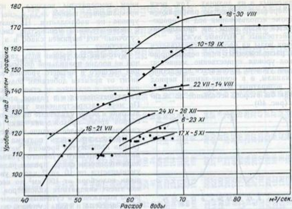
Рис. 39. Кривые расходов р. Бартаг у кишл. Барчадив за 1956 г.
