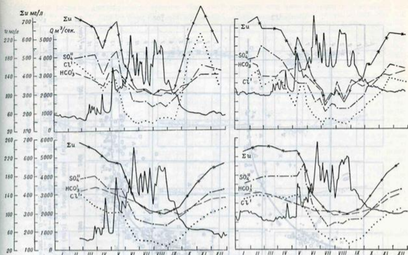
Рис. 132. Внутригодовое изменение расходов воды ( Q ), минерализации и содержания главных анионов в воде р. Амударьи в 1955 г.
