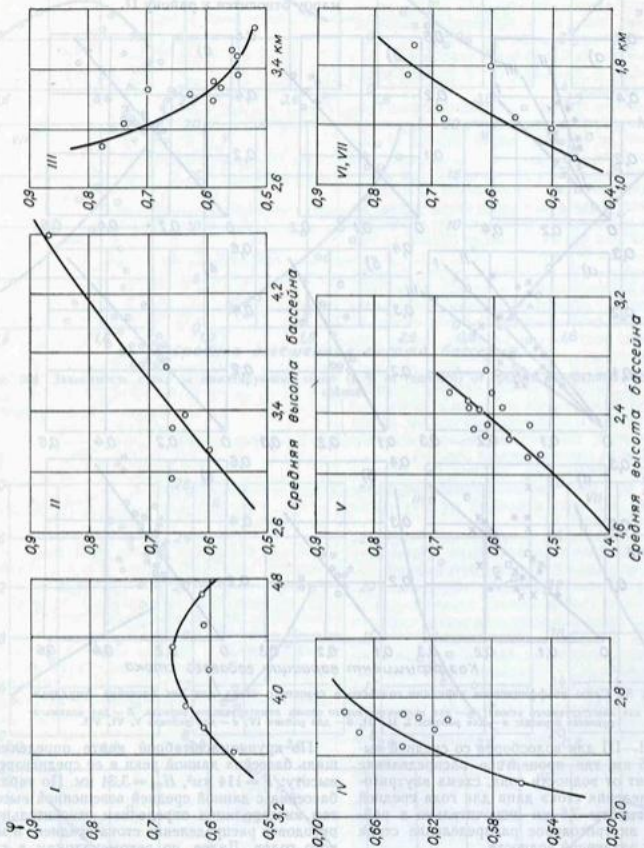
Рис. 52. Зависимость параметра зарегулированности стока \phi от высоты бассейнов.
