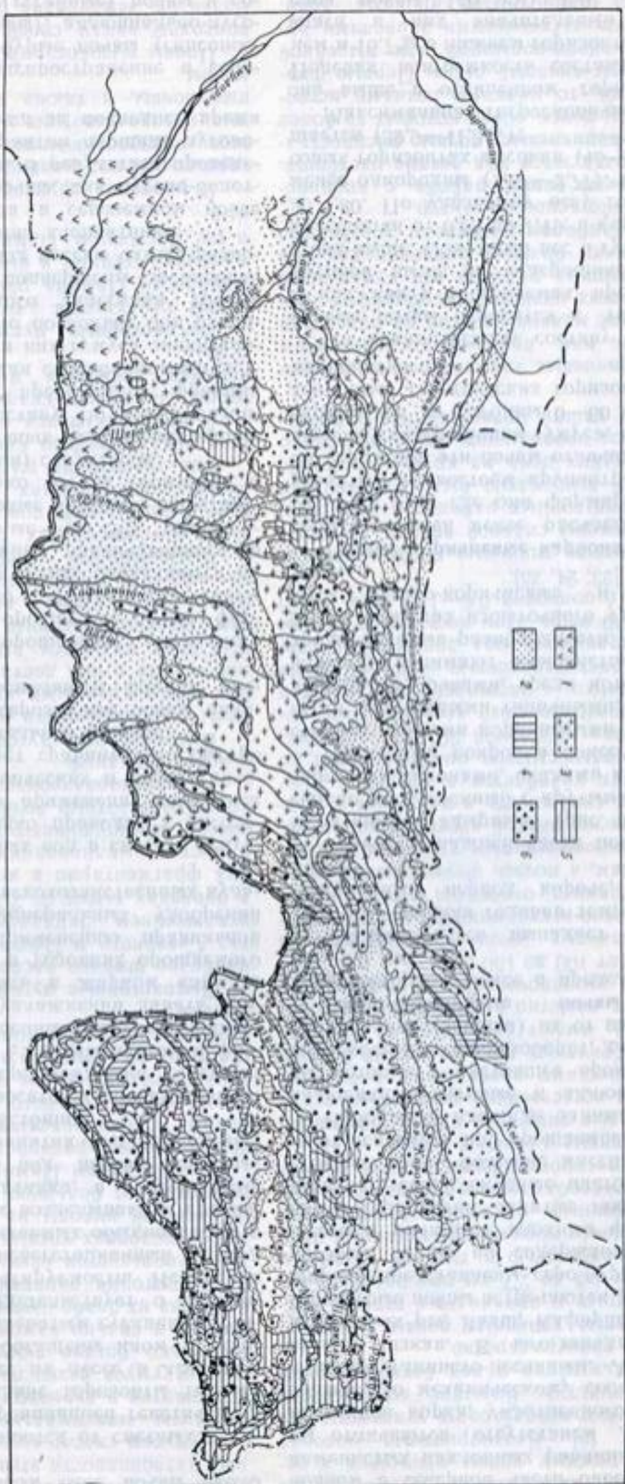
Рис. 9. Схематическая почвенная карта горной части бассейна Амударьи.
