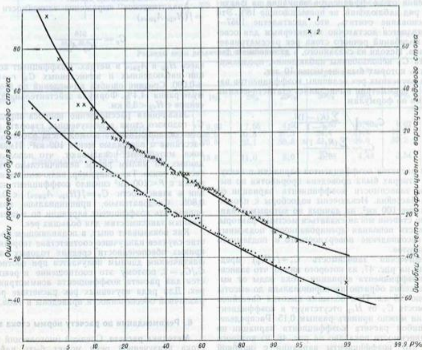
Рис. 48. Обеспеченность относительных ошибок расчета нормы стока (1) и коэффициентов вариации расходов воды (2) для рек бассейна Амударьи.
