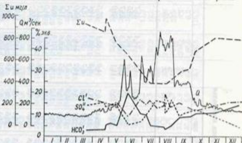
Рис. 111. Внутригодовое изменение расходов воды, минерализации и содержания главных ионов в воде р. Вахш у г. Гарм за 1951 г.
