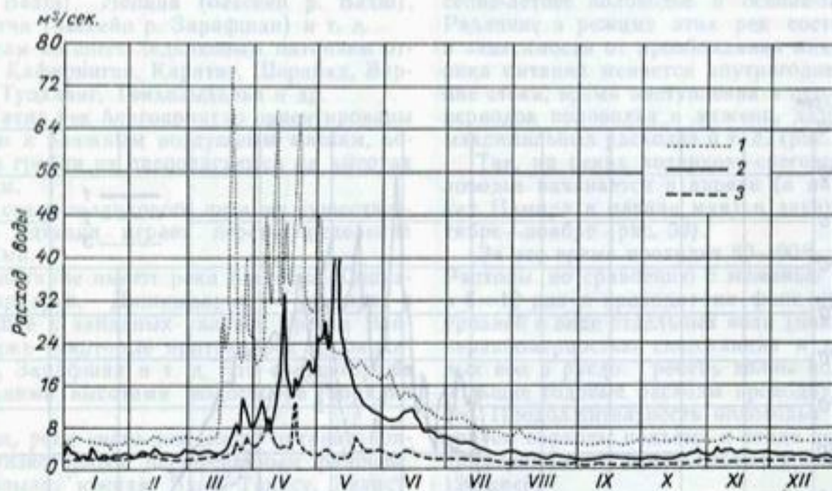
Рис. 32. Гидрограф стока р. Гузардары у кишла. Яртепа за характерные по водности годы.
