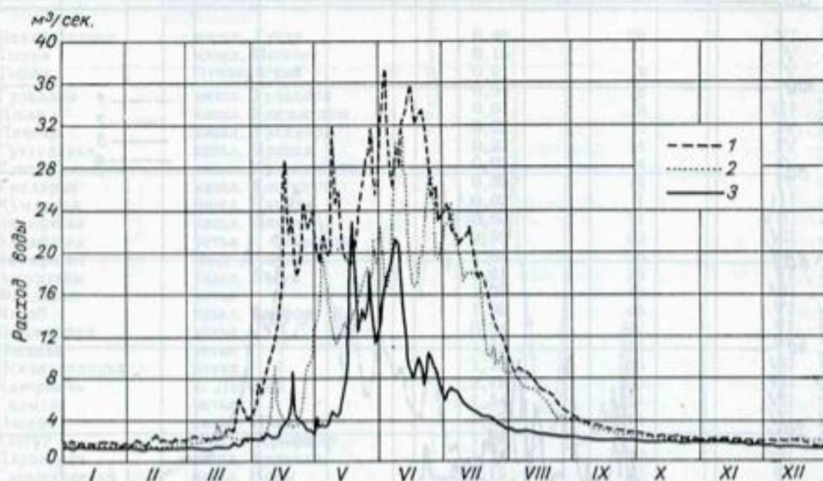
Рис. 31. Гидрограф стока р. Яккабагдары у кишла. Татар за характерные по водности годы.
