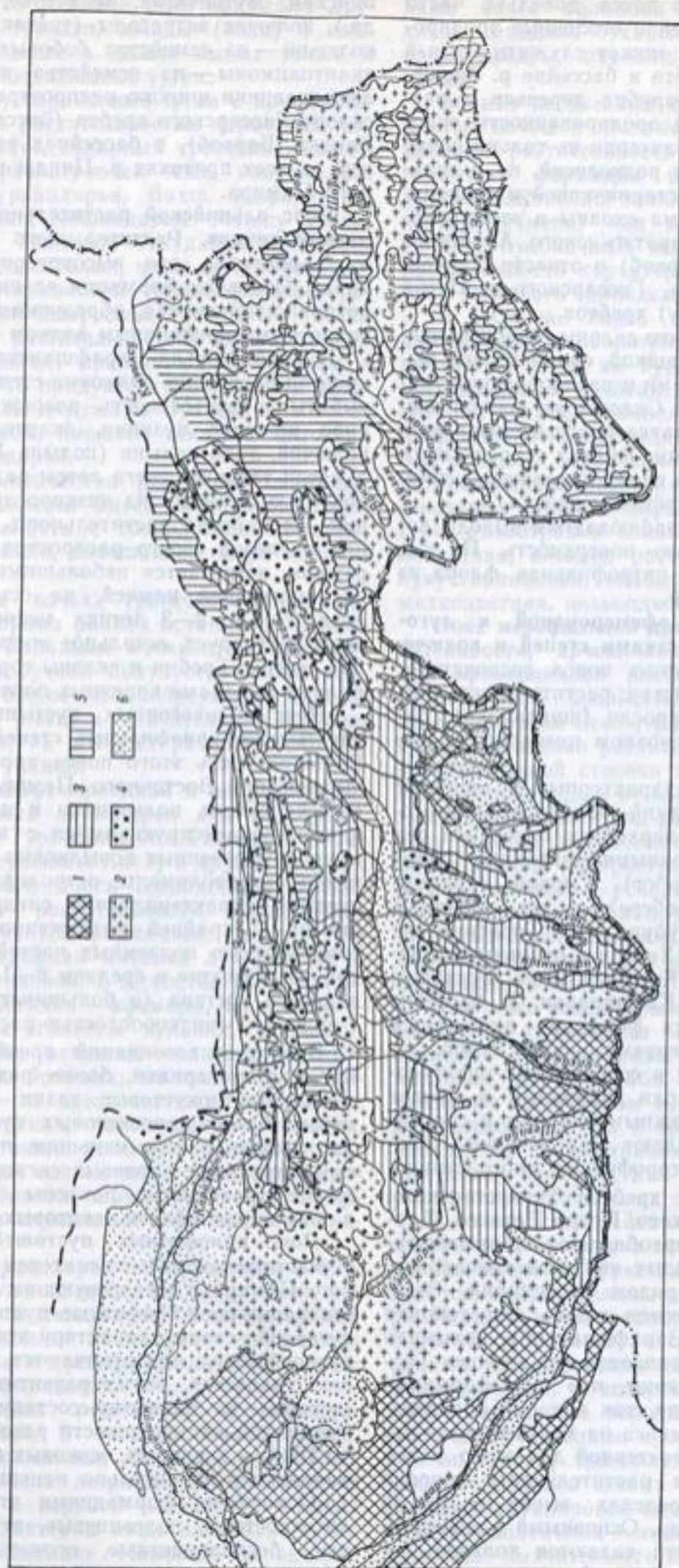
Рис. 10. Схематическая карта типов растительности бассейна Амурарын.
