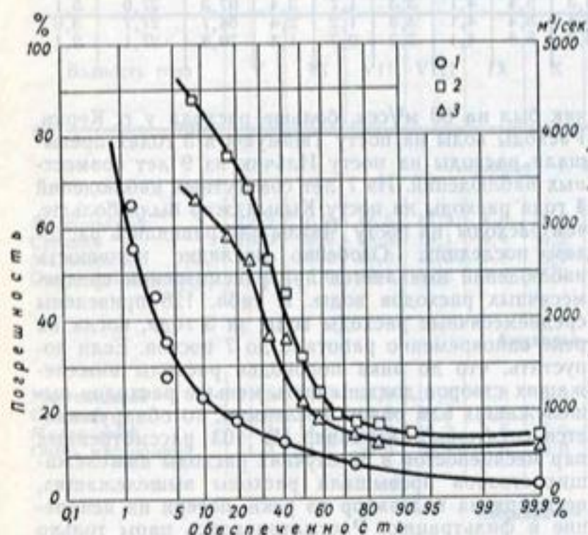
Рис. 123. График обеспеченности относительных ошибок вычисления среднемесячных расходов на постах р. Амударья (1) и кривые обеспеченности среднемесячных расходов по постам Керки (2) и Чатлы (3).
