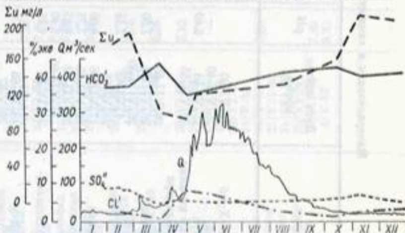
Рис. 112. Внутригодовое изменение расходов воды, минерализации и содержания главных ионов в воде р. Кафирниган у кишл. Чинар за 1950 г.
