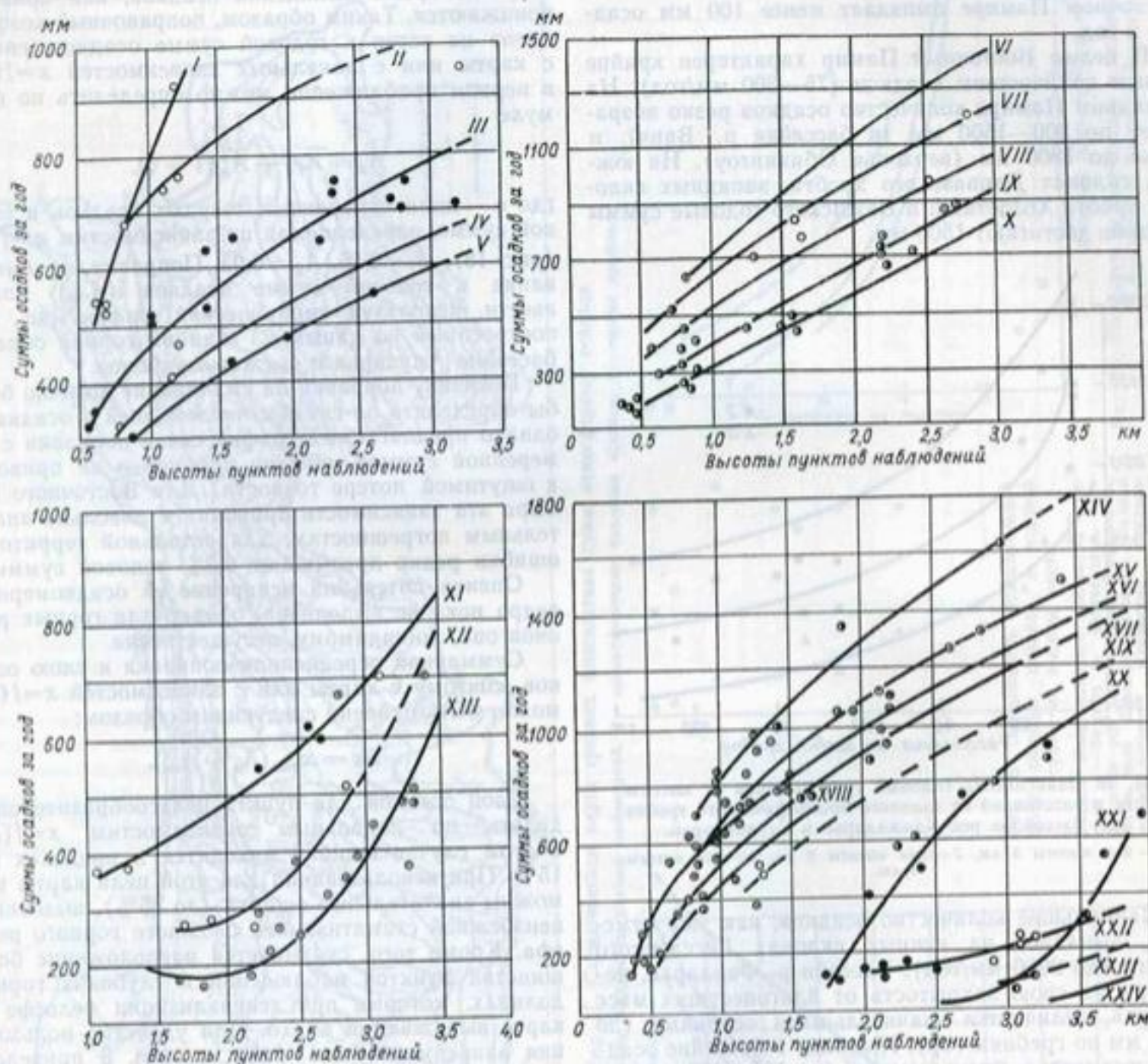
Рис. 15. Зависимость годовых сумм осадков от высоты места.
