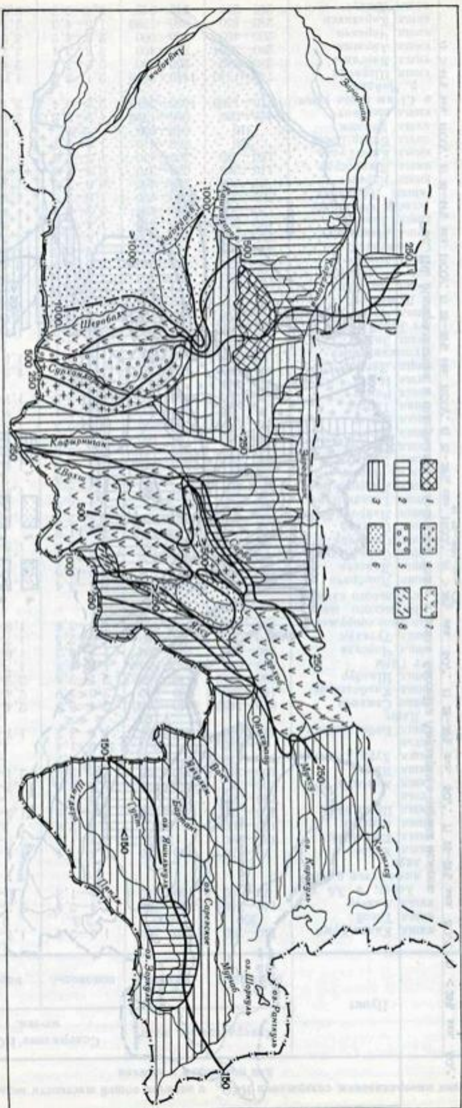
Рис. 109. Минерализация воды и содержание главных ионов в реках бассейна Амударьи в период половодья. 1) >44\% экв. \text{HCO}_3^- ; 2) 36-44\% экв. \text{HCO}_3^- ; 3) 28-36\% экв. \text{HCO}_3^- ; 4) 25-28\% экв. \text{HCO}_3^- ; 5) <25\% экв. \text{HCO}_3^- ; 6) 25-28\% экв. \text{SO}_4^{2-} ; 7) <25\% экв. \text{SO}_4^{2-} ; 8) 28-36\% экв. \text{SO}_4^{2-} .
