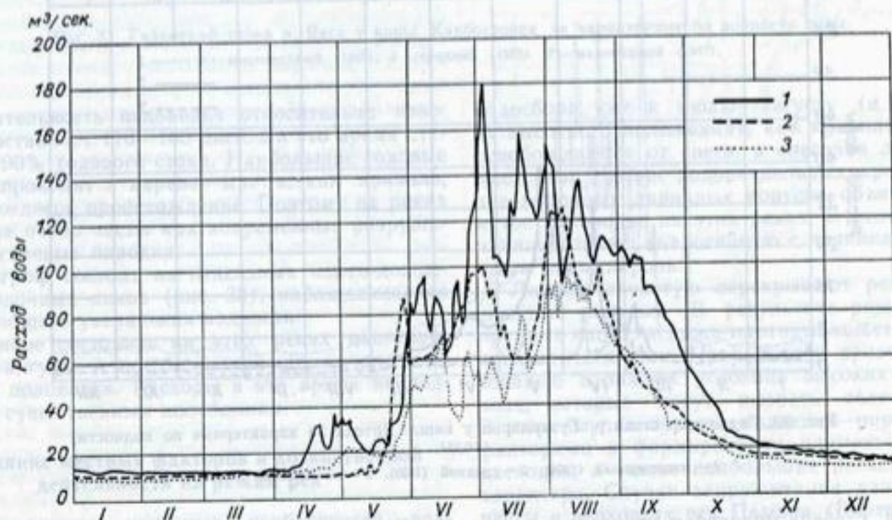
Рис. 30. Гидрограф стока р. Язгулем у кишла. Мотравни за характерные по водности годы. 1 — многоводный (1950), 2 — средний (1951), 3 — маловодный (1955).
