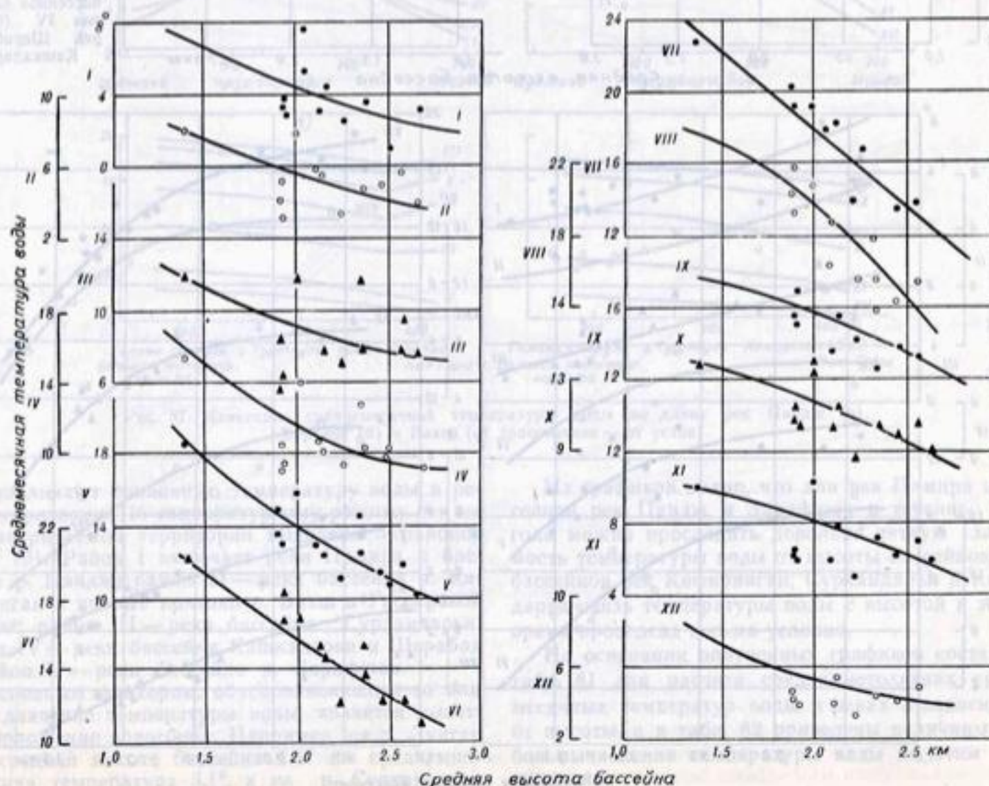
Рис. 84. Зависимость средней многолетней среднемесячной температуры воды рек от средней высоты бассейнов для рек района III (бассейн р. Сурхандарья).
