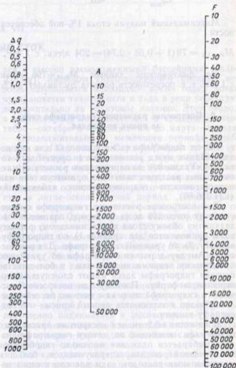
Рис. 69. Номограмма для определения дождевой надбавки \Delta q к наибольшим расходам талых вод.
