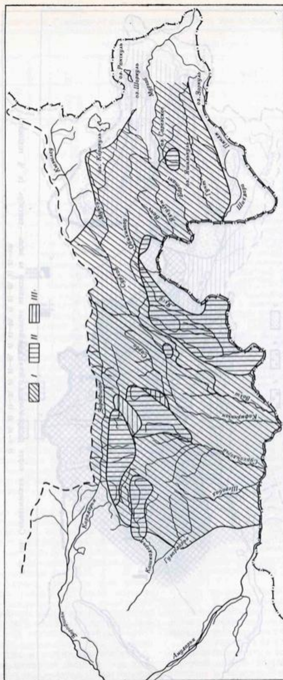
Рис. 102. Схематическая карта распределения стока взвешенных наносов за октябрь — февраль (в % годового). П 0-2, II) 3-5, III) 6-10.
