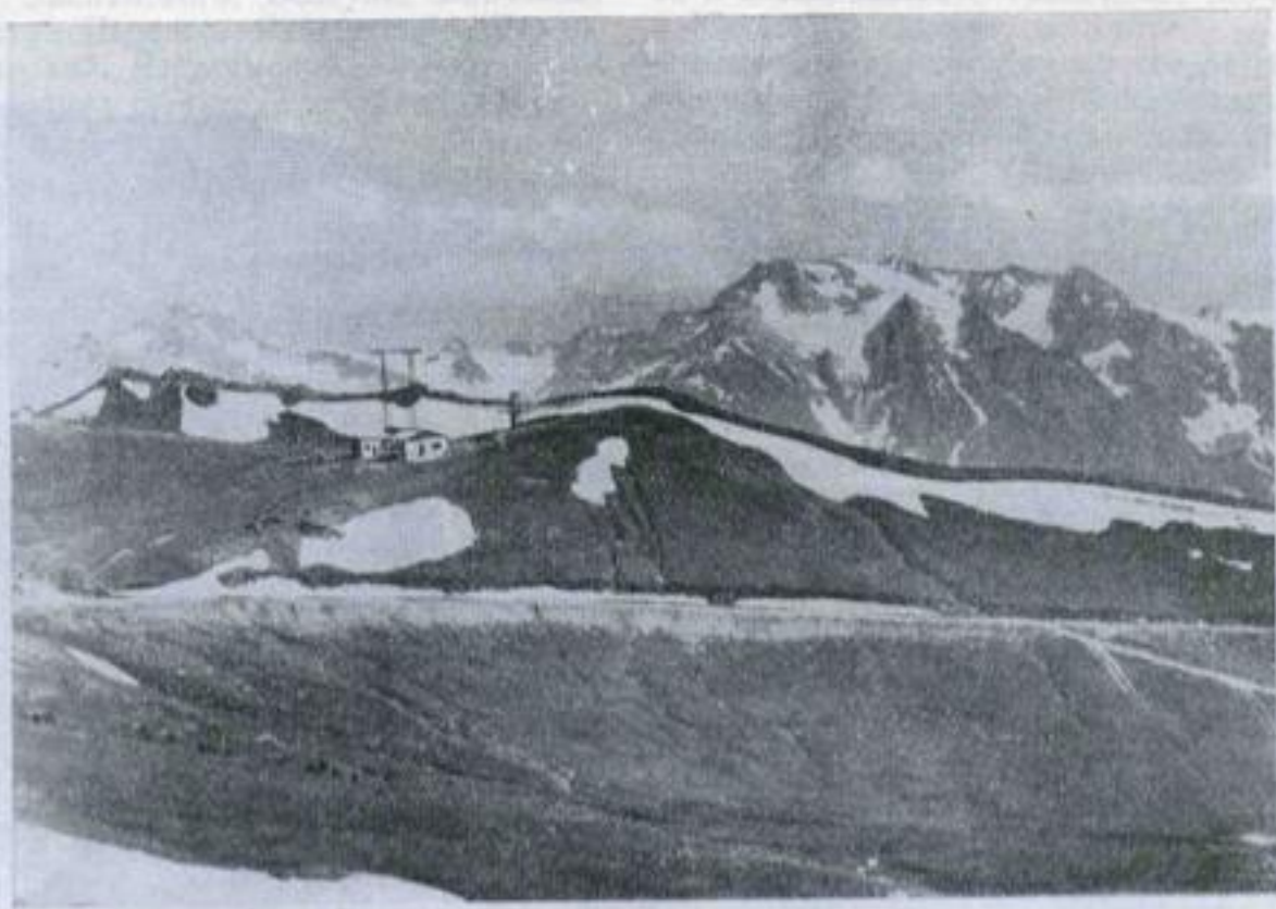
Рис. 3. Вид Гиссарского хребта в районе Анзобского перевала.
