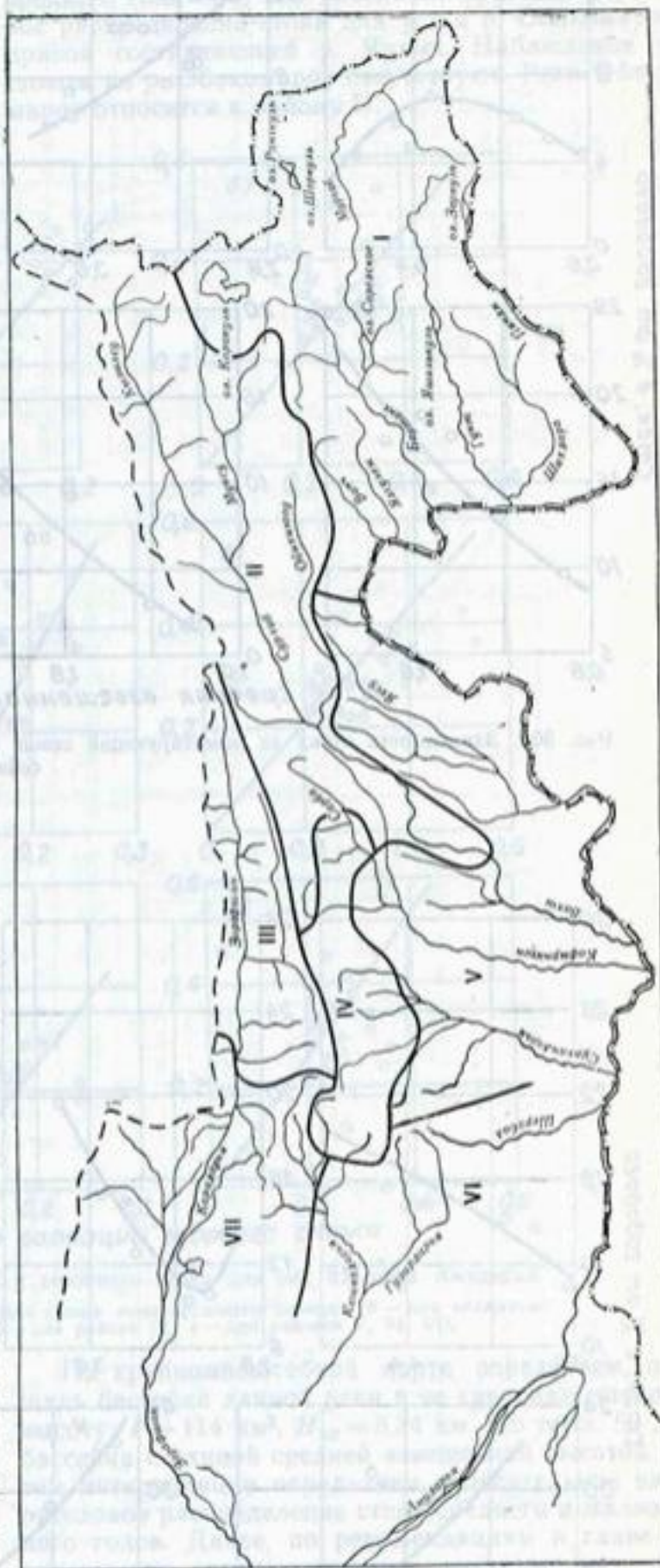
Рис. 49. Схема районирования бассейна Амударьи по виду зависимости внутригодового распределения стока от высоты бассейна.
