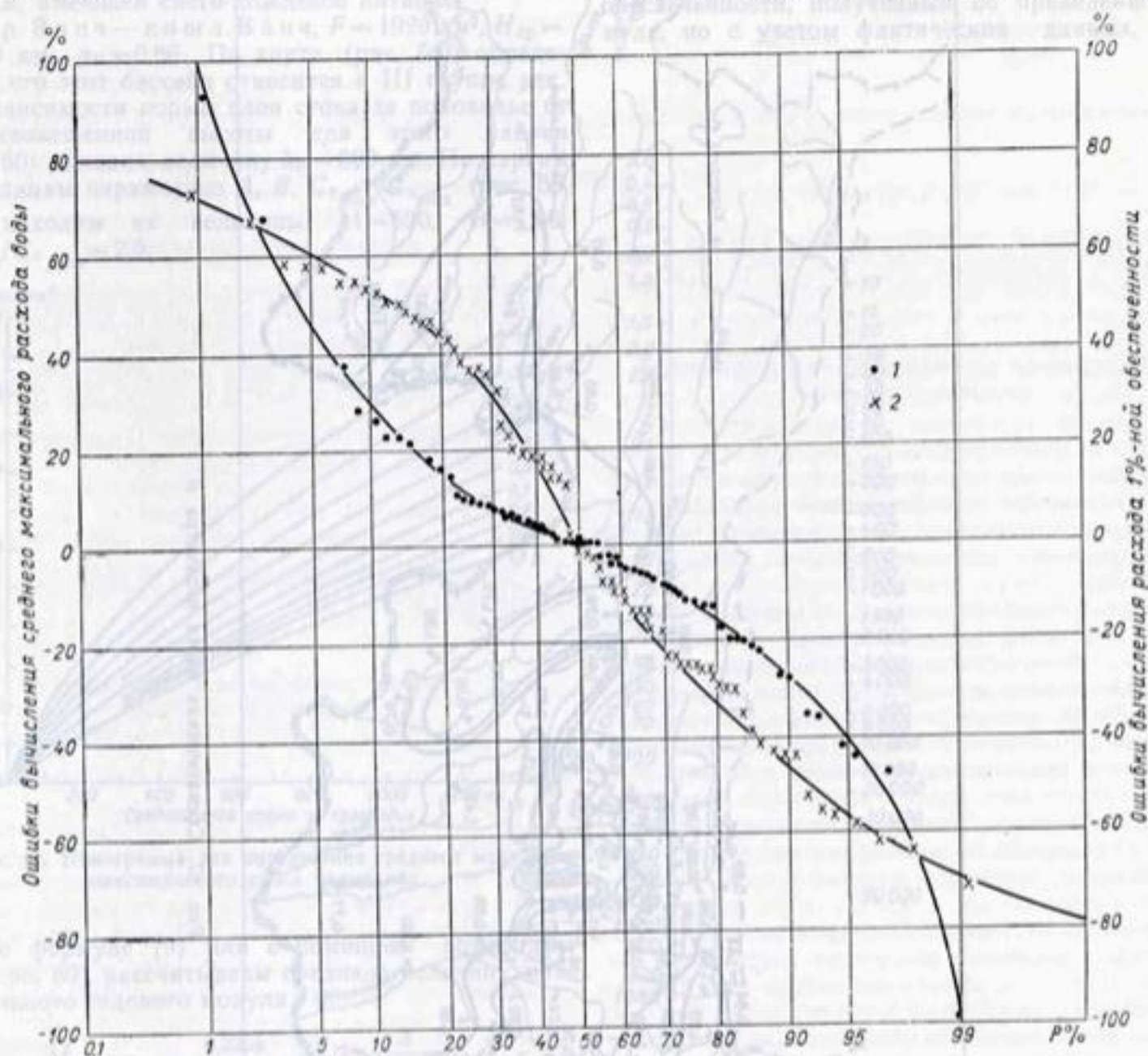
Рис. 66. Обеспеченность относительных ошибок расчета нормы максимального модуля стока (1) и максимальных расходов 1%-ной обеспеченности (2).
