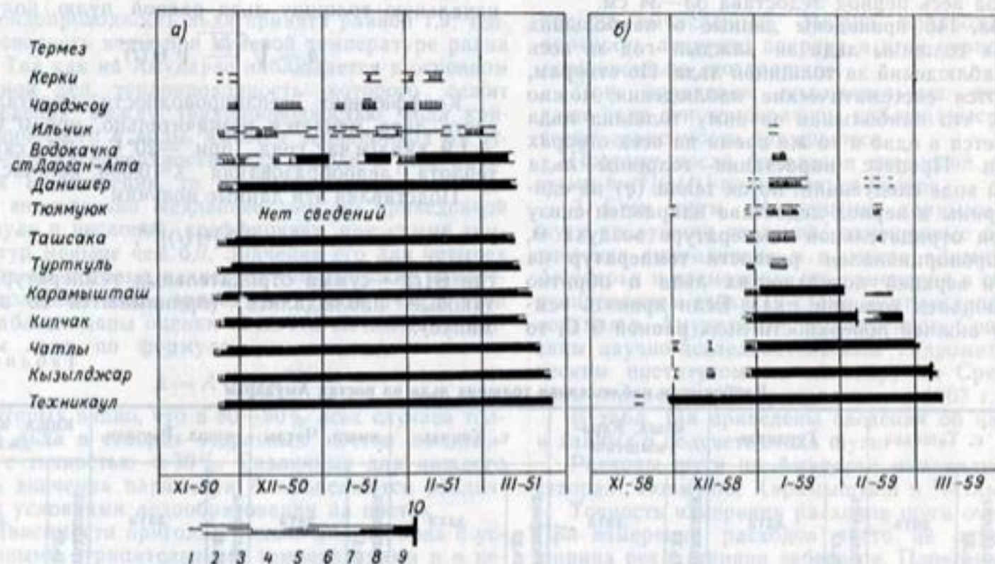
Рис. 130. Характер ледовых явлений на постах р. Амударьи холодной зимой 1950-51 г. (а) и теплой зимой 1958-59 г. (б).
