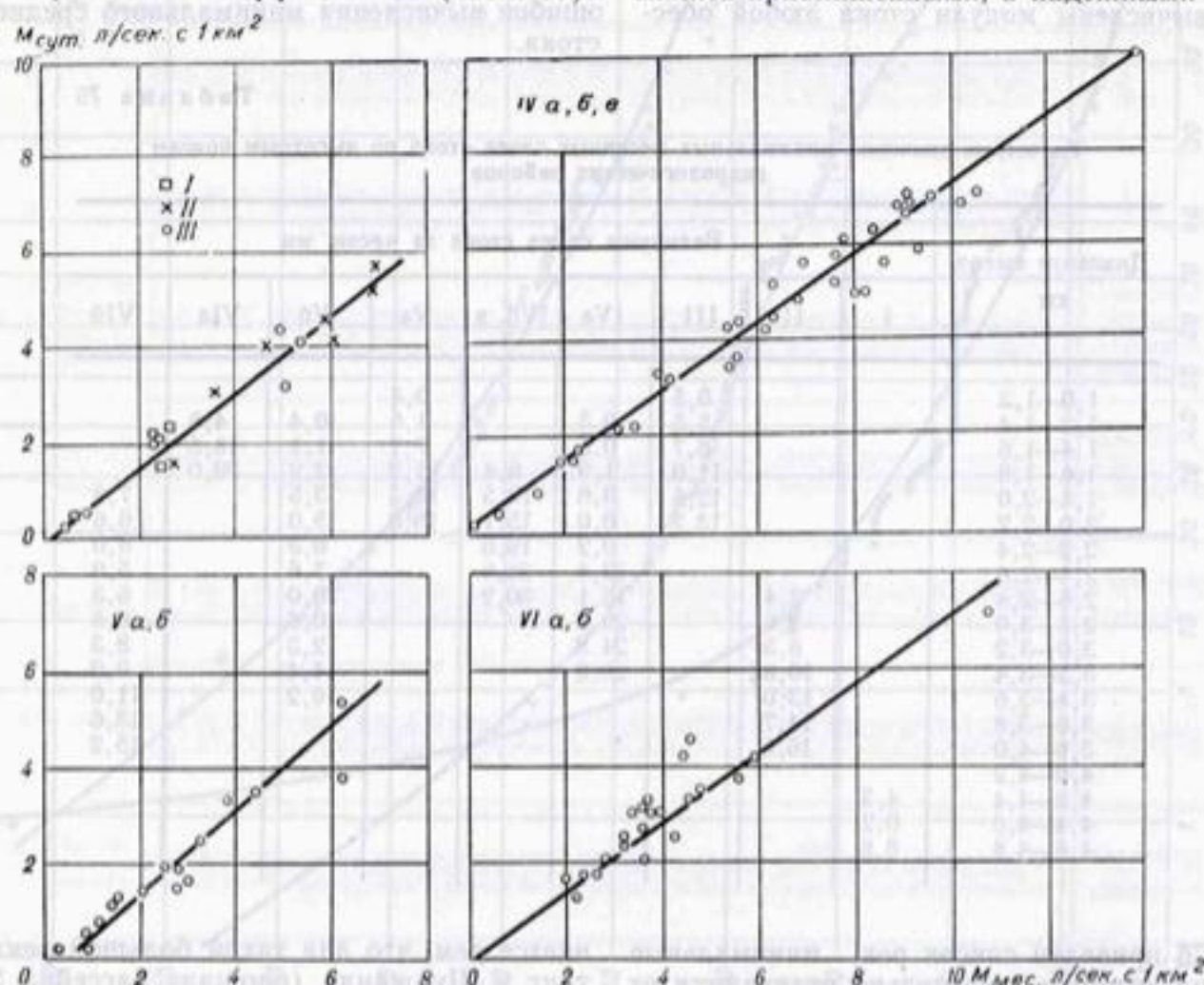
Рис. 77. Зависимость модуля суточного минимального стока ( M_{сут} ) от модуля месячного минимального стока ( M_{мес} ) для различных районов бассейна Амударьи.
