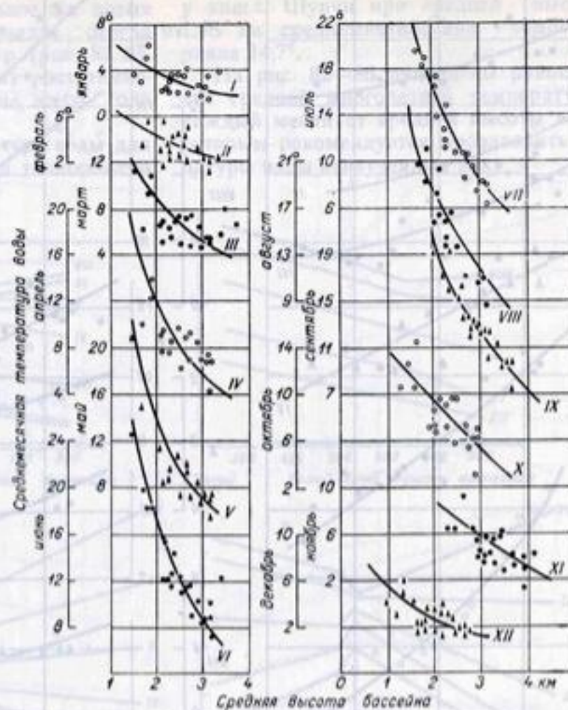
Рис. 83. Зависимость средней многолетней среднемесячной температуры воды рек от средней высоты бассейнов для рек района II (бассейн р. Кафиринган и нижняя часть бассейна р. Вахш).
