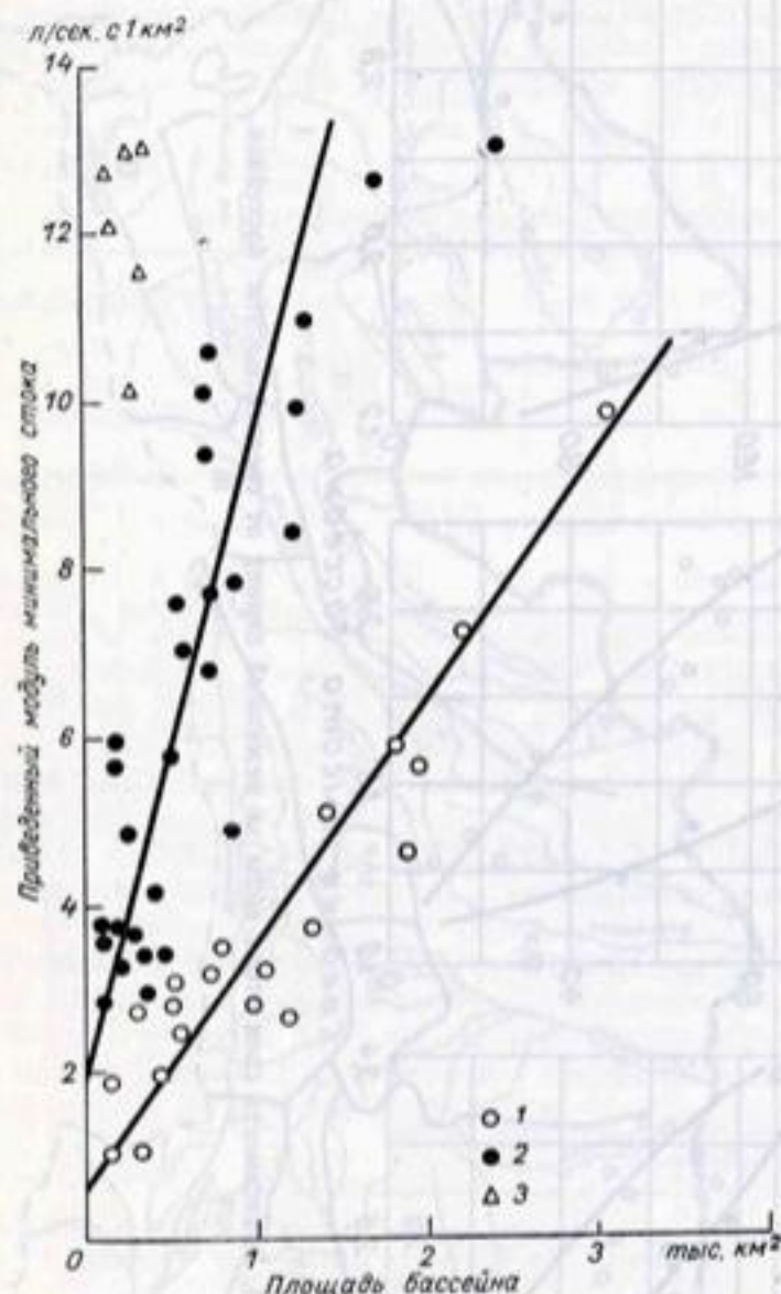
Рис. 72. Зависимость приведенного модуля месячного стока от площади бассейнов рек для области низкого (1), повышенного (2) и высокого (3) меженного стока.
