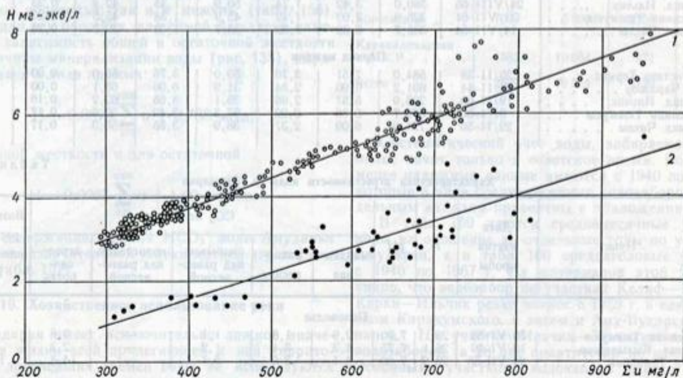
Рис. 135. Характер связи величин общей (1) и остаточной (2) жесткости с минерализацией воды р. Амударьи.
