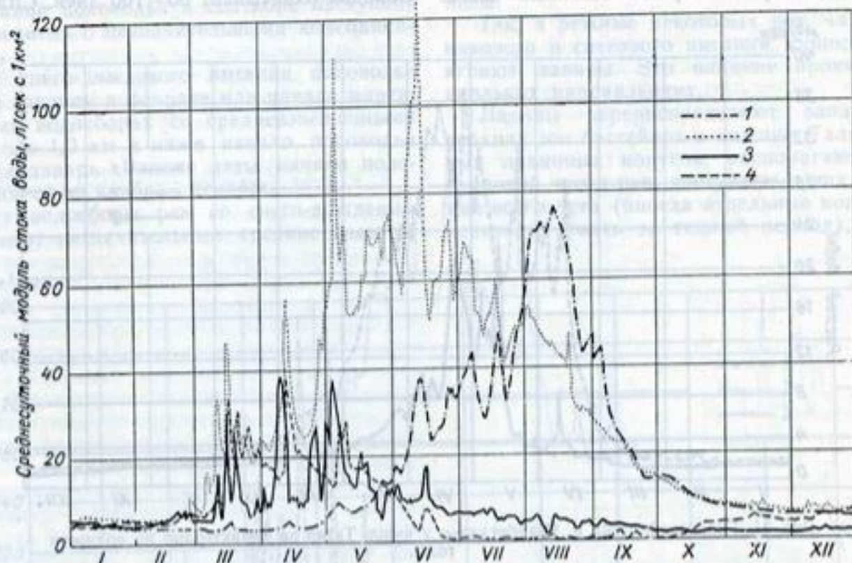
Рис. 29. График колебания ежедневных модулей стока воды за 1955 г. на реках различного типа питания.
