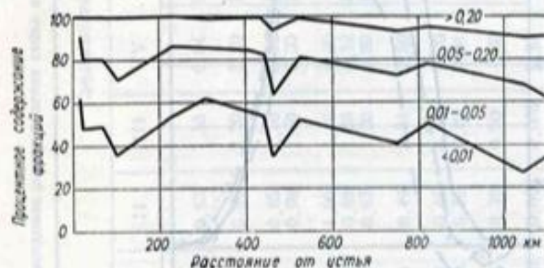
Рис. 127. Изменение среднего многолетнего гранулометрического состава взвешенных наносов по длине р. Амударьи.
