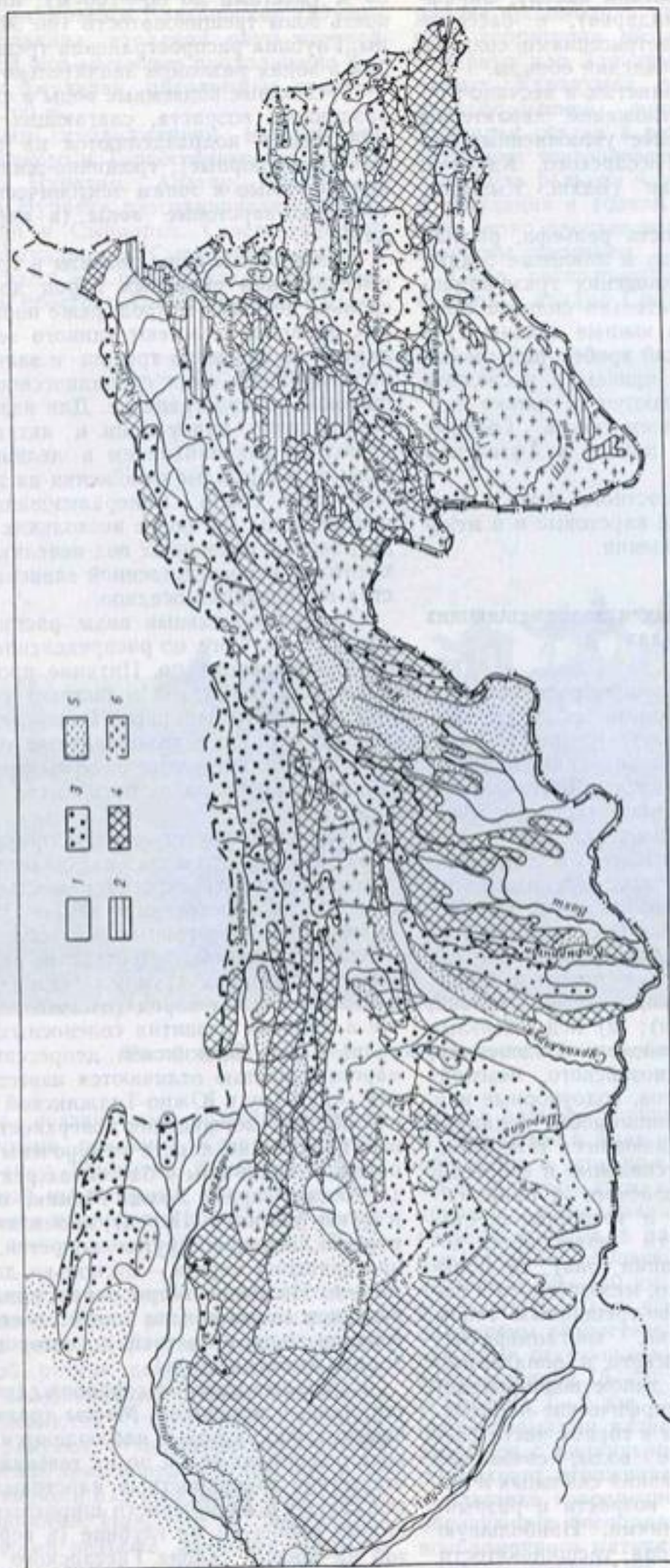
Рис. 8. Геолого-литологическая схема горной части бассейна Амударьи.
