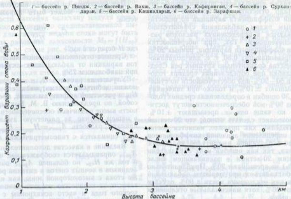
Рис. 47. Зависимость коэффициентов вариации годового стока воды от высоты бассейнов.
