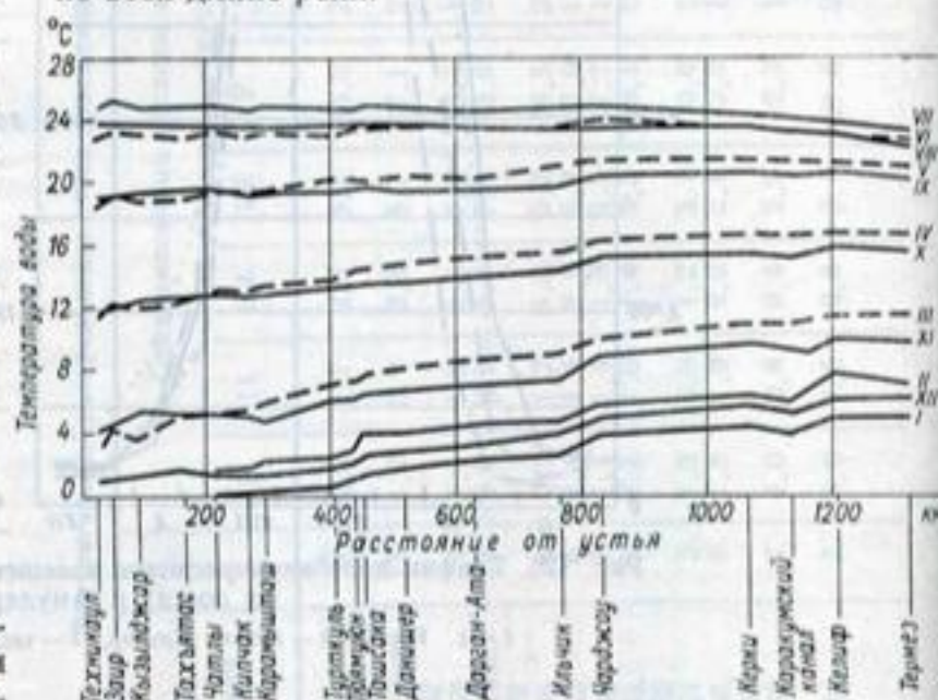
Рис. 128. Изменение средних многолетних среднемесячных температур воды по длине р. Амударьи.
