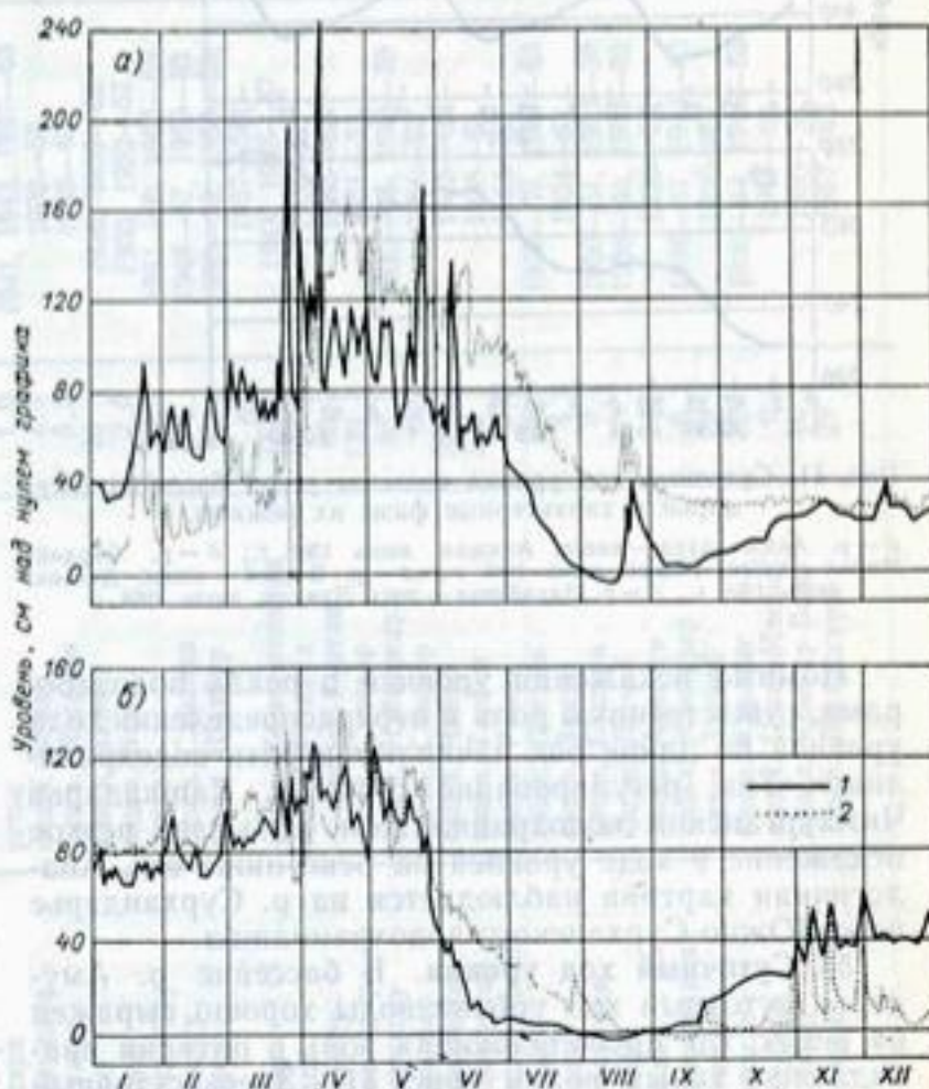
Рис. 40. Годовой ход уровня воды в р. Яхсу на постах выше (1 — кишл. Карбозтонак) и ниже (2 — пгт им. Весе) за многоводный 1949 (а) и маловодный 1947 (б) годы.
