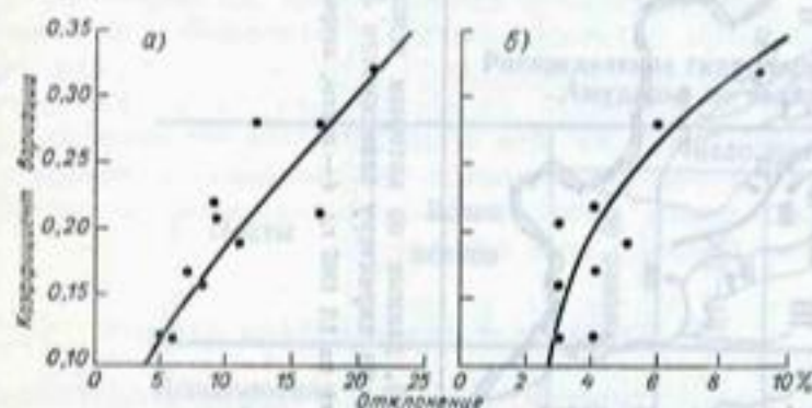
Рис. 43. Зависимость наибольших отклонений Q_n/Q_{cp} от коэффициента вариации.
