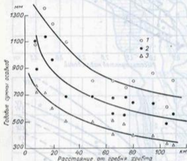
Рис. 16. Зависимость годовых сумм осадков от высоты места и расстояния от главного орографического гребня для бассейнов рек Кашкадарьи и Сурхандарьи.
