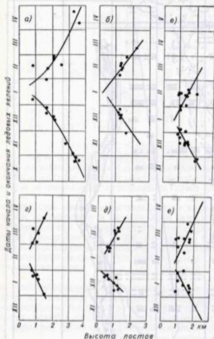
Рис. 91. Зависимость дат начала и окончания ледовых явлений от высоты поста для рек бассейна р. Пяндж (а), бассейна р. Вахш (б), бассейна р. Кафирниган (в), бассейнов рек Сурхандарья и Шерабад (г), бассейна р. Кашкадарья (д), бассейна р. Зарафшан (е).
