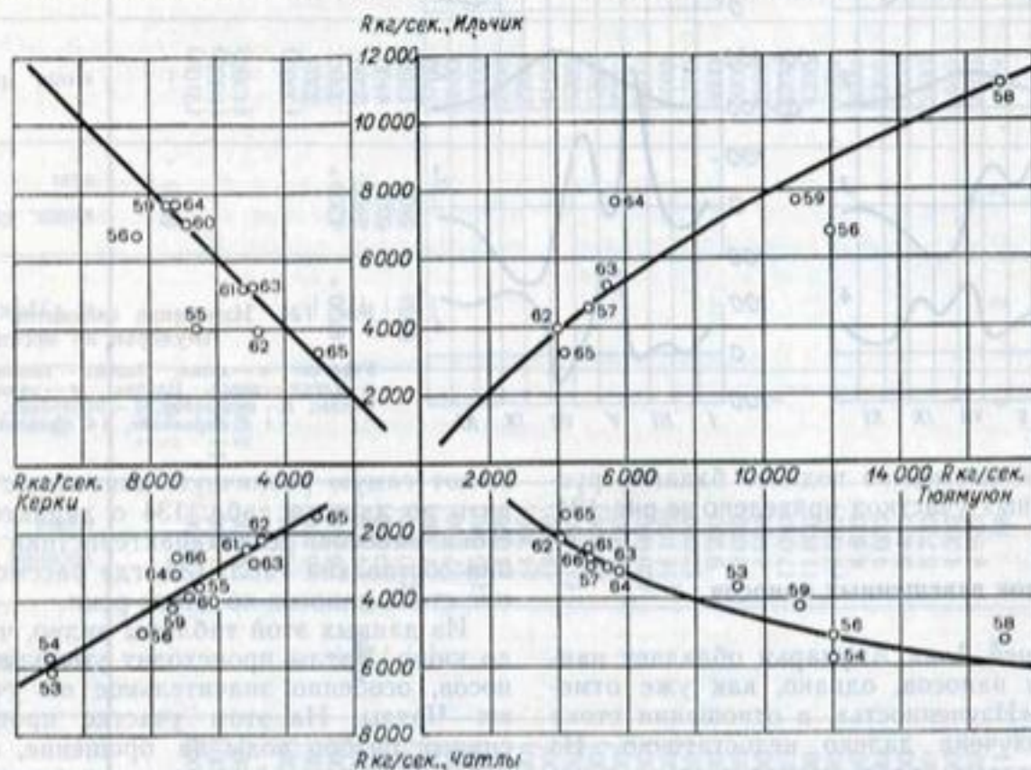
Рис. 125. Графики связи среднегодовых расходов взвешенных наносов по постам р. Амударья.
