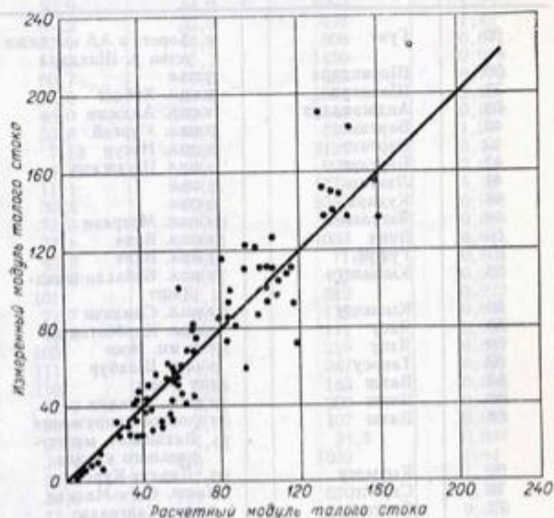
Рис. 63. Сравнение вычисленных и наблюдаемых модулей максимальных талых расходов.
