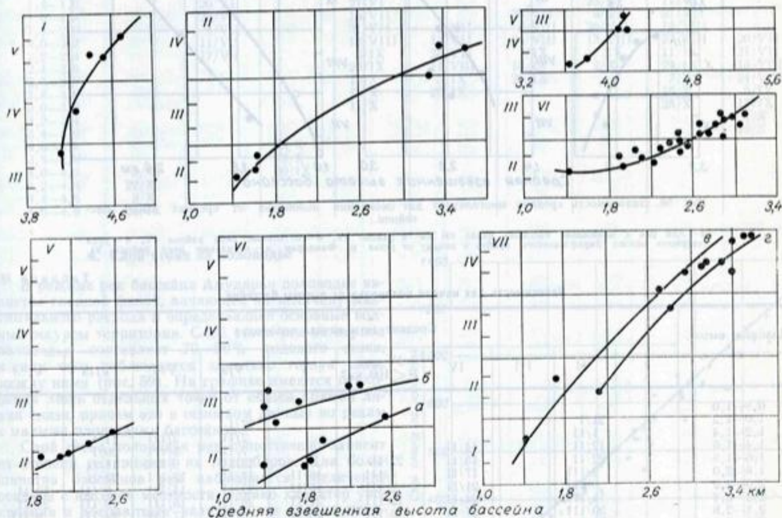
Рис. 57. Зависимость средних многолетних дат начала половодья от средних высот бассейнов для рек бассейна Амударьи.
