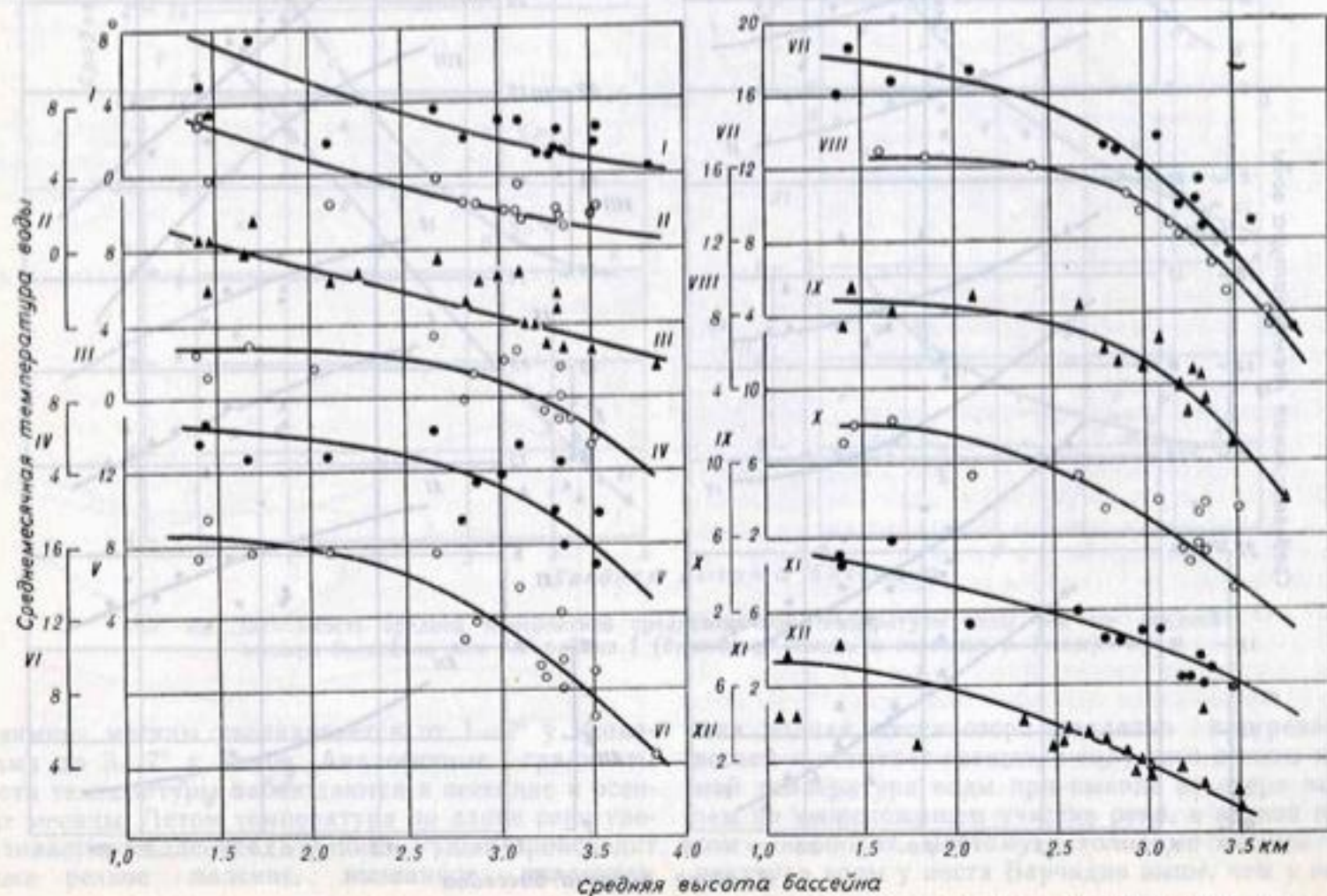
Рис. 86. Зависимость средней многолетней среднемесячной температуры воды рек от средней высоты бассейнов для рек района V (бассейн р. Зарафшан).
