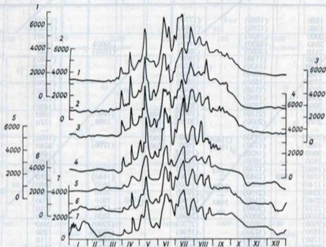
Рис. 121. График колебания расходов воды ( \text{м}^3/\text{сек.} ) на постах р. Амударьи в 1959 г.
