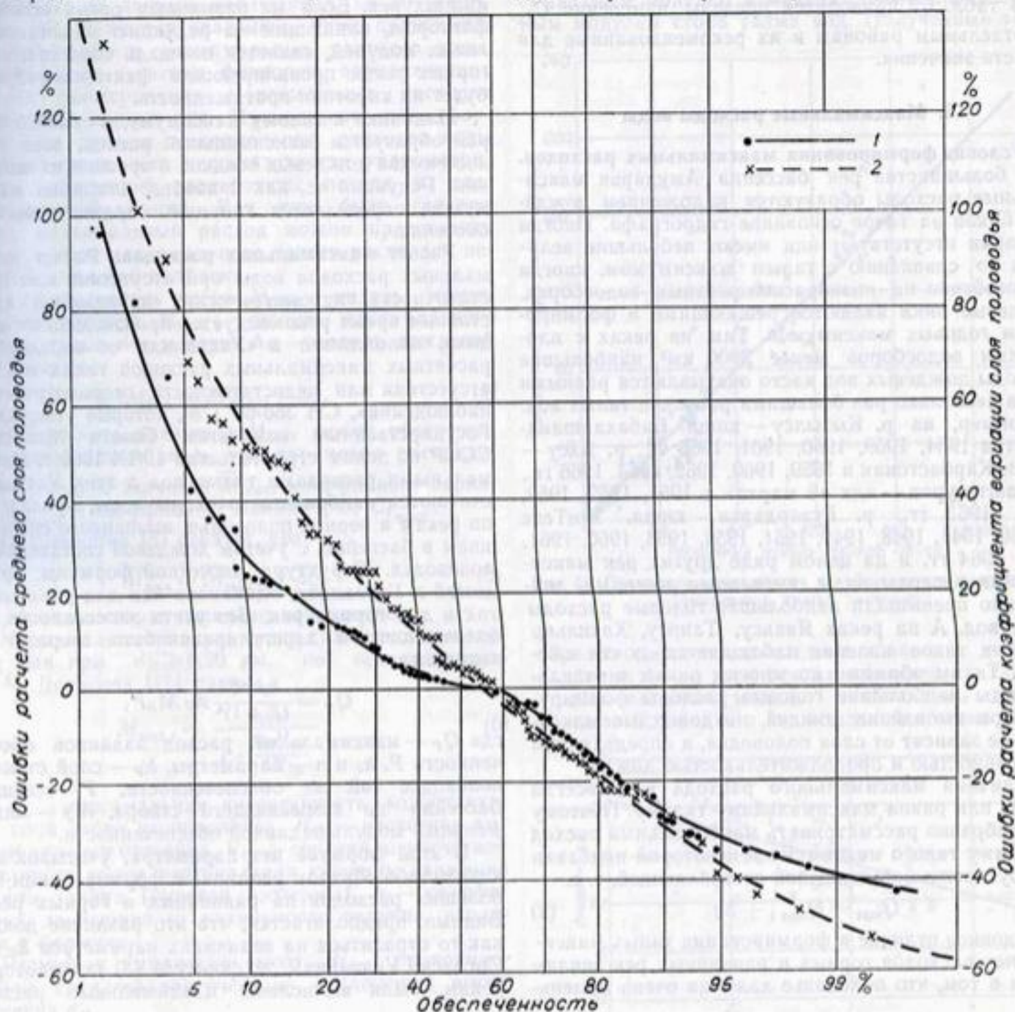
Рис. 62. Обеспеченность относительных ошибок расчета среднего слоя половодья (1) и коэффициента вариации слоя половодья (2).
