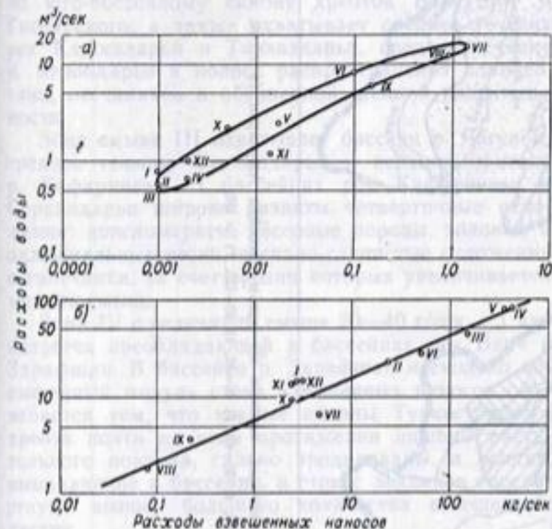
Рис. 93. Зависимость среднемесячных средних многолетних расходов взвешенных наносов от расходов воды.
