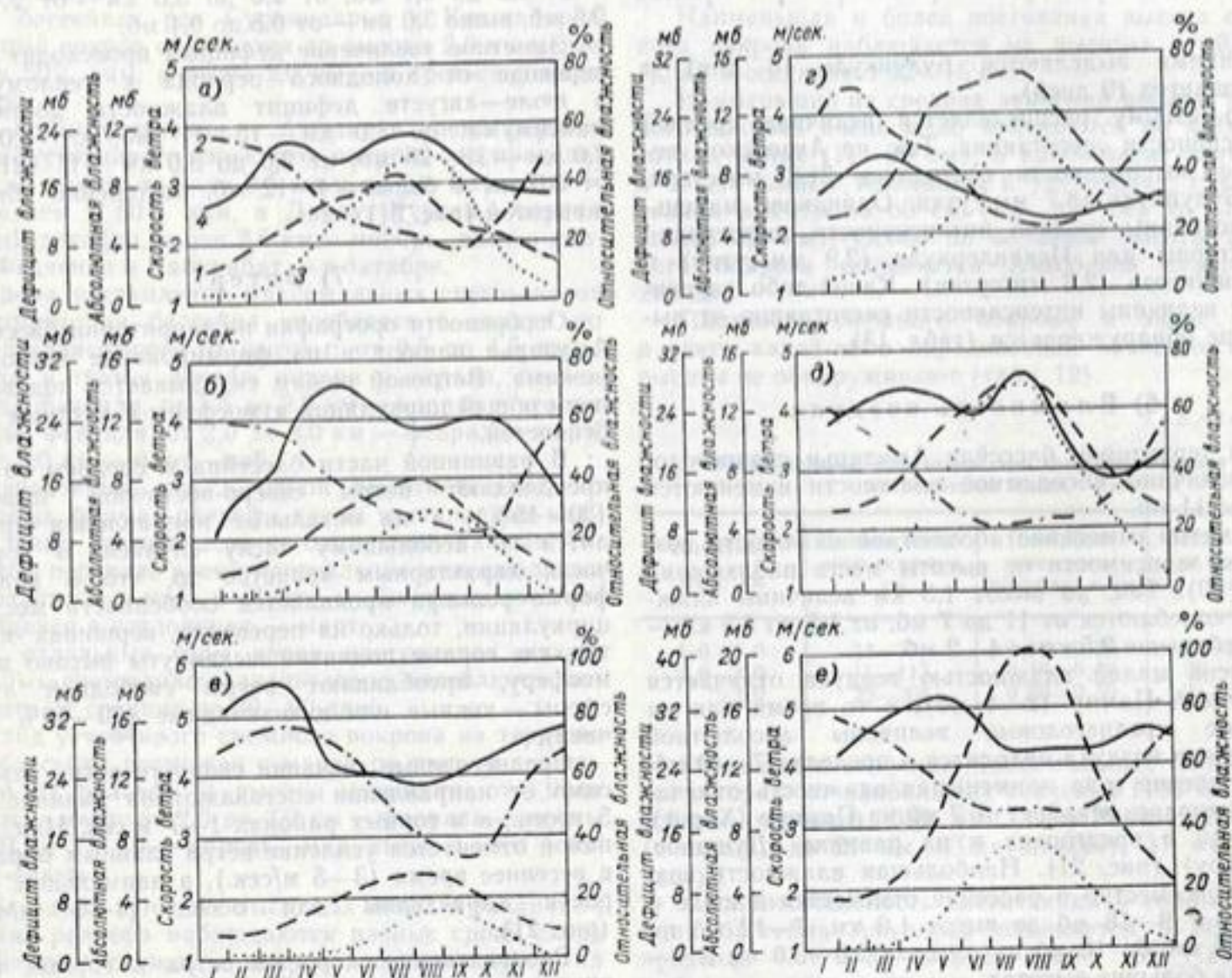
Рис. 21. Годовой ход абсолютной (1), относительной (2) влажности, дефицита влажности (3) воздуха и скорости ветра (4) в различных частях бассейна Амударьи.
