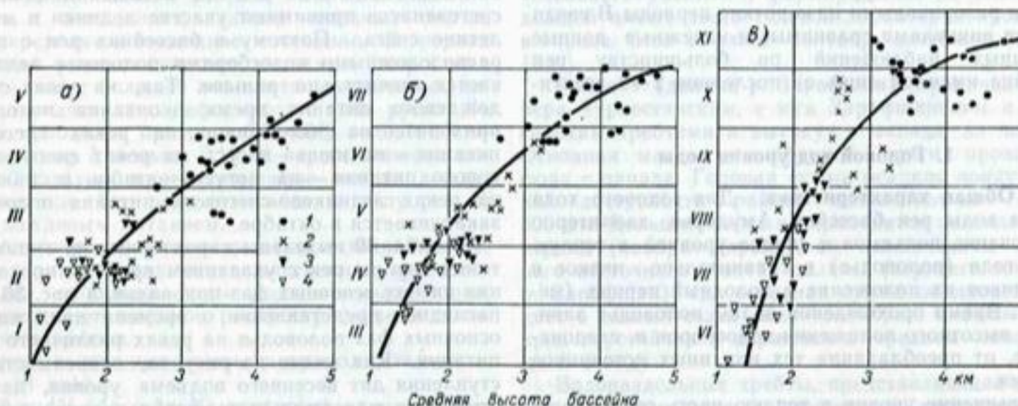
Рис. 36. Время наступления начала половодья (а), прохождения гребня половодья (б) и окончания половодья (в) на реках различного типа питания с различной средней высотой бассейна.
