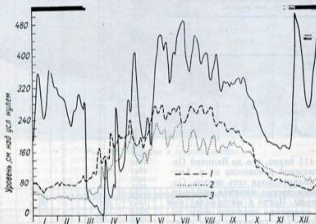
Рис. 120. Ход уровня воды в верхнем (1), среднем (2) и нижнем (3) течении р. Амударьи в 1959 г.
