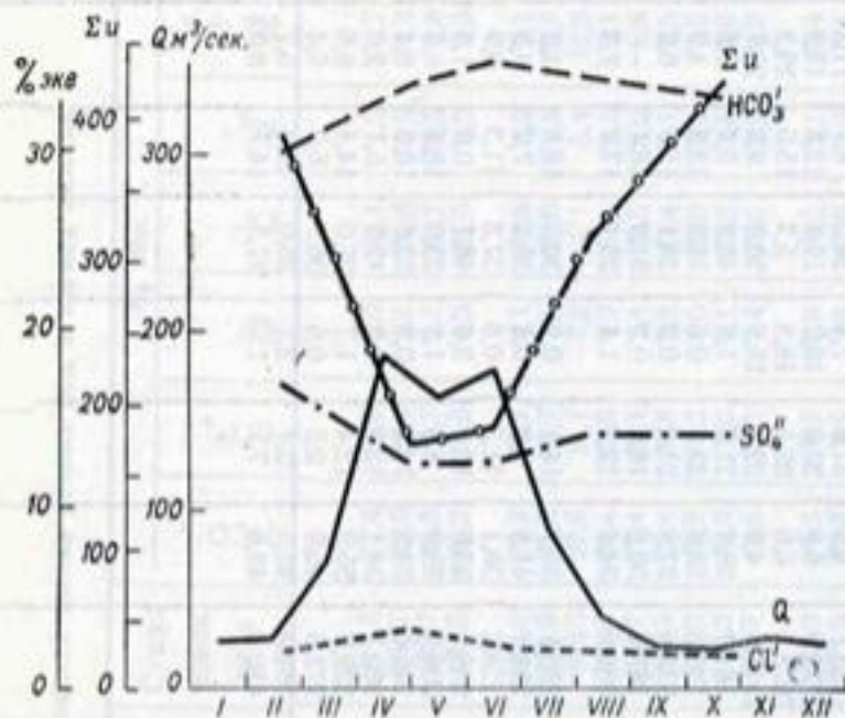
Рис. 113. Внутригодовое изменение расходов воды, минерализации и содержания главных ионов в воде р. Сурхандарьи у клх им. Жданова за 1959 г.
