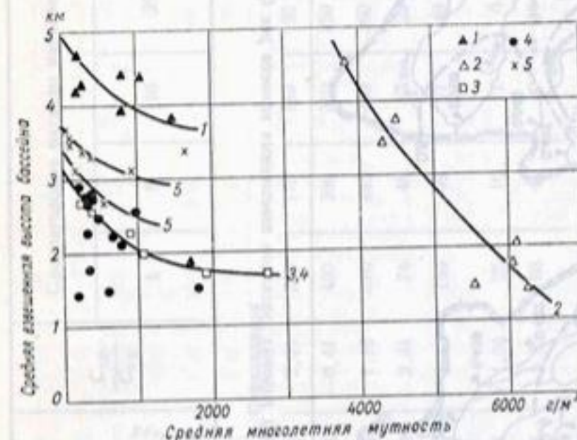
Рис. 97. Зависимость средней многолетней мутности воды в реках от средней высоты бассейнов.
