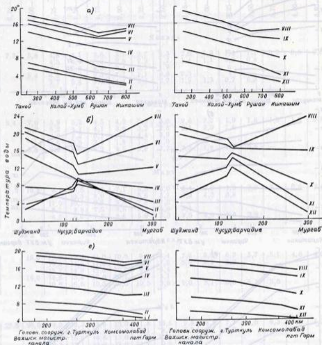
Рис. 87. Изменение среднемесячной температуры воды по длине рек Пяндж (а), Бартаг (б) и Вахш (в) (расстояние — от устья).
