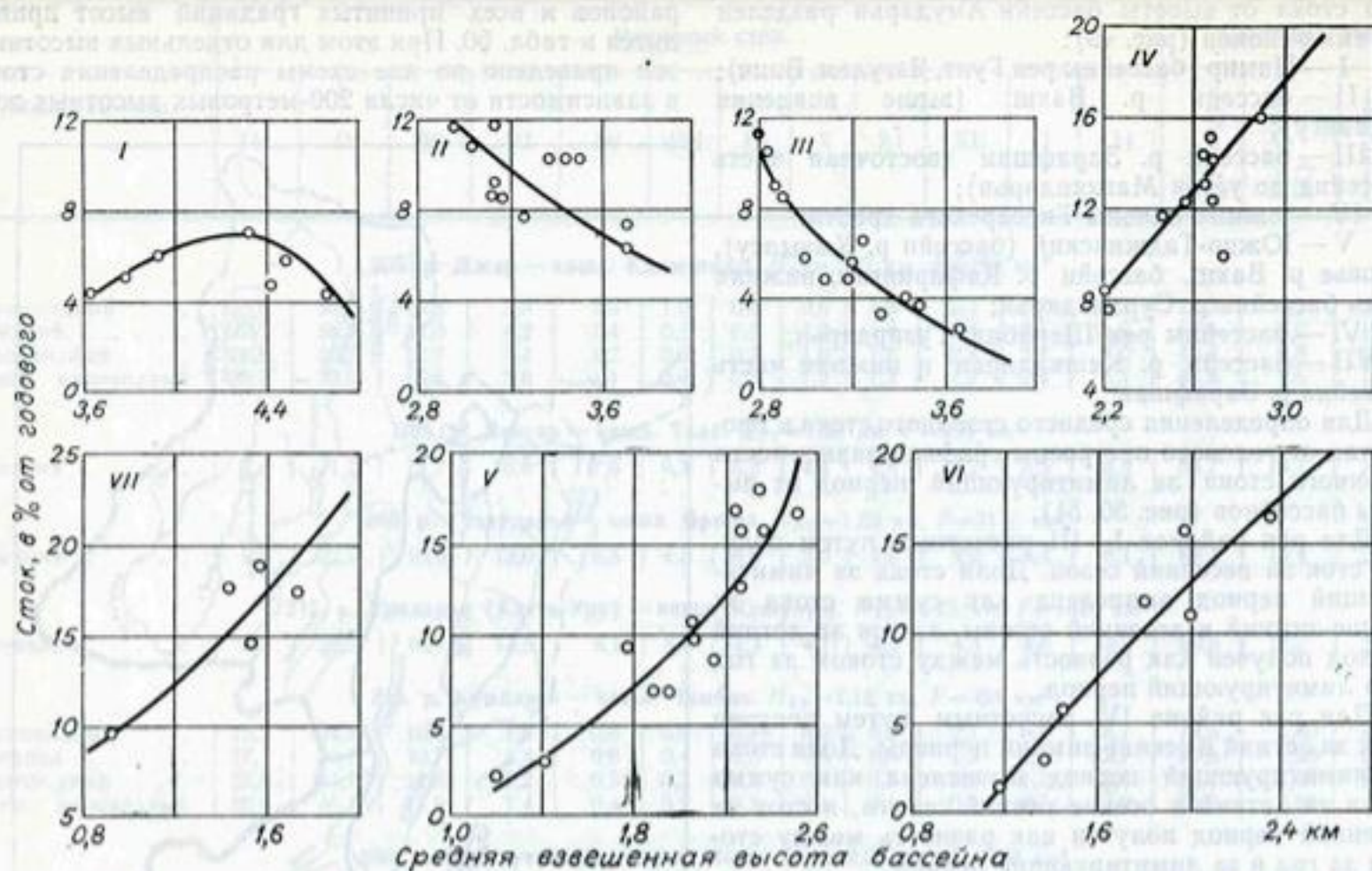
Рис. 50а. Зависимость стока за лимитирующий сезон (в % от годового) от средней взвешенной высоты бассейнов.
