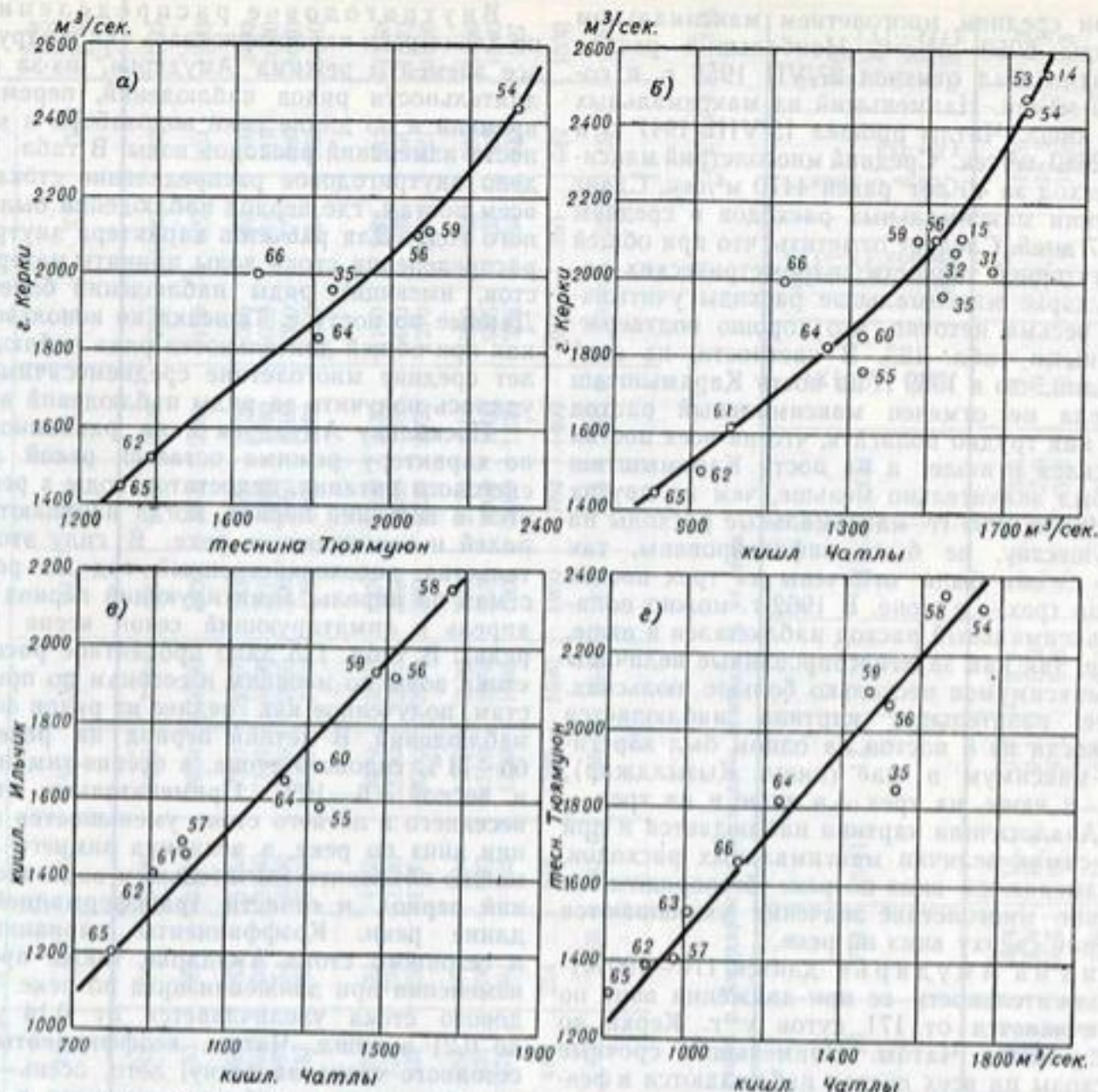
Рис. 122. Графики связи среднегодовых расходов воды по постам р. Амударьи.
