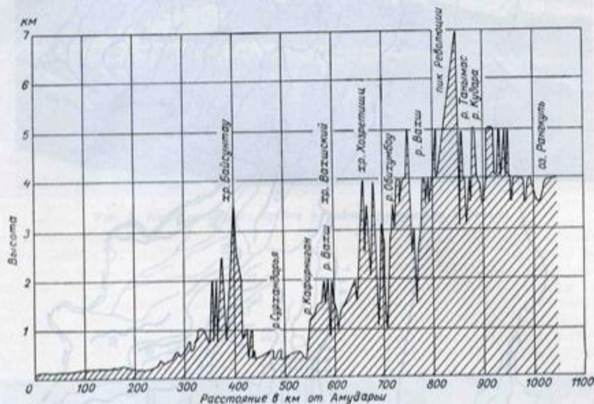
Рис. 1. Разрез рельефа бассейна по параллели 38° 30'.
