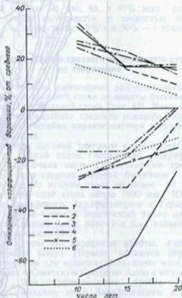
Рис. 46. Максимальные отклонения коэффициентов вариации ( C_v ) по скользящим n -летиям от C_v за фактический ряд наблюдений:
