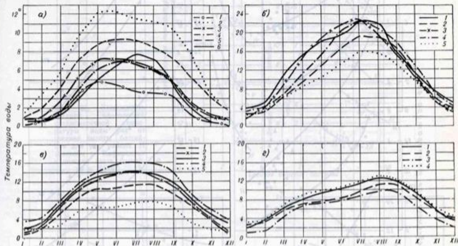
Рис. 80. Годовой ход средней многолетней среднемесячной температуры воды для рек различного типа питания.
