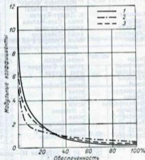
Рис. 53. Средние кривые продолжительности суточных расходов рек различных групп.
