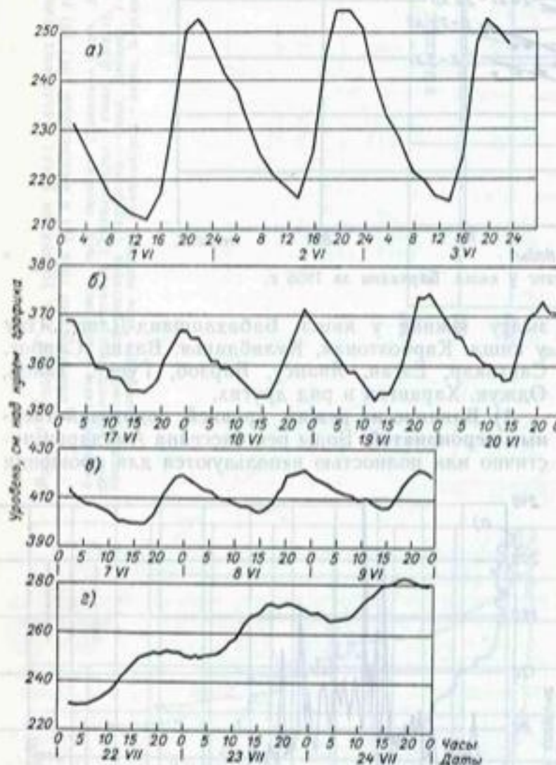
Рис. 41. Суточный ход уровня воды на реках бассейна Амударьи в характерные фазы их режима.
