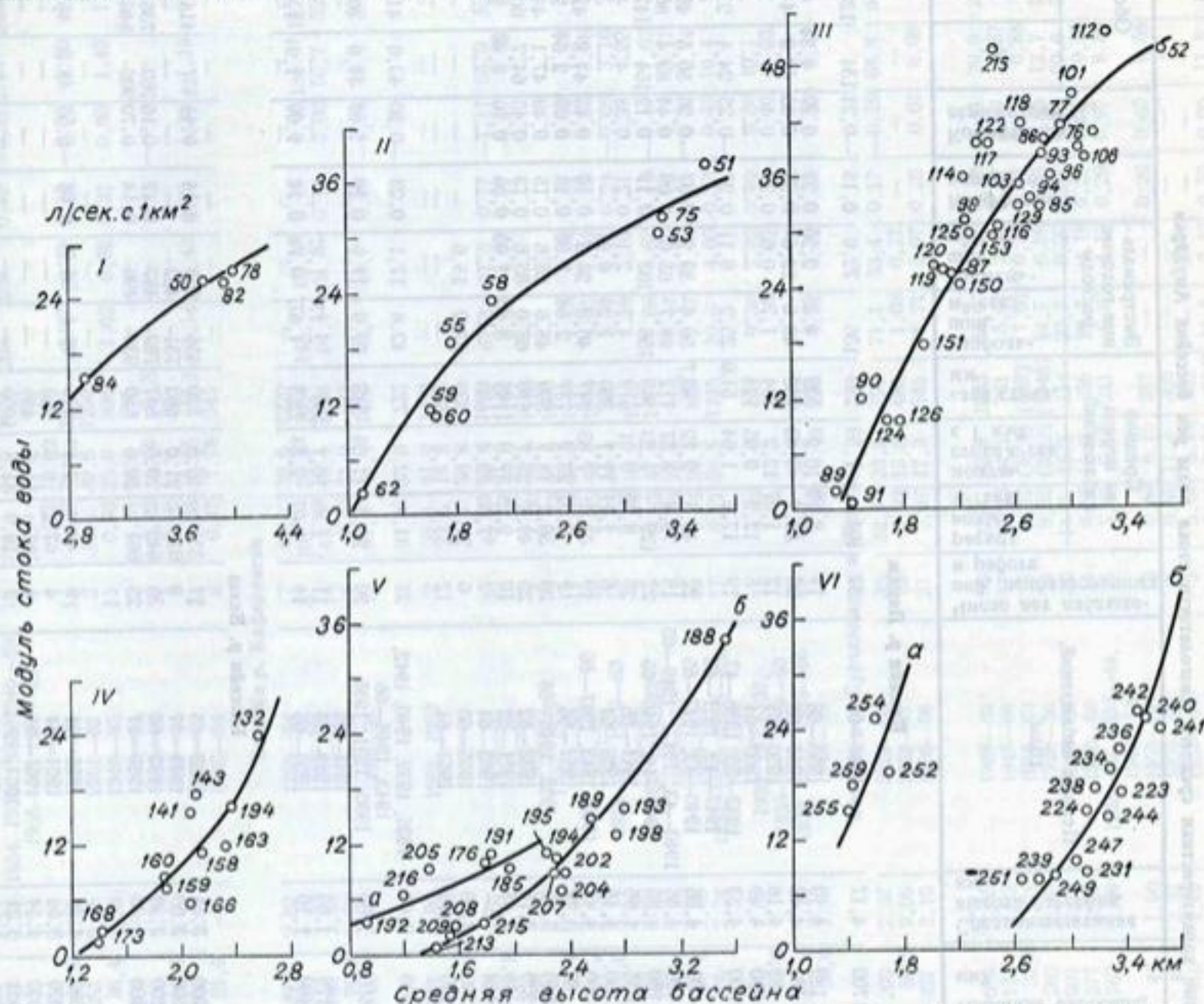
Рис. 44. Зависимость модулей стока M_0 от средней взвешенной высоты бассейнов H_{cp} по рекам бассейна Амударьи для различных районов.
