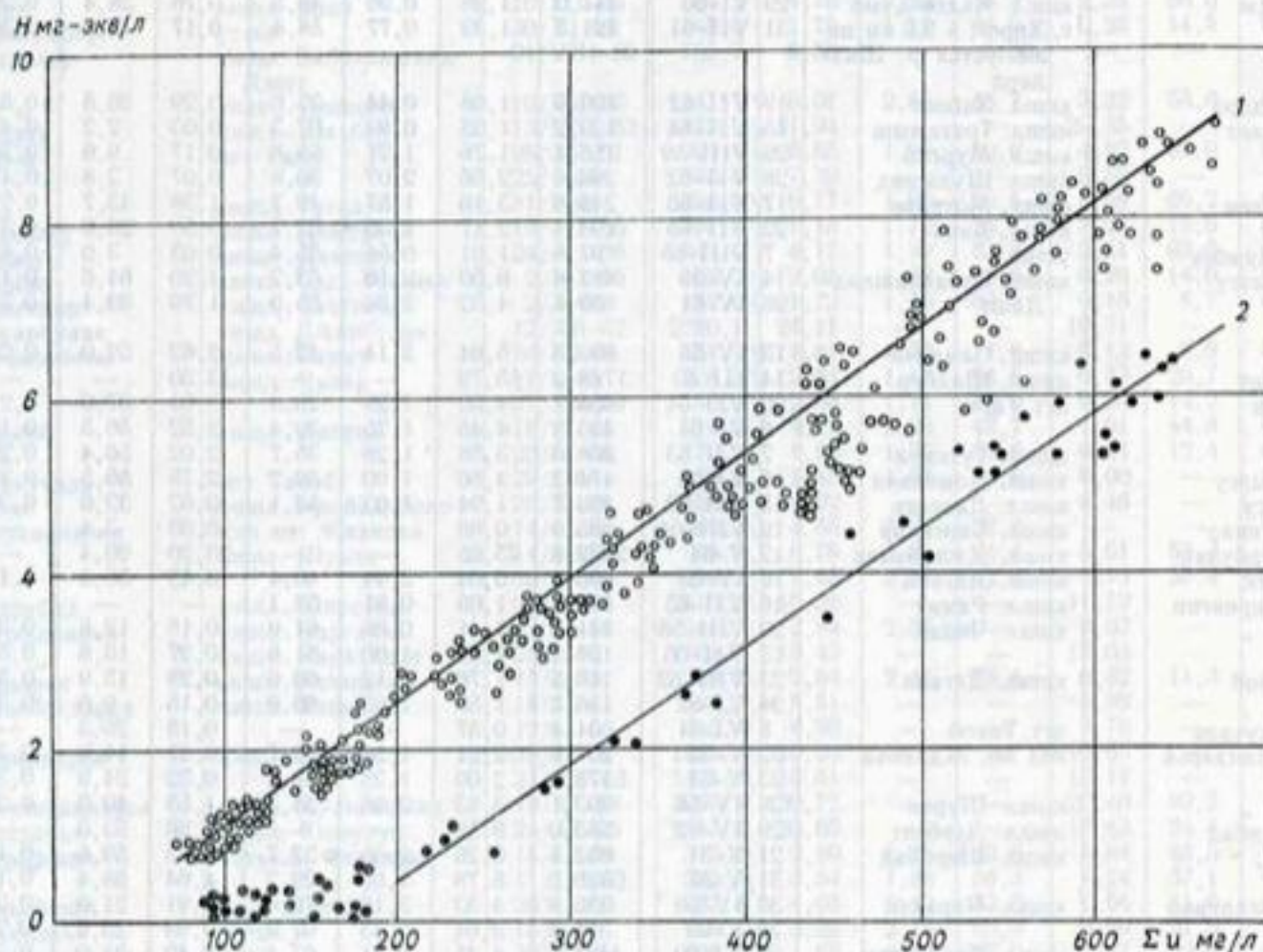
Рис. 117. Характер связи величин общей (1) и остаточной (2) жесткости с минерализацией воды в реках бассейна Амударьи.
