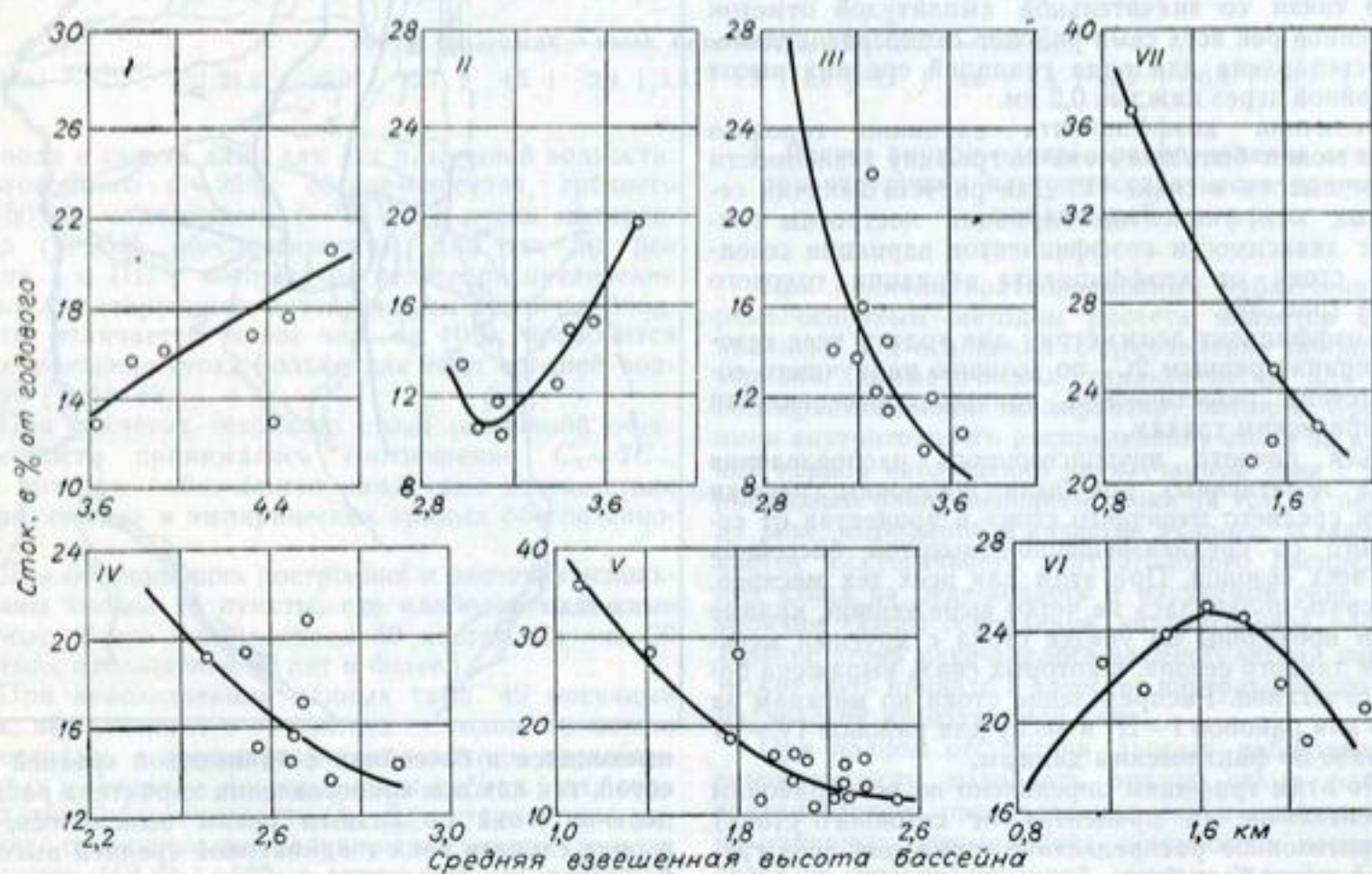
Рис. 50б. Зависимость стока за нелIMITирующий сезон (в % от годового) от средней взвешенной высоты бассейнов.
