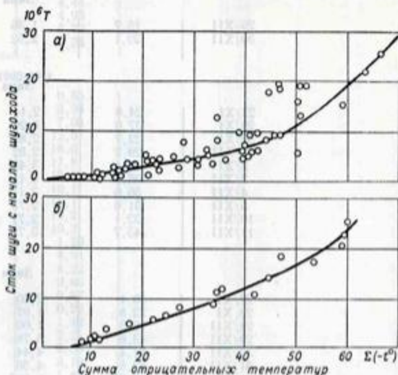
Рис. 131. Зависимость величины стока шуги за шугоход от суммы отрицательных температур для постов Чатлы (а) и Тюмуйун (б).
