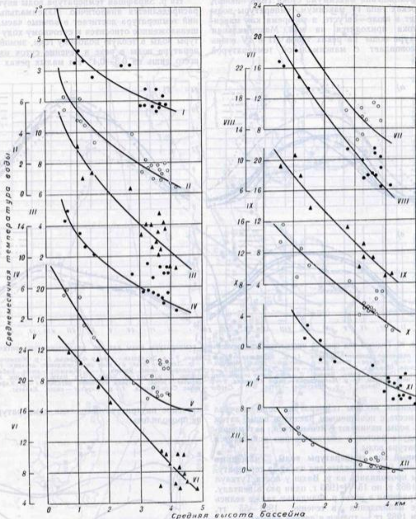
Рис. 82. Зависимость средней многолетней среднемесячной температуры воды рек от средней высоты бассейнов для рек района I (бассейн р. Пяндж и верховья р. Вахш).
