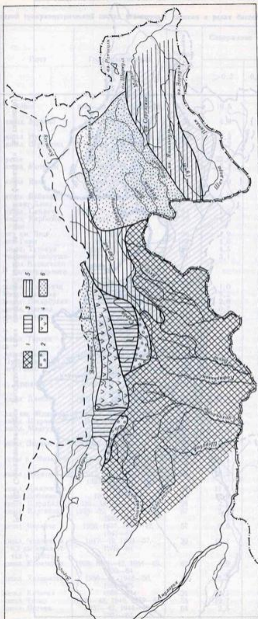
Рис. 101. Схематическая карта распределения стока взвешенных наносов за июль — сентябрь (в % годового). 1) 0—10, 2) 11—20, 3) 21—40, 4) 41—60, 5) 61—80, 6) 81—100.
