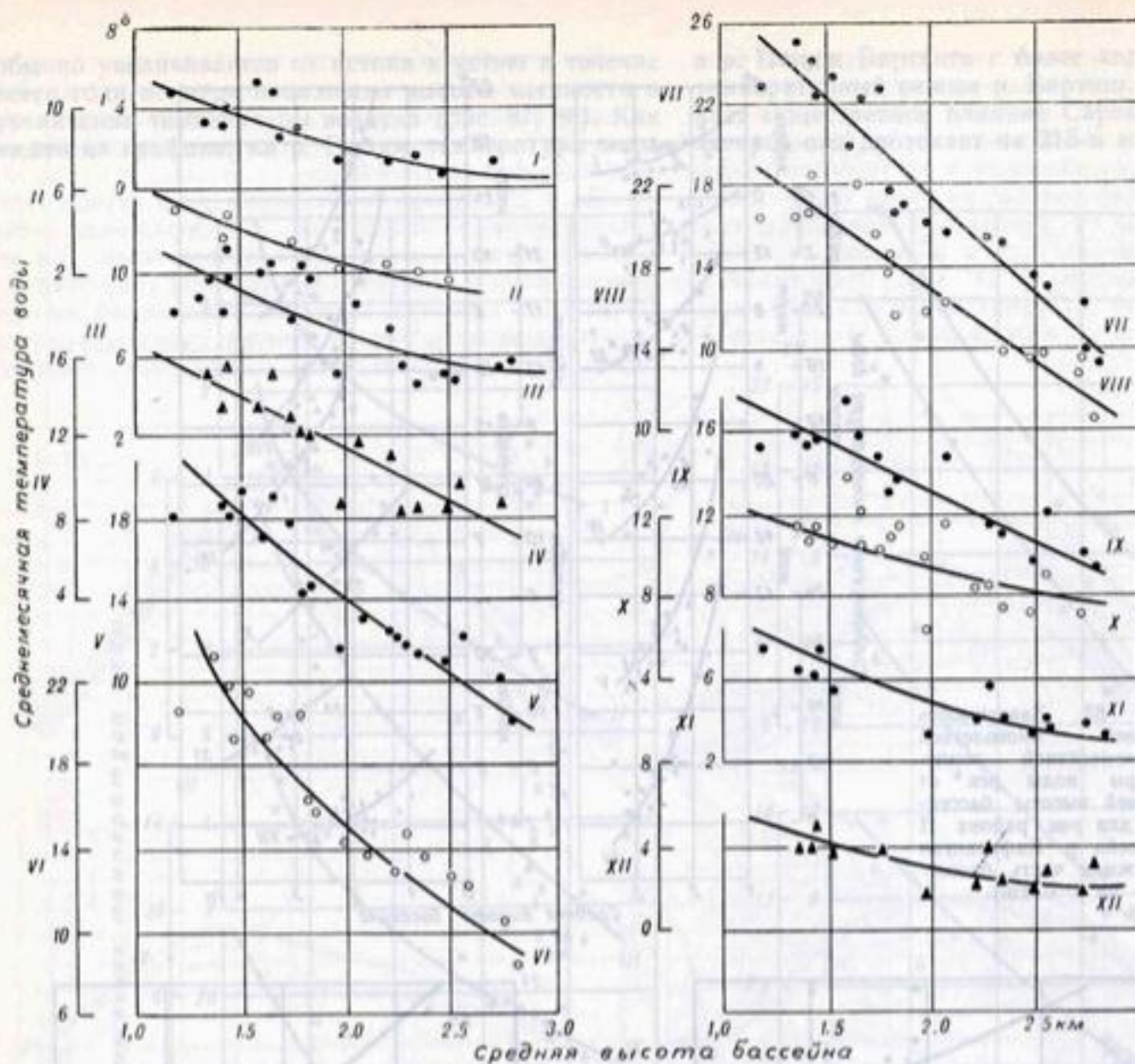
Рис. 85. Зависимость средней многолетней среднемесячной температуры воды рек от средней высоты бассейнов для района IV (бассейны рек Шерабад и Кашкадарья).
