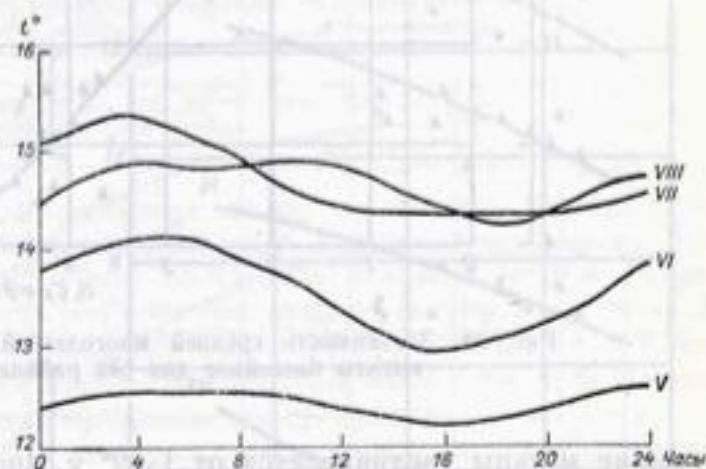
Рис. 81. Суточный ход температуры воды в р. Вахш у кишла. Туткаул в мае—августе 1952 г.
