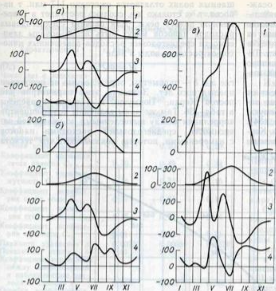
Рис. 124. Изменение элементов водного баланса Амударьи по месяцам.
