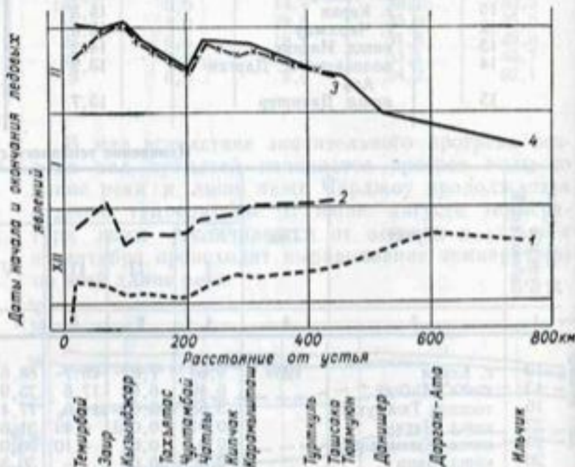
Рис. 129. Характер изменения дат начала (1) и окончания (4) ледовых явлений, начала (2) и окончания (3) ледостава по длине р. Амударьи.
