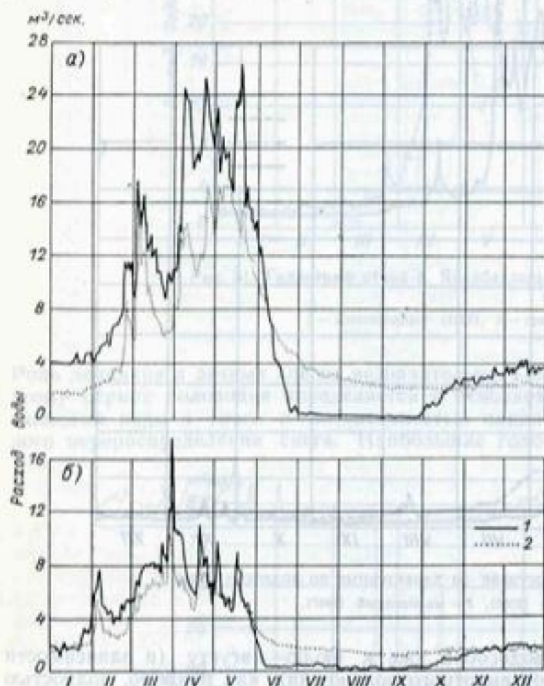
Рис. 34. Гидрограф стока р. Кашкадарьи в верхнем (1 — кишл. Варганза) и нижнем (2 — кишл. Каратикон) течении за многоводный — 1960 (а) и маловодный 1947 (б) годы.
