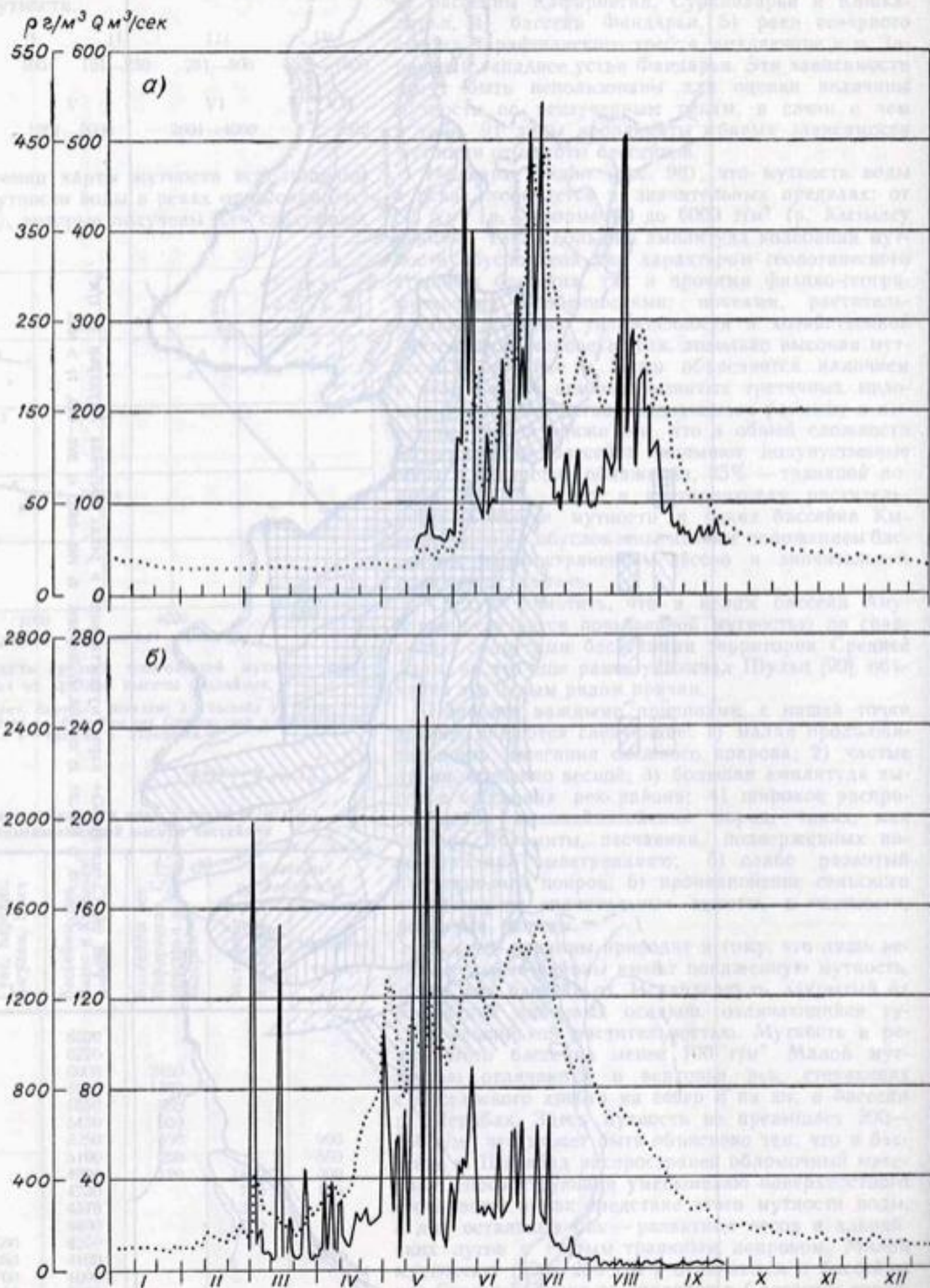
Рис. 99. Хронологические графики хода а — р. Гунт — г. Хорог, б — р. Варзоб — кишл. Даганата.
