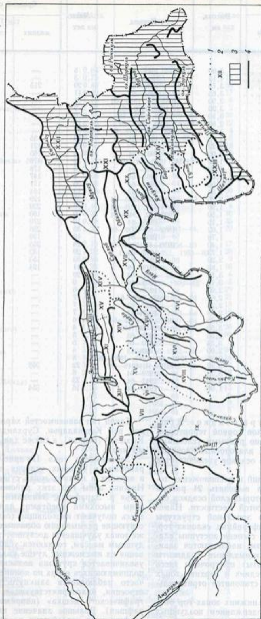
Рис. 14. Районирование территории бассейна Амударьи по характеру зависимости осадков от высоты места. 1 — границы районов, 2 — номера районов, 3 — территория с весенне-летним максимумом осадков, 4 — горные хребты.
