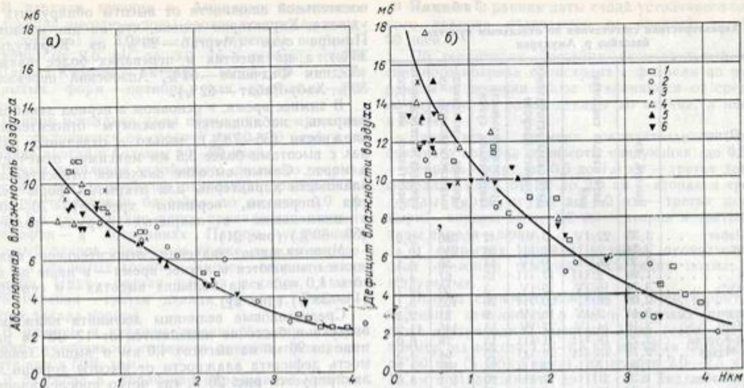
Рис. 20. Зависимость абсолютной влажности (а) и дефицита влажности (б) воздуха от высоты места. 1 — бассейны р. Пяндж, 2 — бассейны р. Вахш, 3 — бассейны р. Кафирниган, 4 — бассейны р. Сурхандарья, 5 — бассейны р. Кашкадарья, 6 — бассейны р. Зарафшан.
