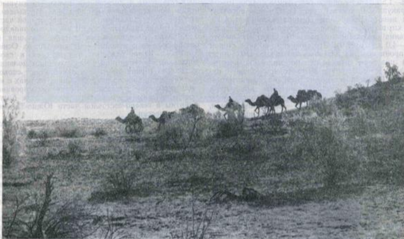
Рис. 7. Характер рельефа и растительности в Кызылкумах.
