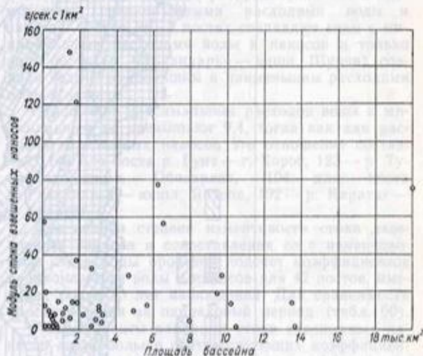
Рис. 94. Зависимость среднего многолетнего модуля стока взвешенных наносов от площади бассейна.
