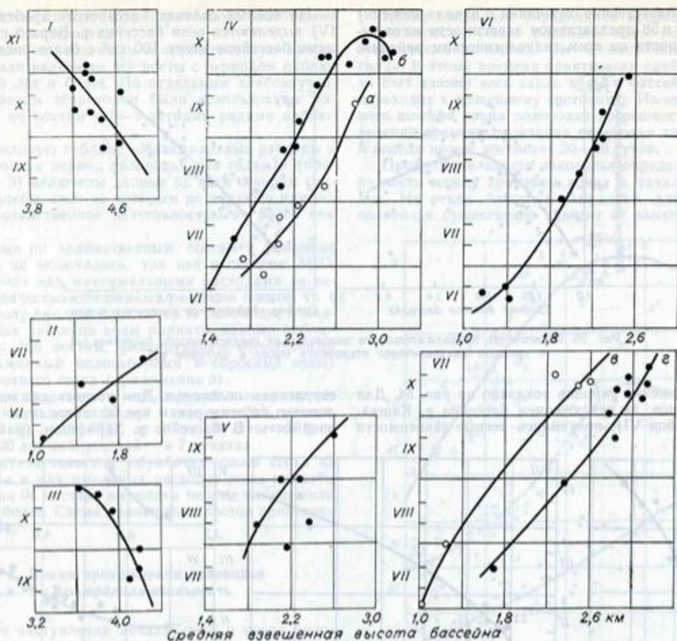
Рис. 58. Зависимость средних многолетних дат окончания половодья от средних высот бассейнов.
