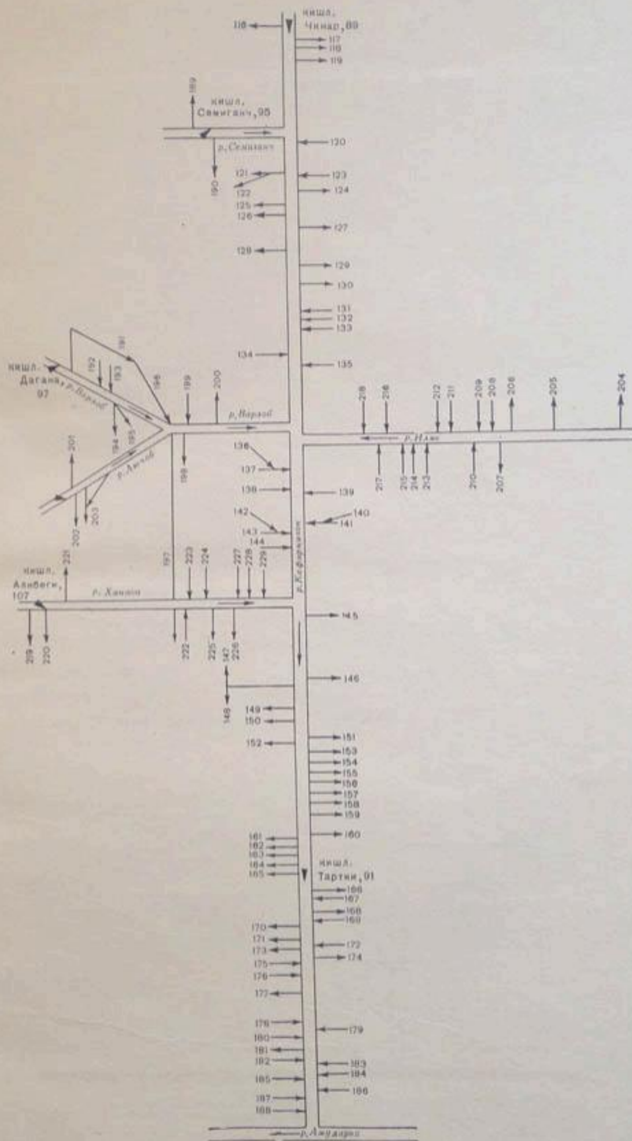
Рис. 5. Схема расположения водозаборов, коллекторов и сбросов в бассейне р. Кафиринган.
