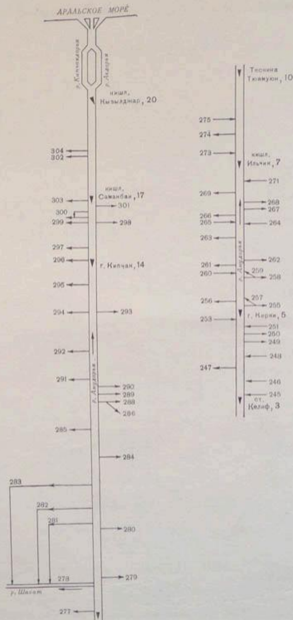
Рис. 6. Схема расположения водозаборов, сбросов и коллекторов в бассейне р. Аму-Дарья от ст. Келыф до Аральского моря.
