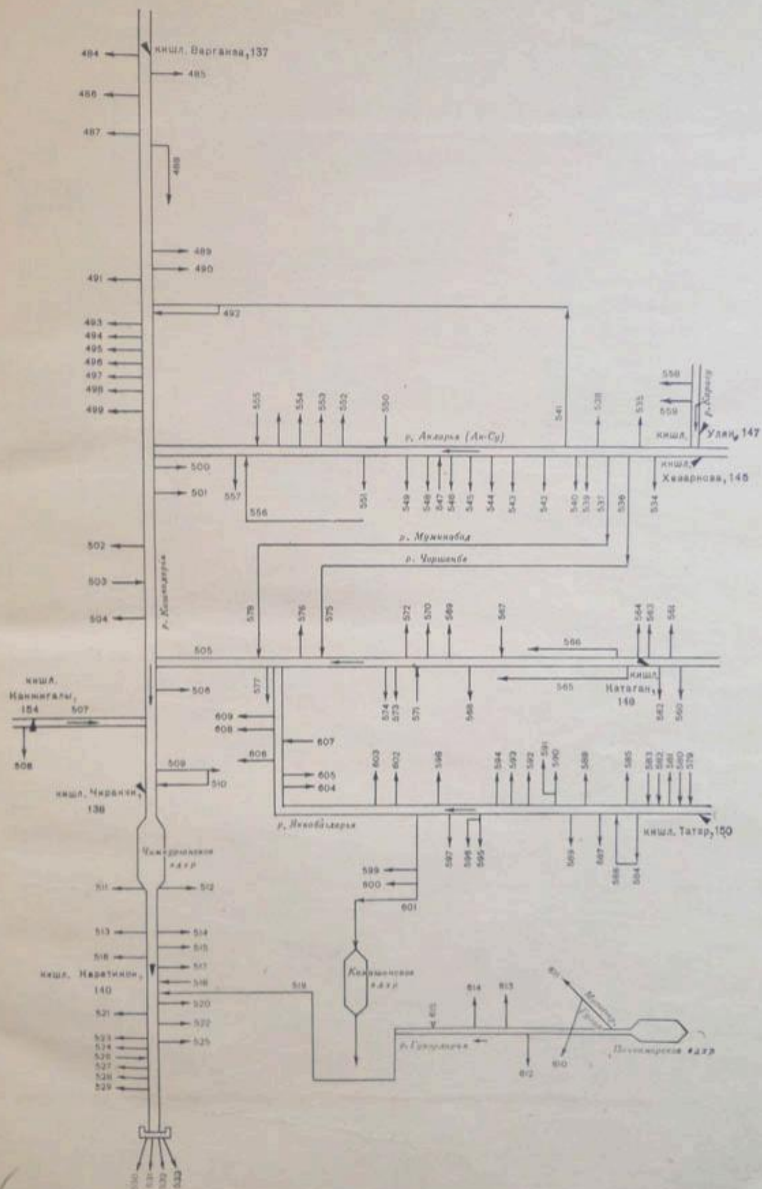
Рис. 8. Схема расположения водозаборов и сбросов в бассейнах рек Кашкадарья, Джинодарья, Акдарья, Ташкентдарья, Якубовдарья и Гузардарья.
