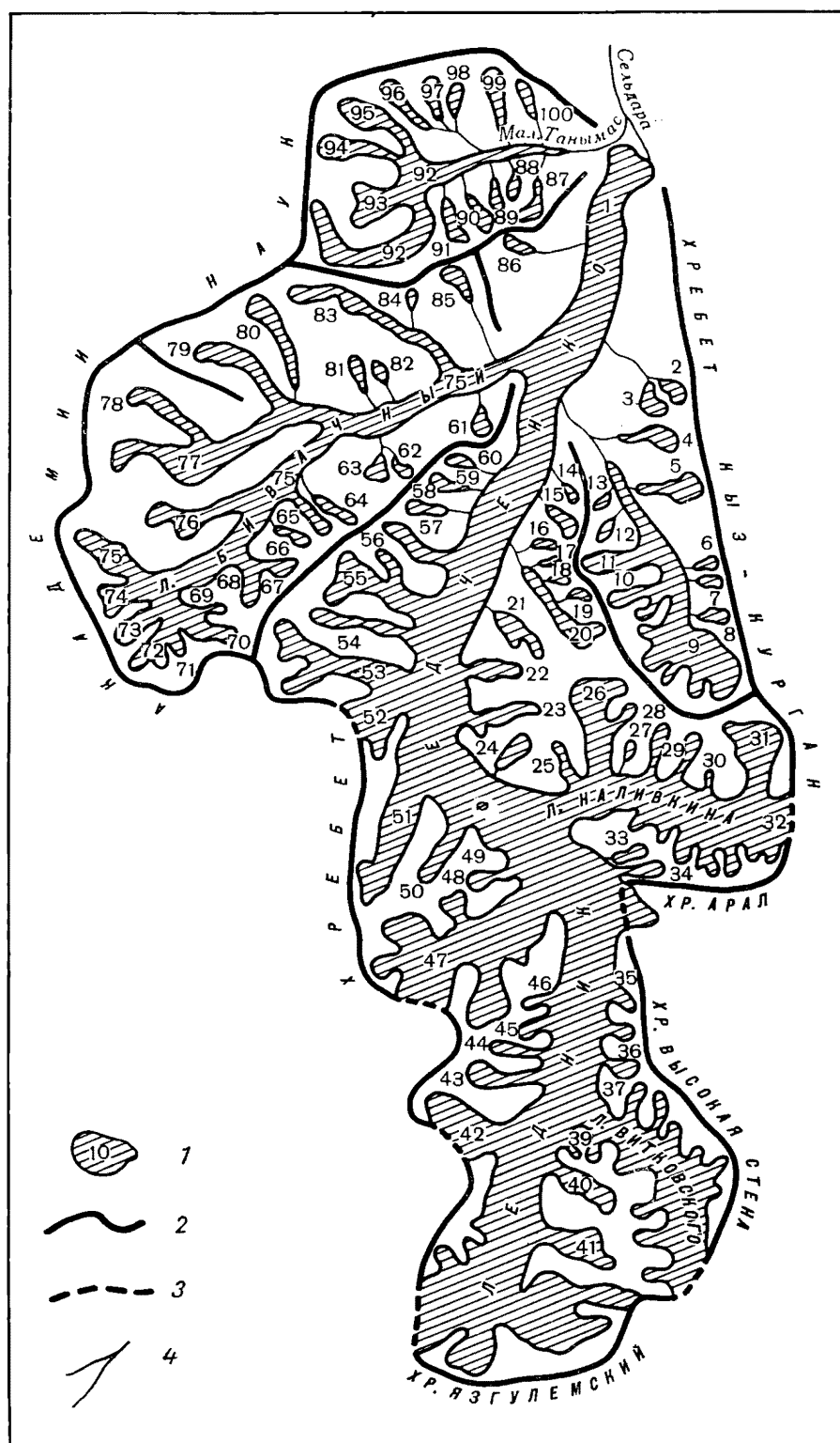
Рис. 3. Схема расположения ледников в бассейне р. Муксу (А — система ледника Федченко).
