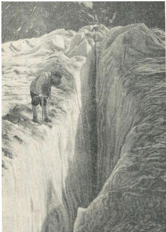
Рис. 21. Ледниковая трещина в среднем течении ледника Федченко.
