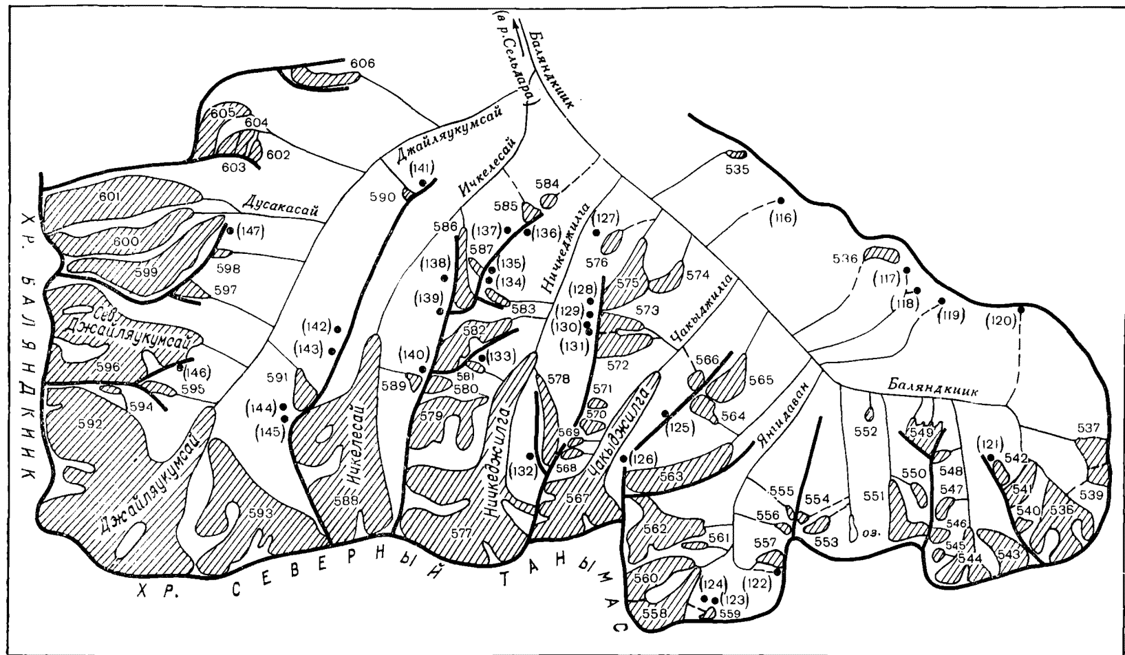
Рис. 25. Схема расположения ледников в верховьях р. Баяндзик.
