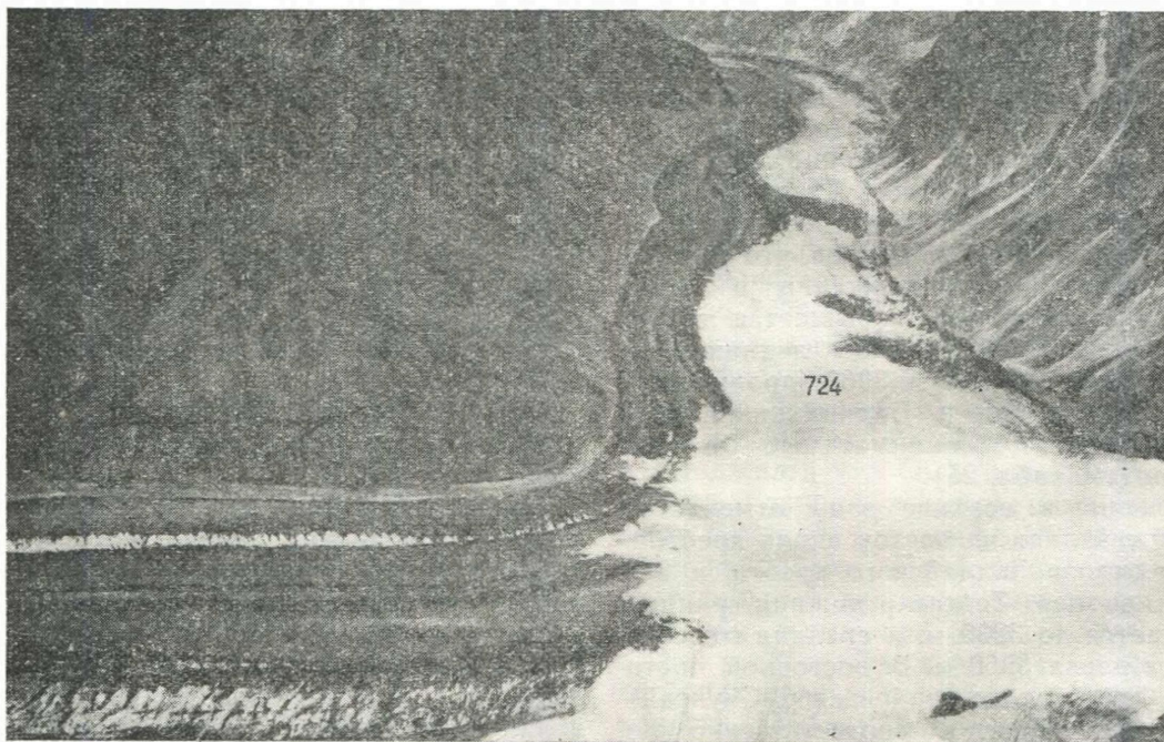
Рис. 15. Средняя часть ледника Фортамбек (№ 724). В правом нижнем углу возрожденный ледник за счет обвалов с ледопада Трамплинного. Фото В. А. Рудакова и Л. В. Десина.
