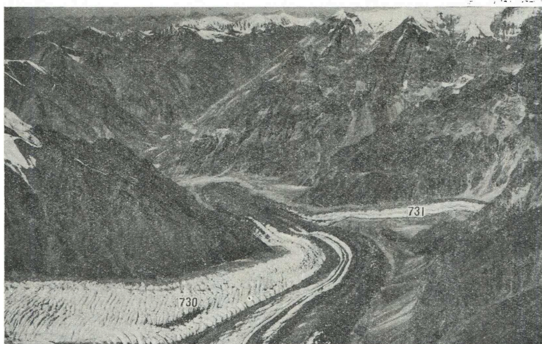
Рис. 44. Языки ледников Вальтера (№ 730) и Москвина (№ 731). Внизу долина р. Фортамбек, Фото В. А. Рудакова и Л. В. Десинова.
