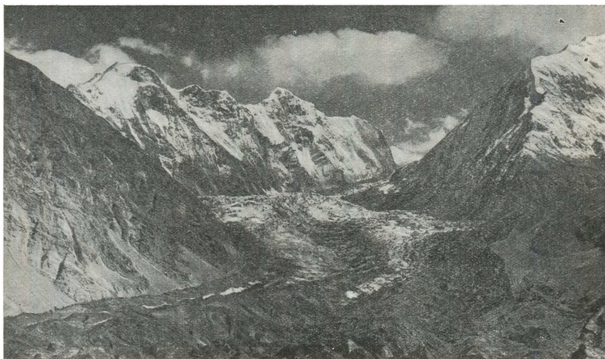
Рис. 42. Кинематическая волна на леднике Мушкетова (Карасель) (№ 710). Фото Г. В. Калинина.
