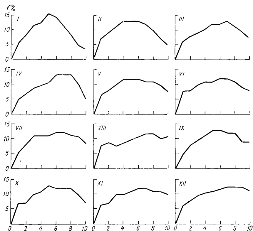
Рис. 11. Среднее относительное распределение площади ледников f^0_{\%} различных морфологических типов по 10 высотным интервалам.
