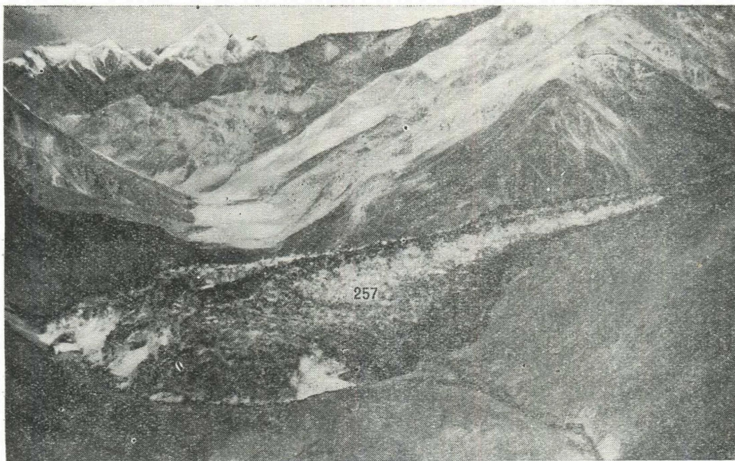
Рис. 6. Ледник Вали (№ 257) перекрывает долину р. Сауксай (вид вниз по долине). Фото В. А. Рудакова и Л. В. Десинова.
