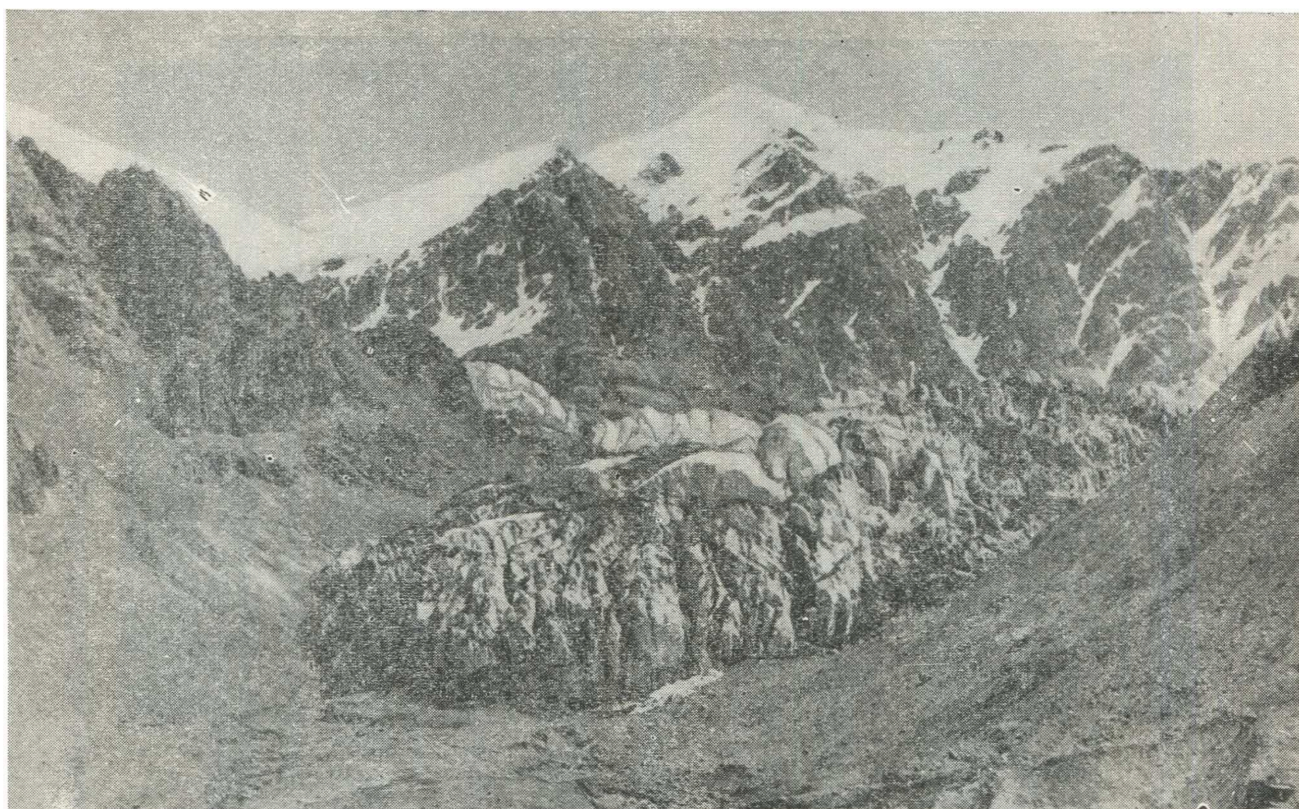
Рис. 36. Поверхность ледника № 219 в бассейне р. Чакманташ. Фото Л. В. Десичова.
