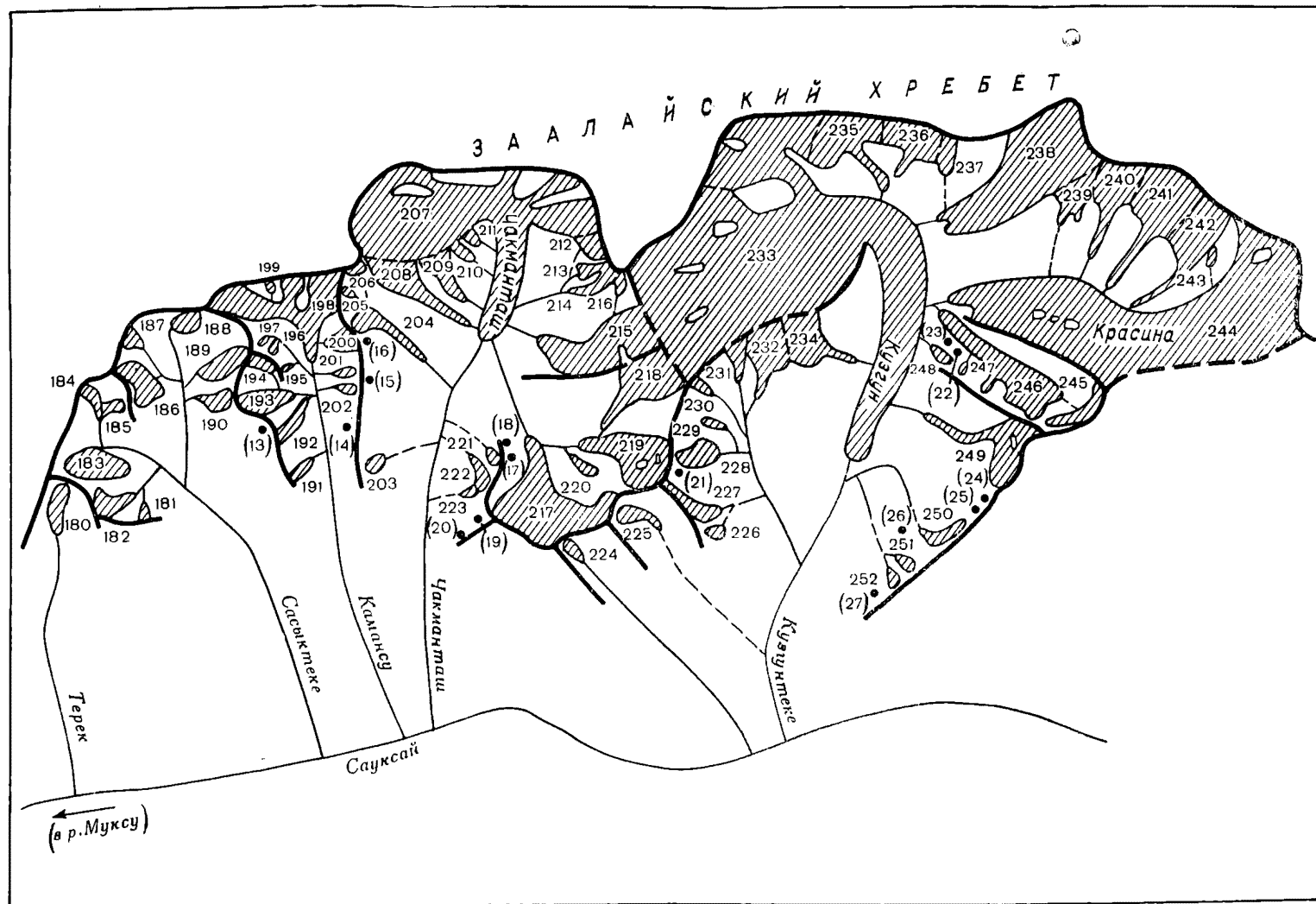
Рис. 19. Схема расположения ледников в бассейнах рек Терек, Сасыктык, Камансу, Чакманташ и Кузгунтеке. Усл. обозначения см. на рис. 18.
