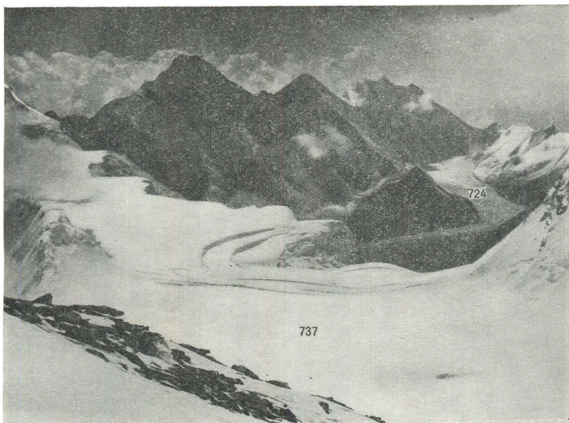
Рис. 13. Западная часть Памирского фирнового плато (№ 737). Трещины оконтуривают ледопад Трамплинный. На заднем плане левая ветвь ледника Фортамбек (№ 724) ледник Турамыс. Фото Г. В. Калинина.
