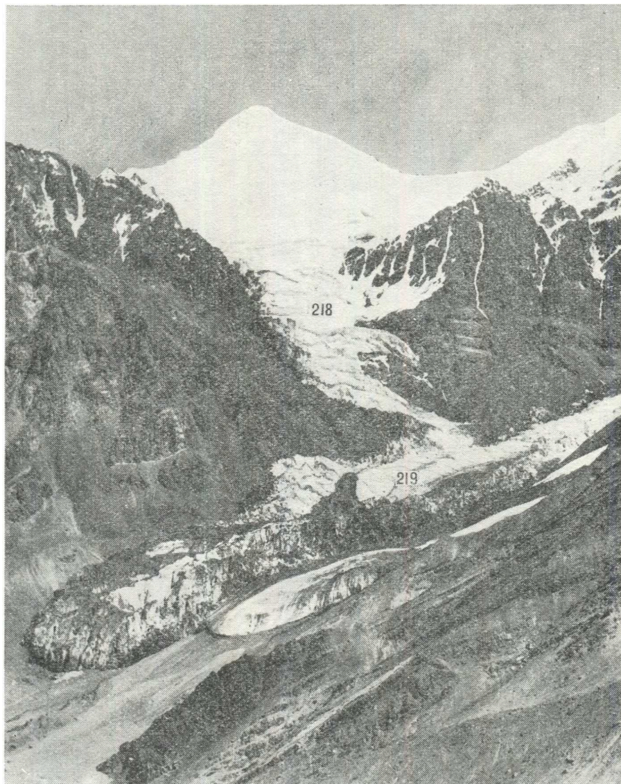
Рис. 35. Ледники бассейна р. Чакманташ (№ 218 и 219). Фото Л. В. Десинова.
