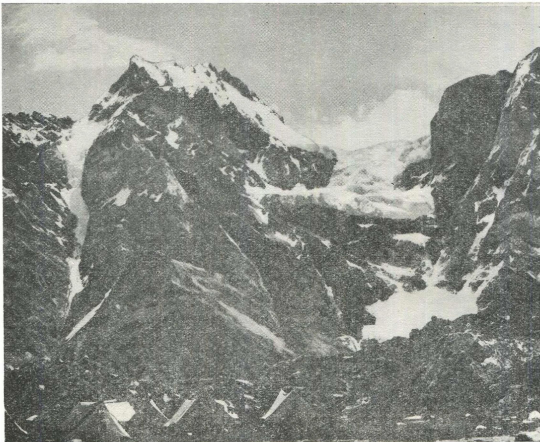
Рис. 14. Ледопад Трамплинный — сброс с Памирского фирнового плато. Фото Г. В. Калинина.
