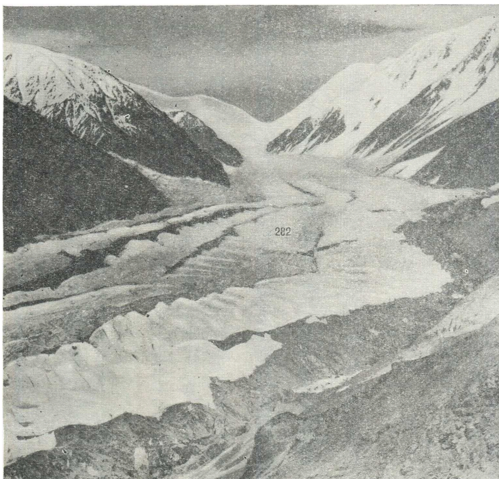
Рис. 9. Поверхность ледника Большой Саукдара (№ 282). Фото В. И. Рацка.
