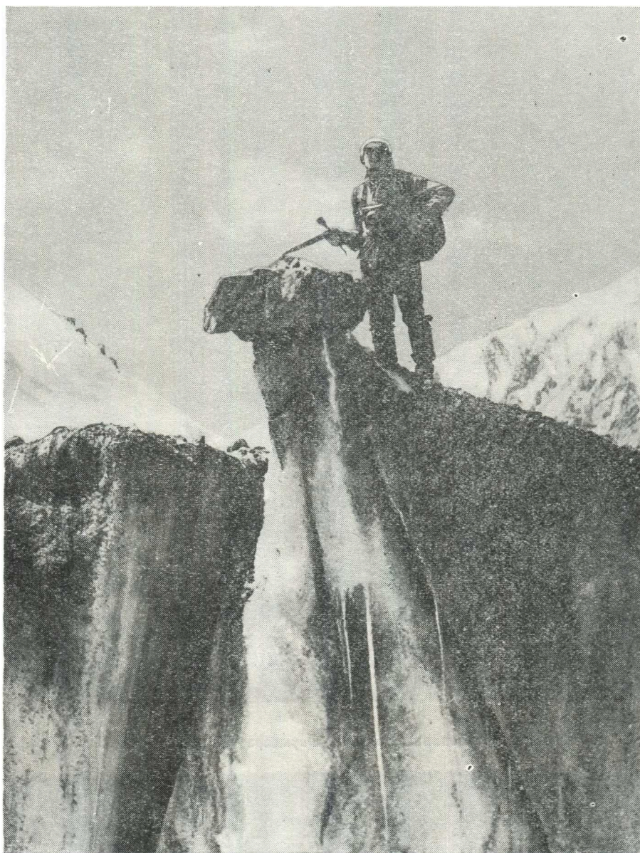
Рис. 38. Трещины и ледниковый стол на поверхности ледника Большой Саукдара (№ 282). Фото Л. В. Десинова.
