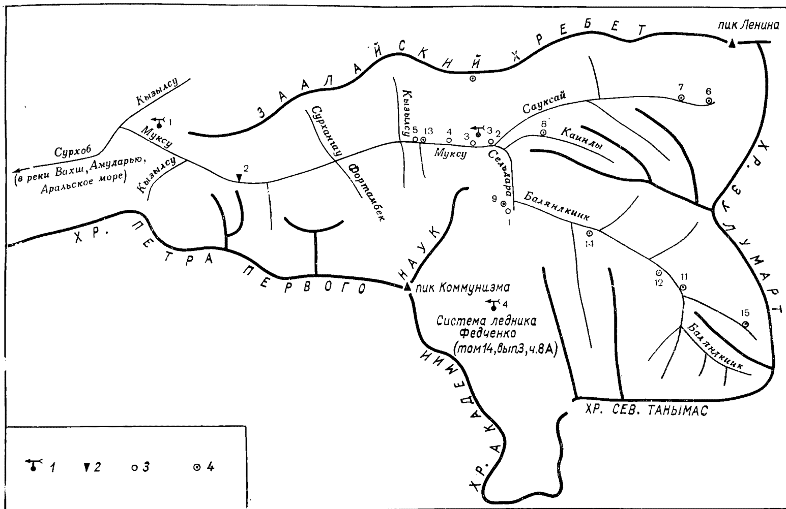
Рис. 32. Схема расположения метеорологических станций и гидрологических постов, осадкомеров и снегомерных пунктов в районе ледников. 1 — метеорологическая станция, 2 — гидрологический пост, 3 — снегомерный пост, 4 — суммарный осадкомер.
