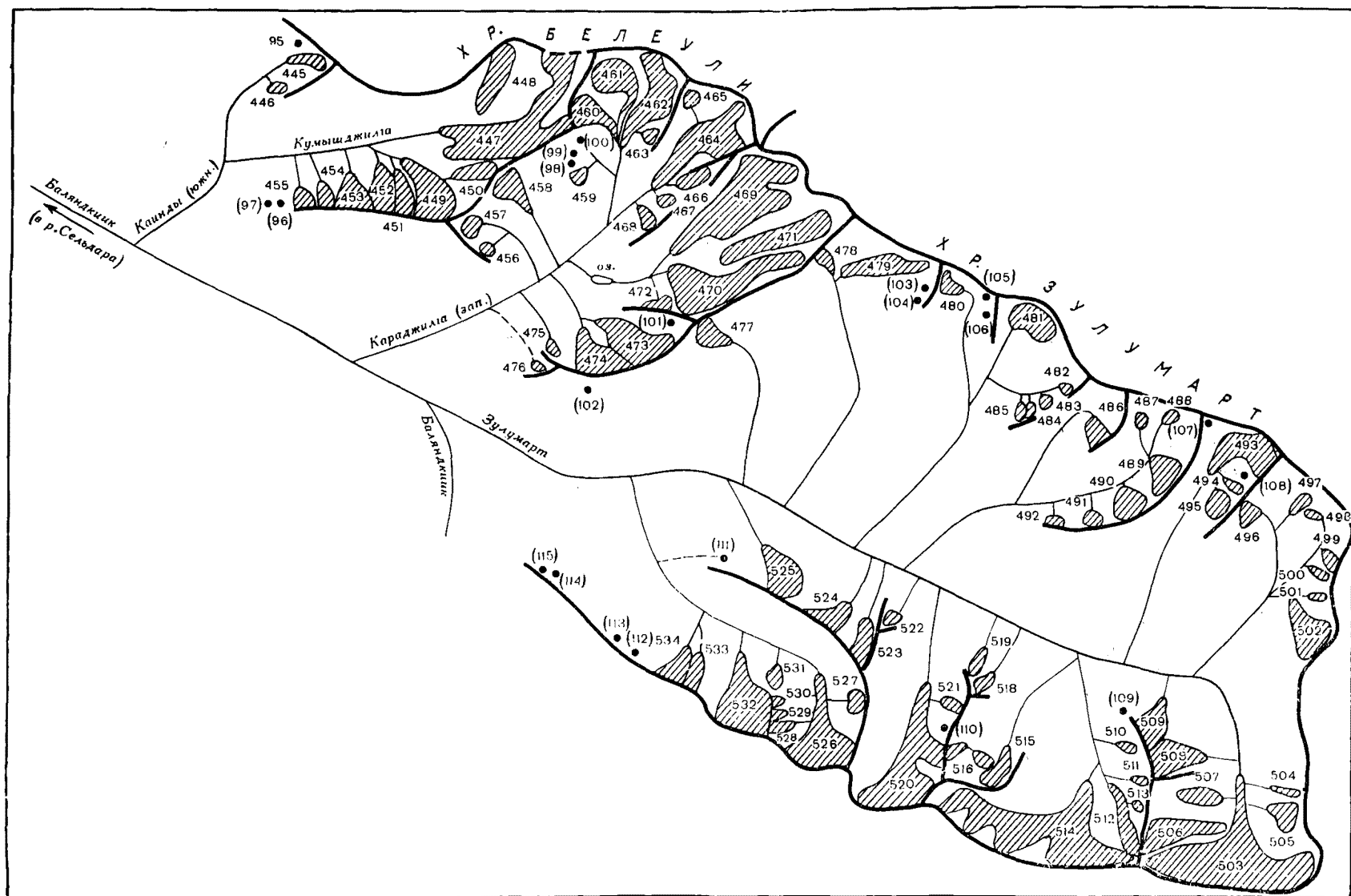
Рис. 24. Схема расположения ледников в бассейнах правых притоков р. Баландик.
