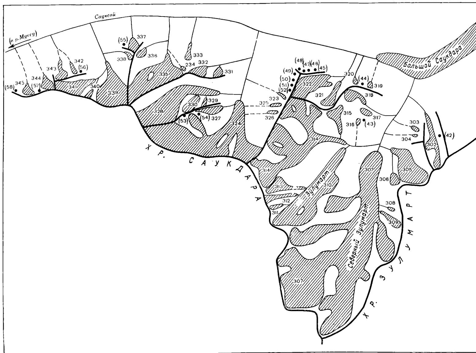
Рис. 21. Схема расположения ледников в бассейнах левых притоков р. Сауксай. Усл. обозначения см. на рис. 18.
