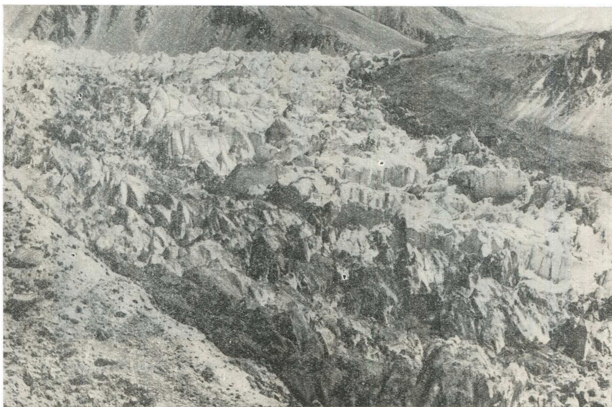
Рис. 37. Поверхность ледника Дзержинского (№ 265). Фото Л. В. Десинова.
