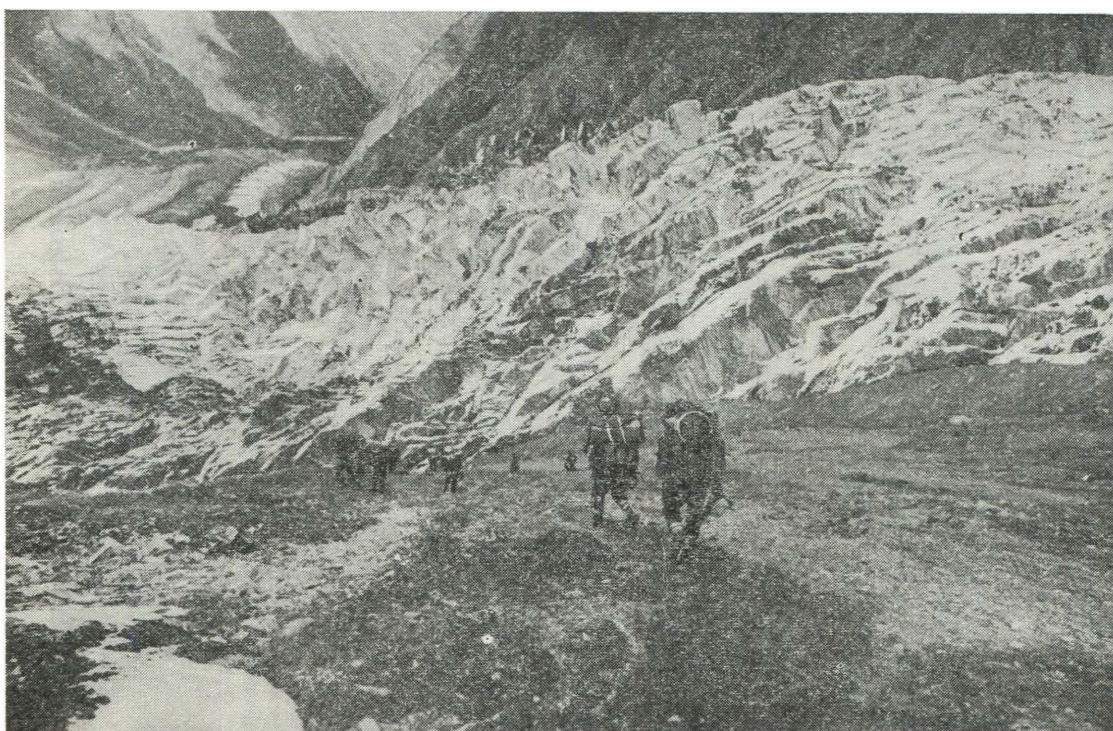
Рис. 43 Среднее течение ледника Мушкетова (Карасель) (№ 710). Вид вниз по долине. Фото Г. В. Калинина.
