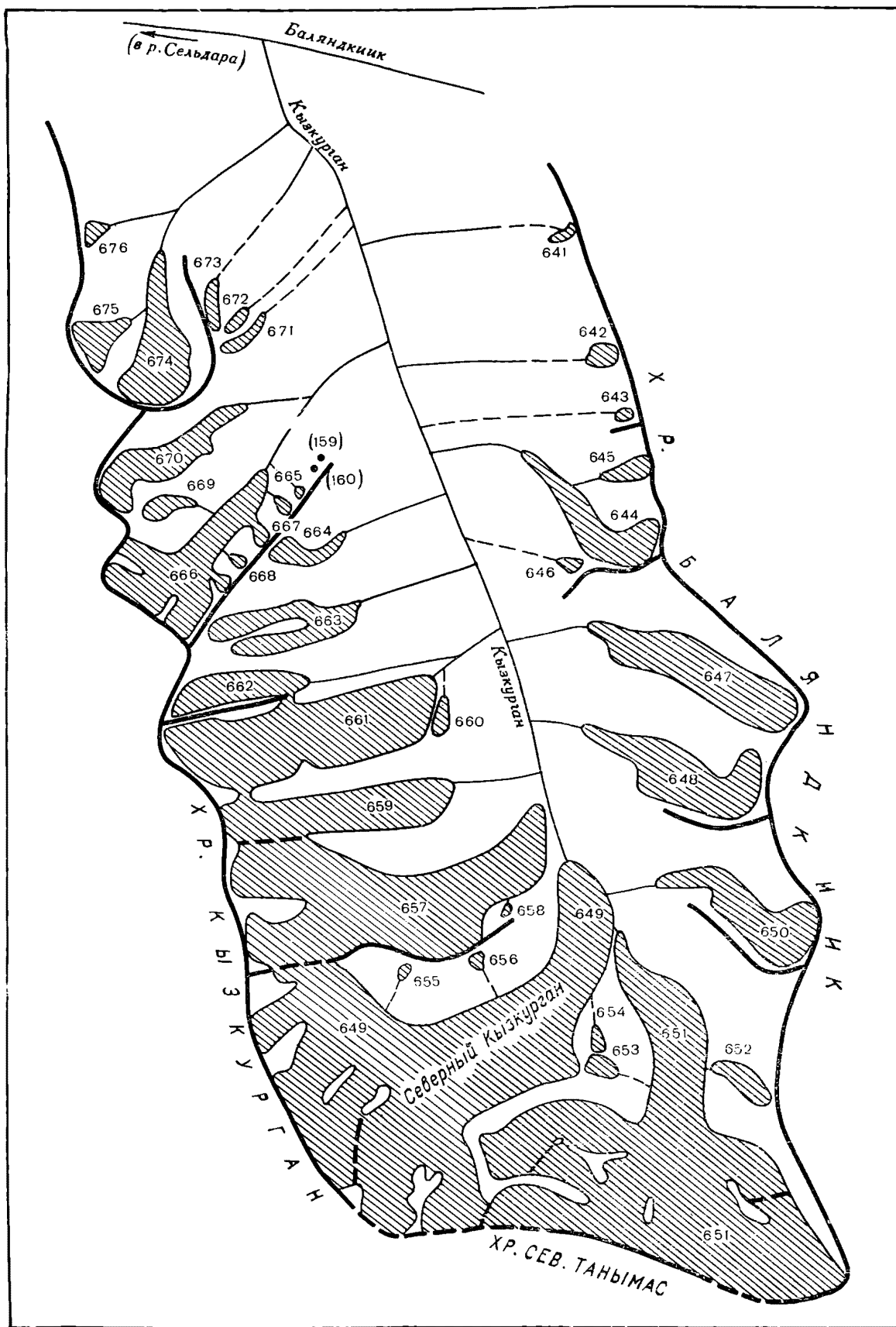
Рис. 27. Схема расположения ледников в бассейне р. Кызурган.
