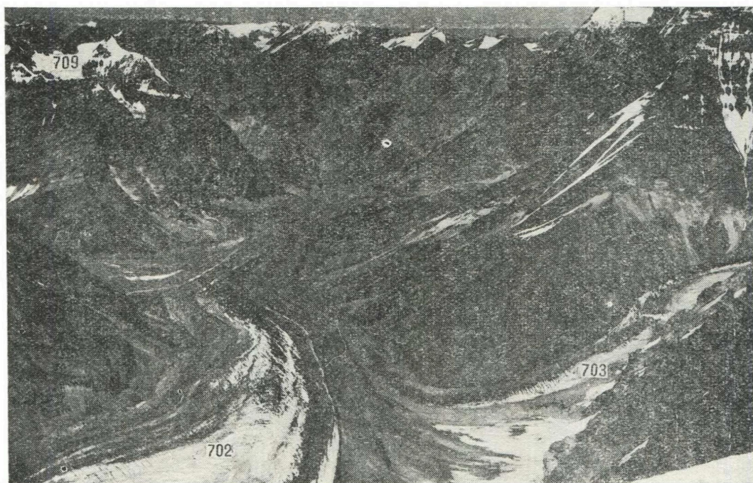
Рис. 40. Средняя и нижняя части ледника Аюджилга (№ 702). Фото В. А. Рудакова и Л. В. Десинова.
