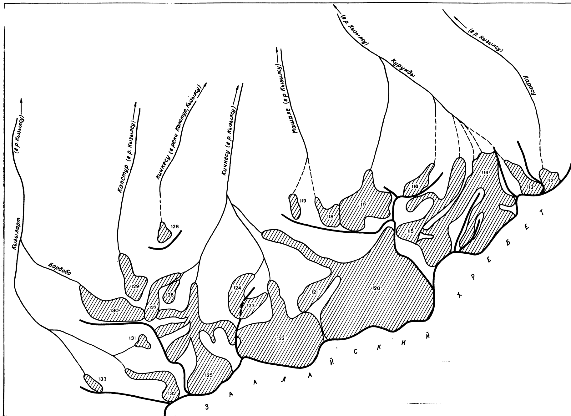
Рис. 23. Схема расположения ледников в бассейнах рек Карасу, Курумды, Машале, Кичкесу, Капстур и Кызыларт.
