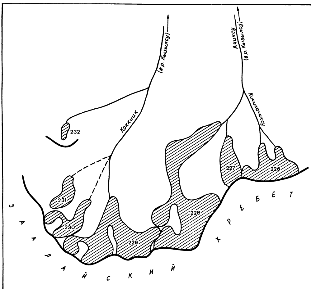
Рис. 27. Схема расположения ледников в бассейнах рек Ачиксу и Коккик. Усл. обозначения см. на рис. 17.
