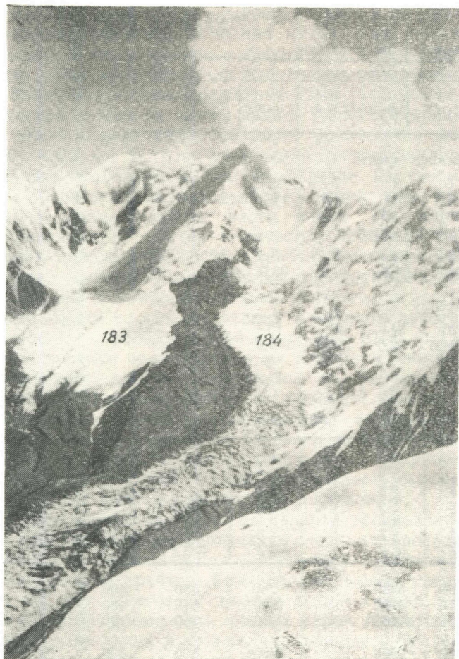
Рис. 3. Долинный ледник № 184 в хр. Ледяной мыс (бассейн р. Туюксу). Фото В. И. Рацка.
