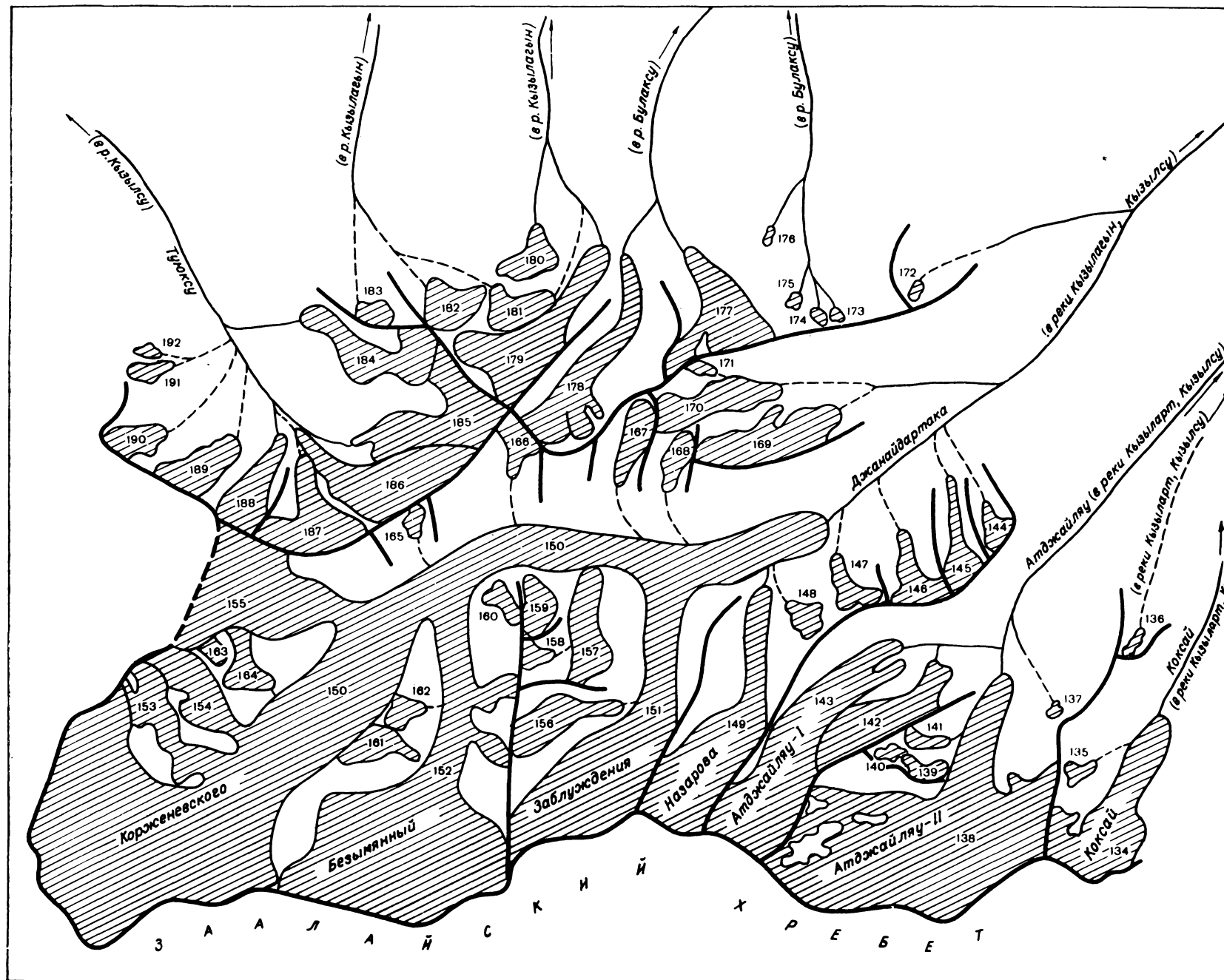
Рис. 24. Схема расположения ледников в бассейнах рек Коксай, Аtdжайлыу, Джанайдартака, Кызылагын и Туюксу.
