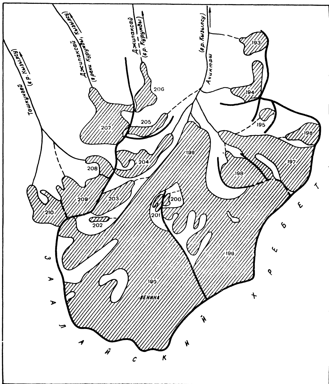
Рис. 25. Схема расположения ледников в бассейнах рек Ачикташ, Дзипаксай, Ташкунгей. Усл. обозначения см на рис. 17.
