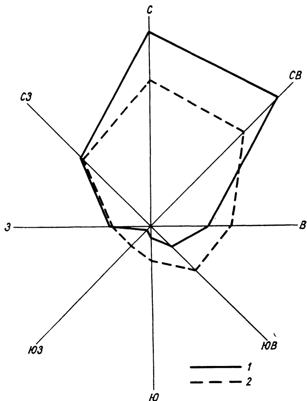
Рис. 7. Распределение ледников бассейна р. Кызылсу по экспозициям. 1 — количество ледников, 2 — площадь ледников.
