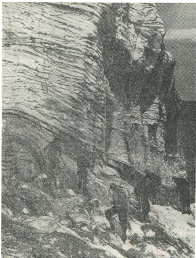
Рис. 12. Краевая часть ледника Корженевского. Фото В. И. Рацека.
