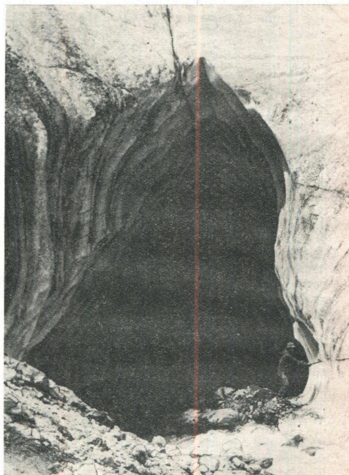
Рис. 8. Ледяной грот на леднике Корженевского (№ 150). Фото В. И. Рацка.
