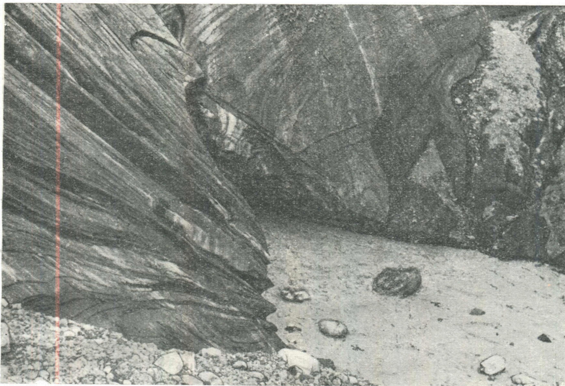
Рис. 9. Истоки р. Джанайдартака, берущей начало из ледника Корженевского. Фото В. И. Рацека.
