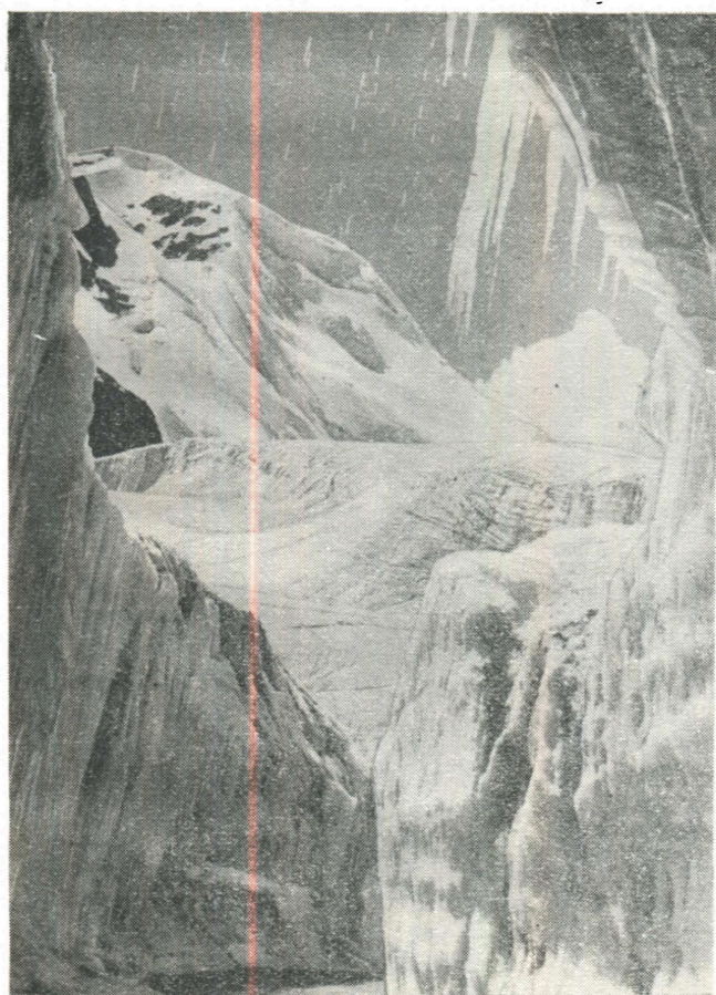
Рис. 10. Промоина на поверхности ледника Корженевского. Фото В. И. Рацека.
