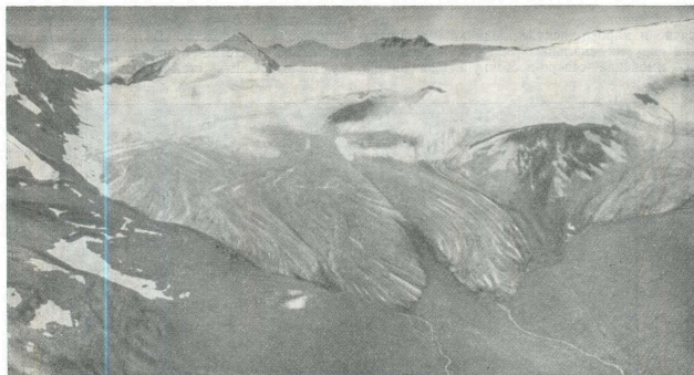
Рис. 26. Склоновый ледник № 270.
