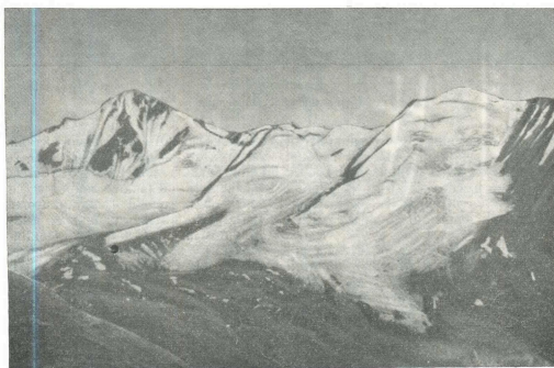
Рис. 27. Склоновый ледник № 480.
