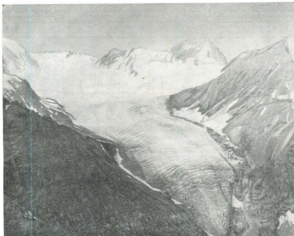
Рис. 13. Долинный ледник № 48.
