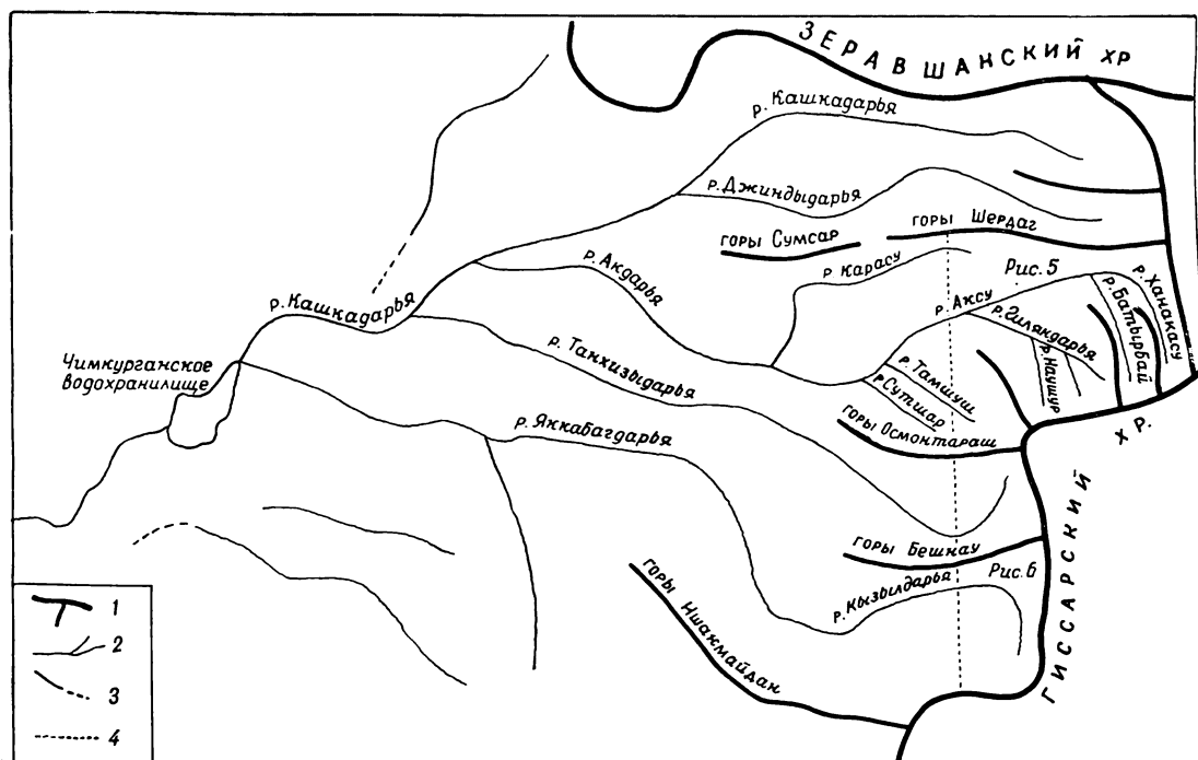
Рис. 4. Орогидрографическая схема бассейна р. Кашкадарья.
