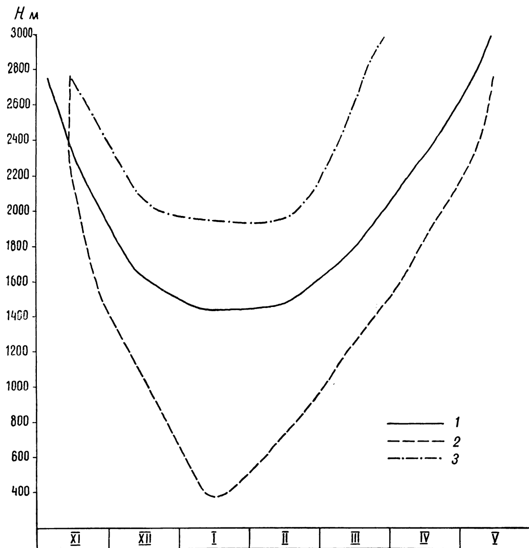
Рис. 3. Средняя многолетняя и экстремальная высота сезонной снеговой границы в бассейне р. Кашкадарья.
