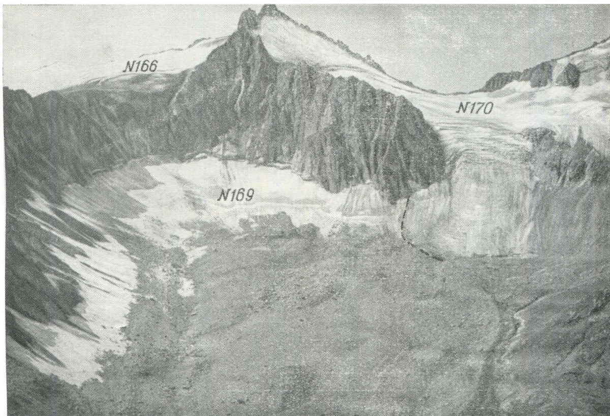
Рис. 19. Фирновая область ледника Дiahандара-1 и язык ледника Дiahандара-2. Фото А. С. Щетинникова.
