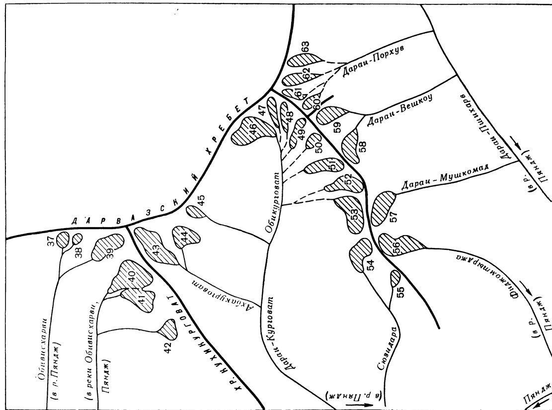
Рис. 9. Схема расположения ледников в бассейнах рек Обивисхари, Даран-Курговат, Филджомтырдж и Даран-Пшихарь. Усл. обозначения см. на рис. 6.
