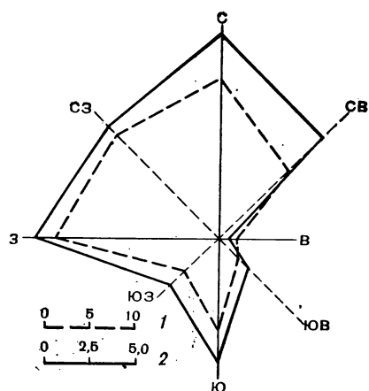
Рис. 3. Распределение ледников по экспозициям. 1 — количество, 2 — площадь, км 2 .
