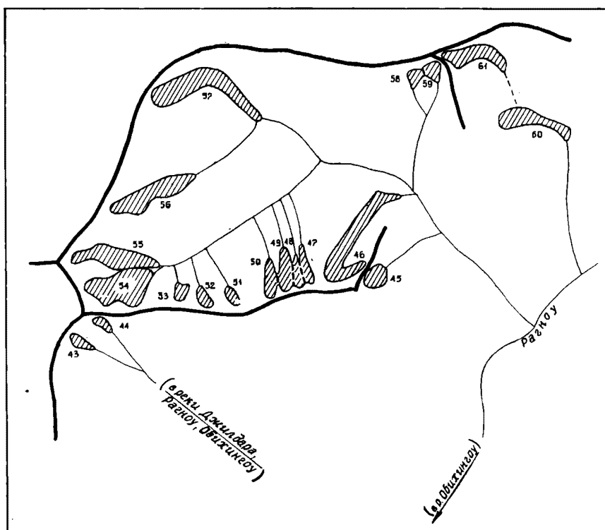
Рис. 26. Схема расположения ледников в бассейнах правых нижних притоков р. Рагноу. Уст. обозначения см. на рис. 25.
