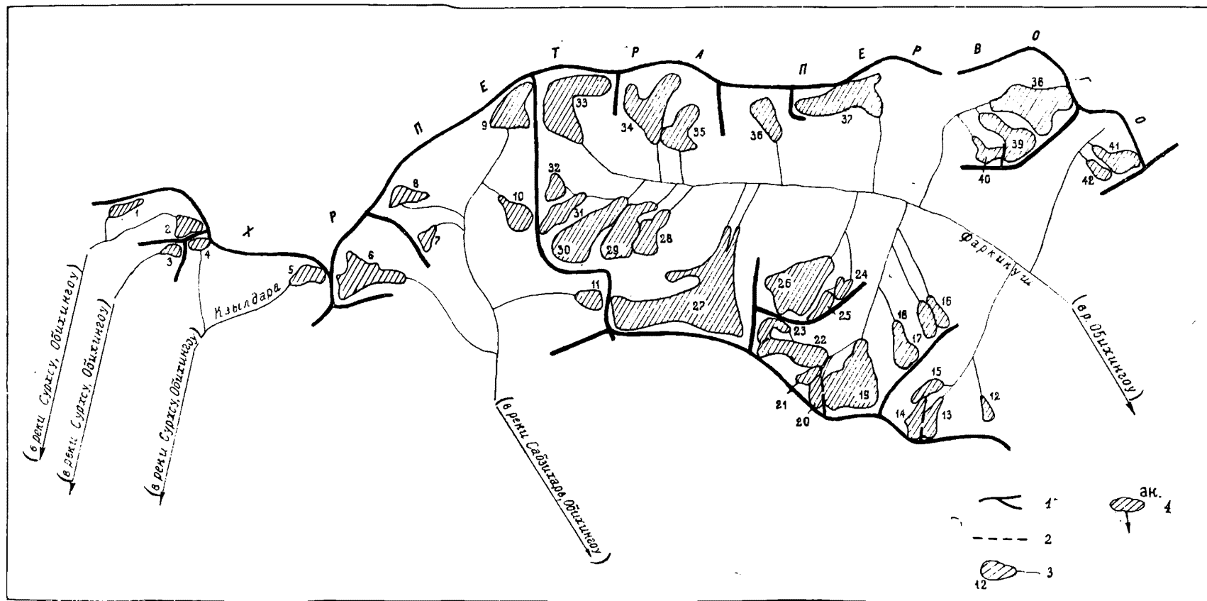
Рис. 25. Схема расположения ледников в бассейнах правых нижних притоков р. Обихингоу.
