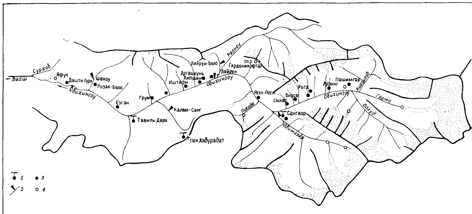
Рис. 45. Схема расположения гидрометеорологических станций и суммарных осадкомеров в районе ледников.
