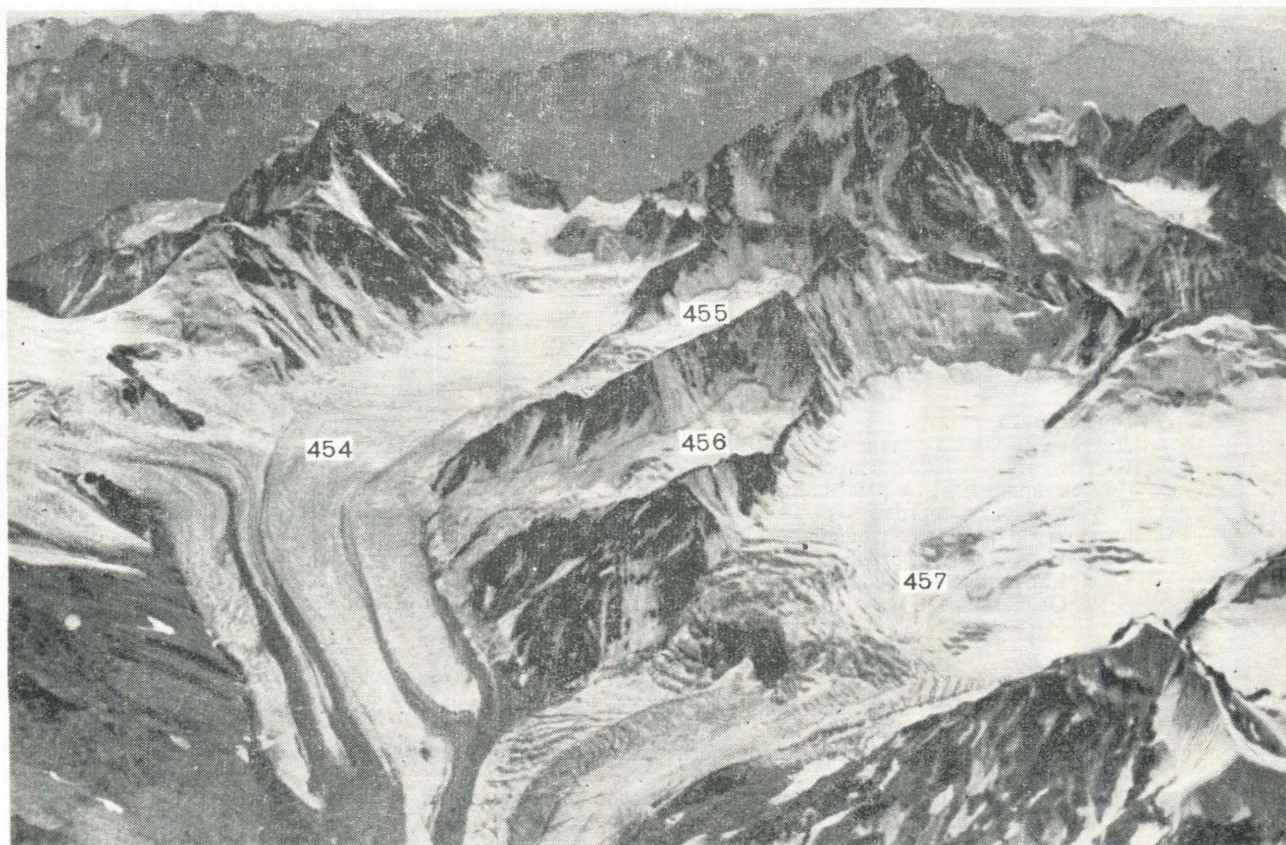
Рис. 58. Сложный долинный ледник (№ 452—457) в истоках р. Дархарвак.
