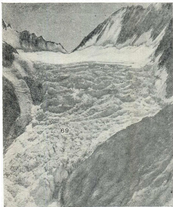
Рис. 13. Ледопад в верховьях ледника Петра Первого (№ 69).
