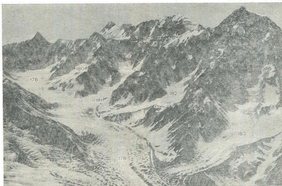
Рис. 16. Ледник Девлохан (№ 178) с притоками.
