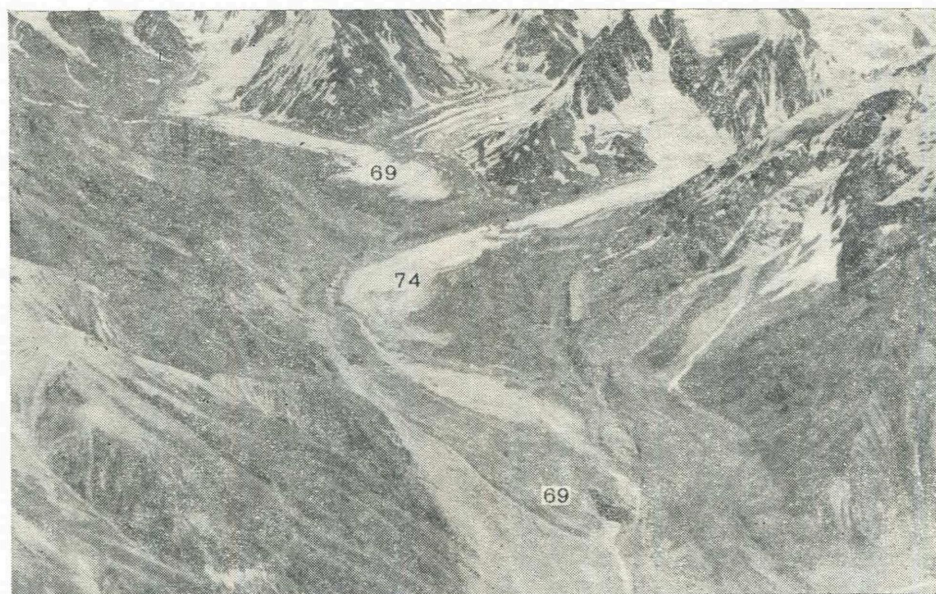
Рис. 15. Конец языка ледника Петра Первого (№ 69).
