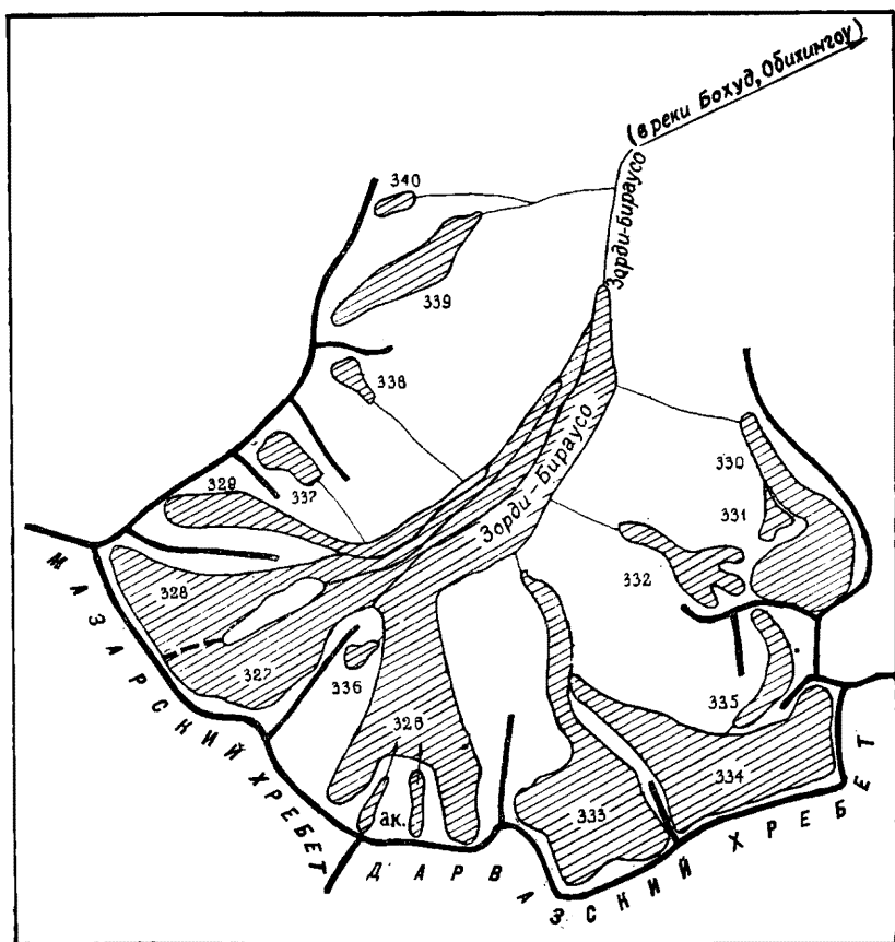
Рис. 35. Схема расположения ледников в бассейне р. Зорди-Бираусо.
