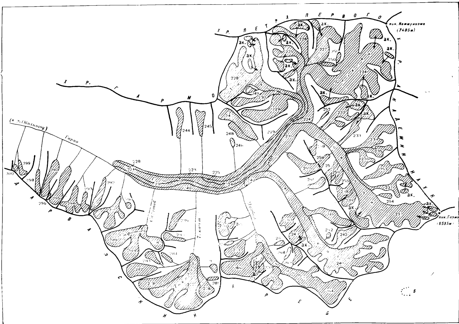
Рис. 33. Схема расположения ледников в бассейне р. Гармо.
