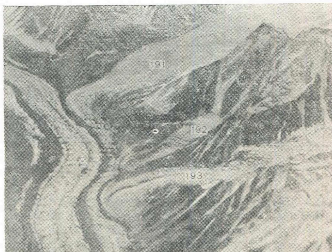
Рис. 12. Левые притоки ледника Гандо.
