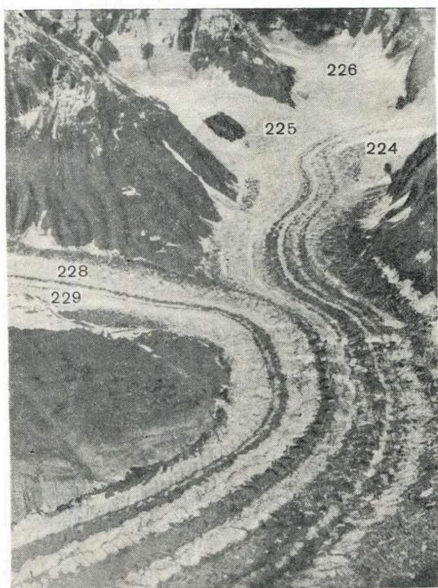
Рис. 50. Ледник Гармо. Участок слияния ледников Беляева (№ 224—227) и Липского (№ 228—230).
