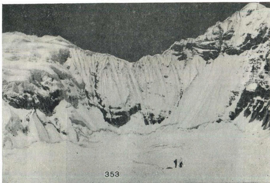
Рис. 52. Типичный участок фирновой области ледника Скогач (№ 353).
