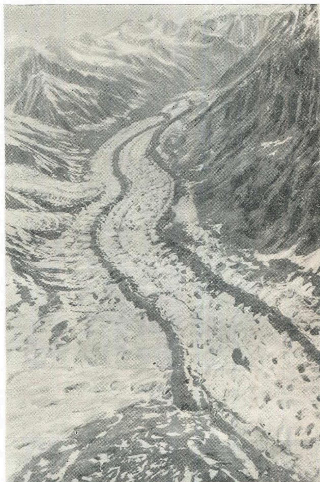
Рис. 11. Язык ледника Гандо.
