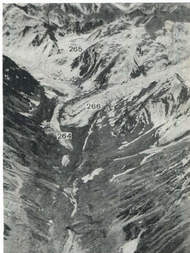
Рис. 51. Ледник Ванчара (№ 264—266) в бассейне ледника Гармо.
