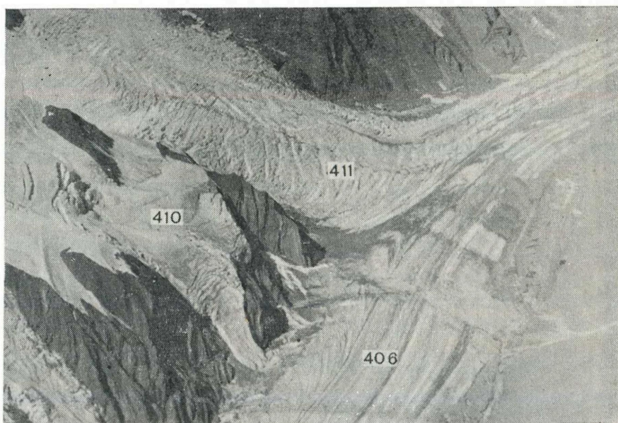
Рис. 55. Участок слияния Дарвазского ледника (№ 406) с его левым притоком № 411.
