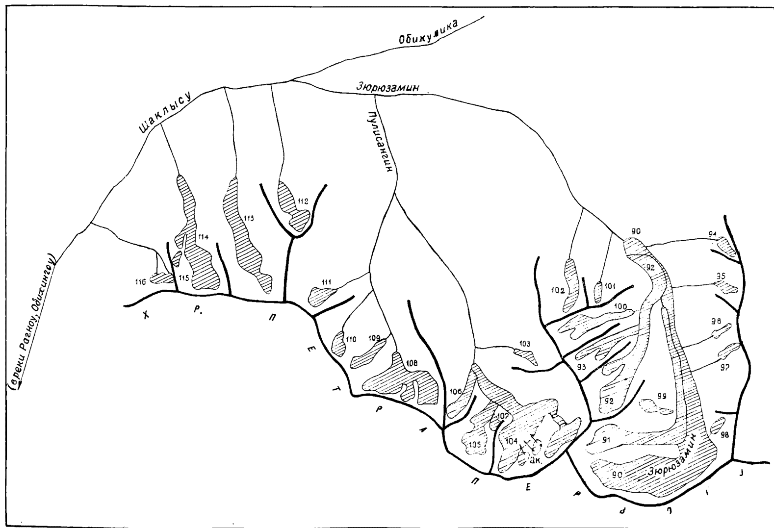
Рис. 28. Схема расположения ледников в бассейне р. Шаклысу.
