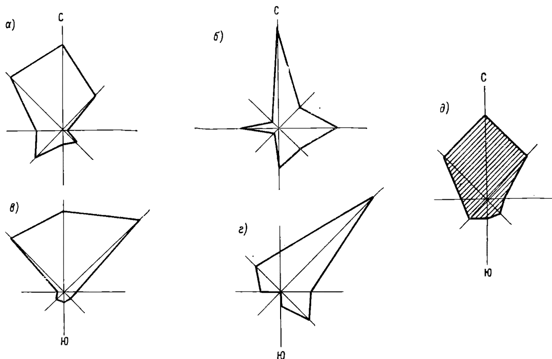
Рис. 7. Распределение площади ледников по экспозициям по основным районам бассейна р. Обихингоу.
