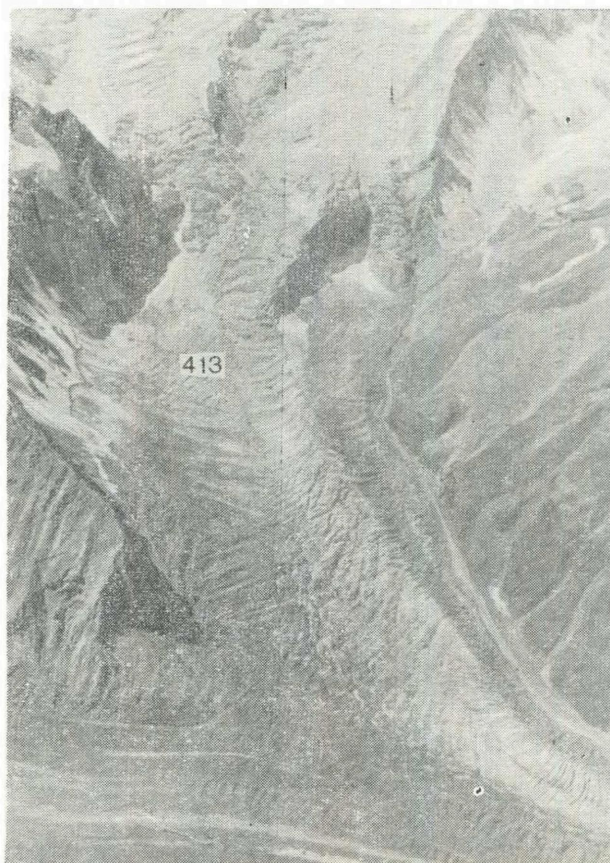
Рис. 56. Левый приток Дарвазского ледника (№ 413).
