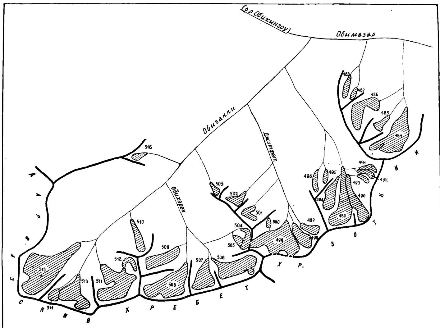
Рис. 43. Схема расположения ледников в бассейнах р. Обизанки и левых притоков р. Обмазар.
