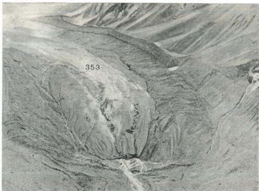
Рис. 54. Конец языка ледника Скогач (№ 353).
