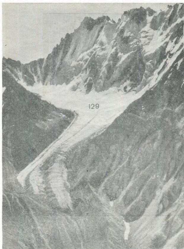
Рис. 46. Ледник Пир-Ях (№ 129), хр. Петра Первого.
