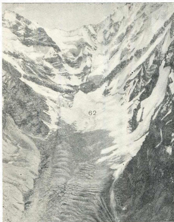
Рис. 19. Верховья ледника Баральмас (№ 62).
