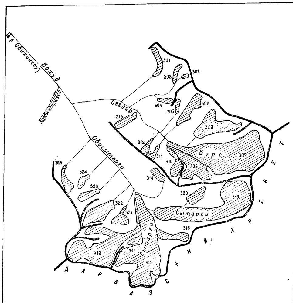
Рис. 34. Схема расположения ледников в бассейнах рек Сагдар и Обисыртарги.
