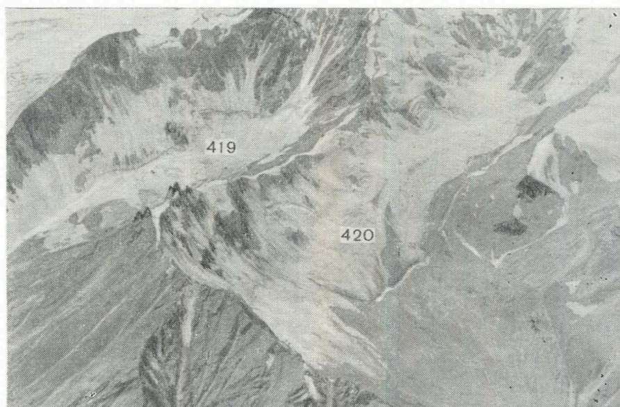
Рис. 57. Асимметричные долинные ледники № 419, 420 в бассейне Дарвазского ледника.
