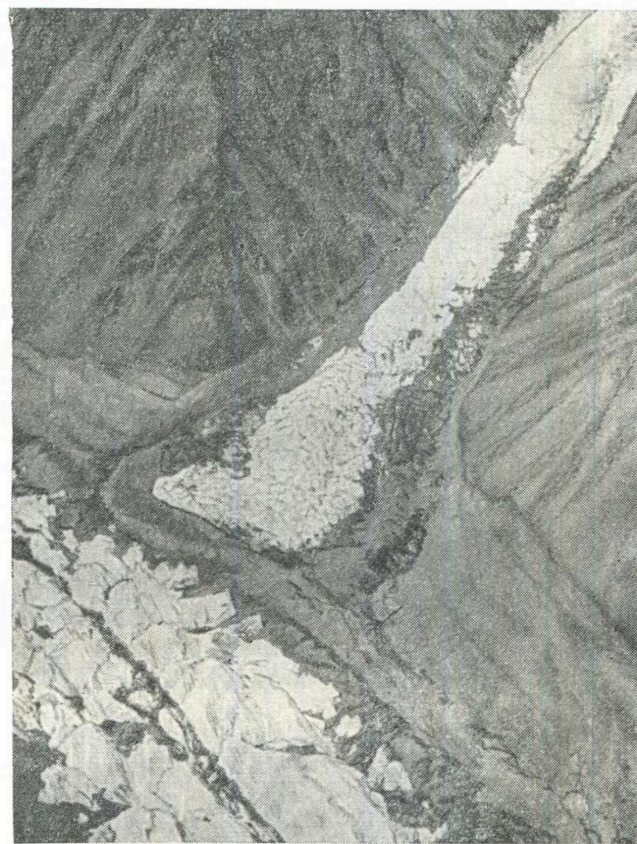
Рис. 23. Конец ледника № 285 (левого притока ледника Октябрьского).
