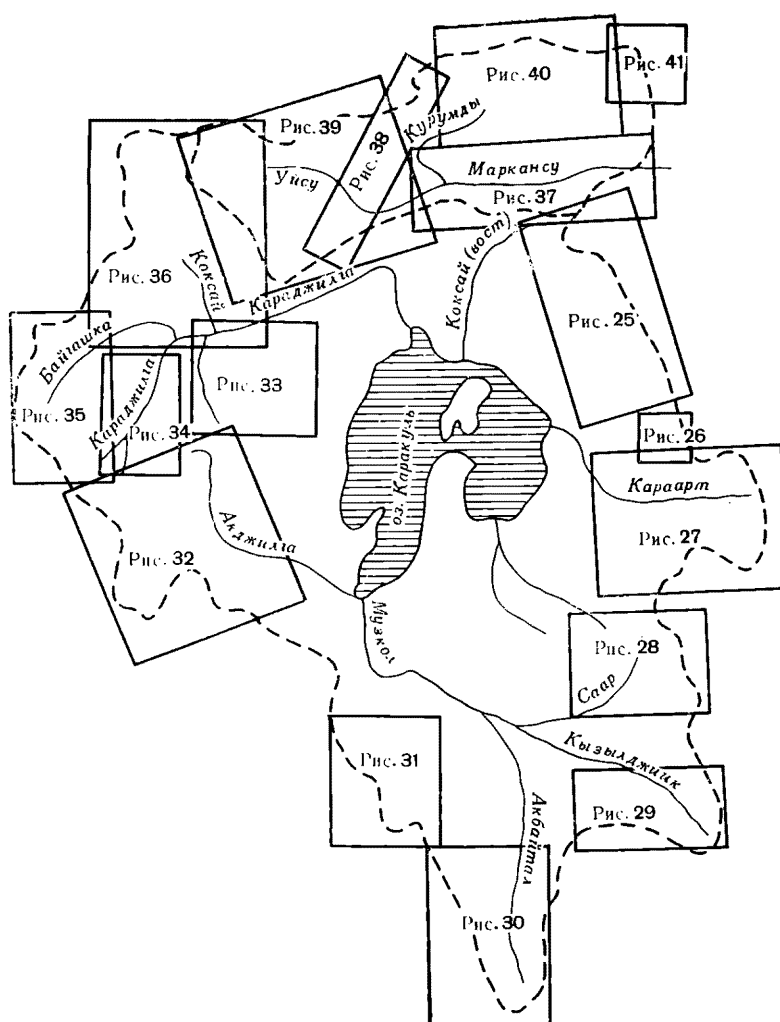
Рис. 24. Общая схема расположения бассейнов, в пределах которых размещаются ледники, показанные на рис. 25—41.
