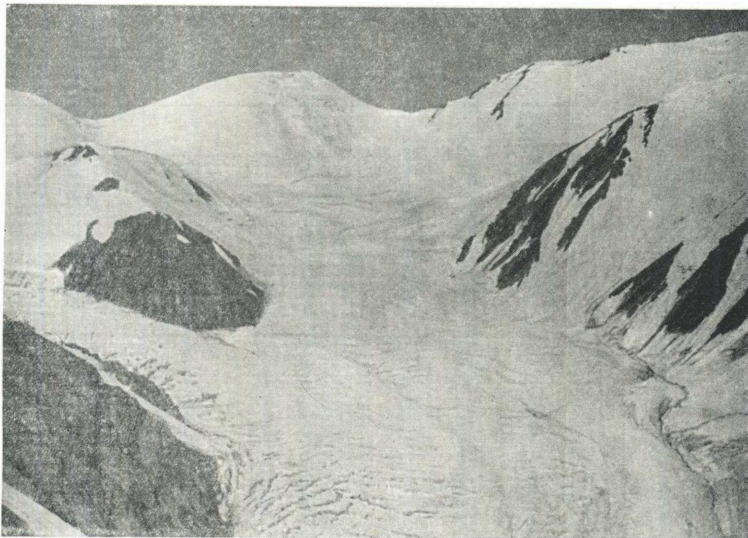
Рис. 10 Верховья основного потока ледника Октябрьского (№ 275).
