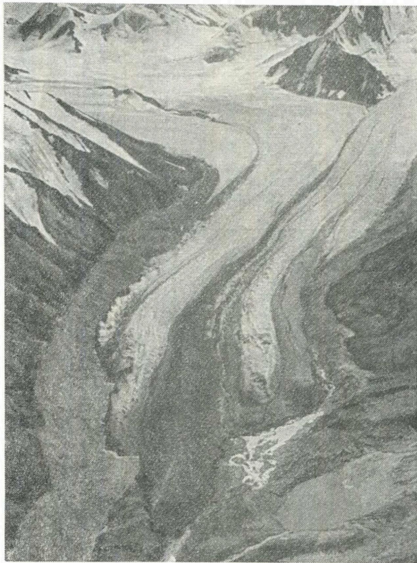
Рис. 22. Язык ледника Володарского (№ 243—245). Справа — озеро у конца ледника № 54.
