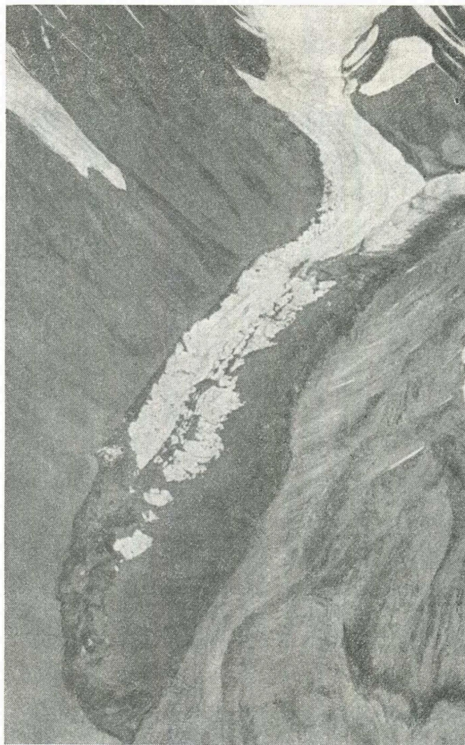
Рис. 46. Язык сложного долинного ледника № 294—296 в бассейне ледника Октябрьского.
