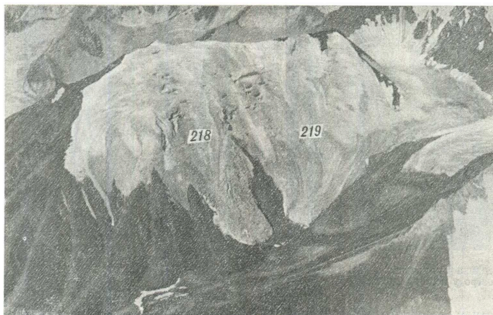
Рис. 20. Склоновые ледники № 218, 219 на левом склоне бассейна р. Караджилга.
