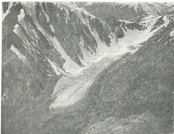
Рис. 18. Долинный ледник № 268 с преимущественно лавинным питанием.
