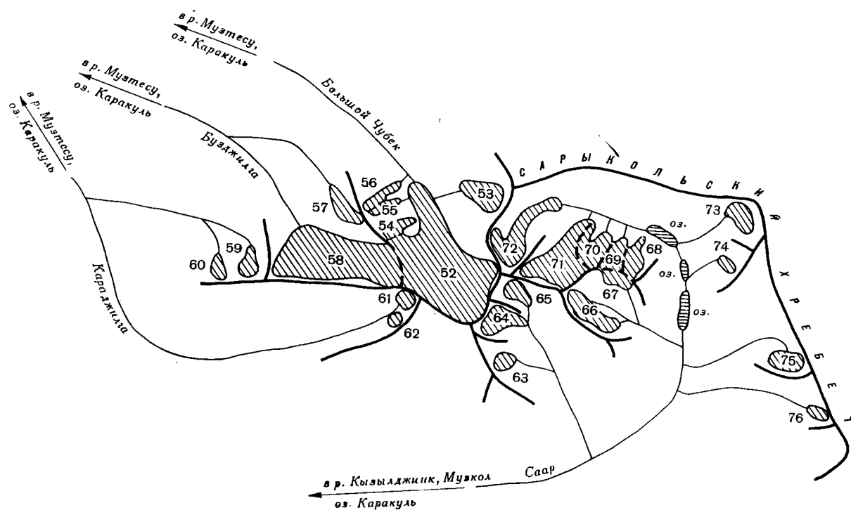
Рис. 28. Схема расположения ледников в бассейнах рек Муатесу и Саар. Усл. обозначения см. на рис. 25.
