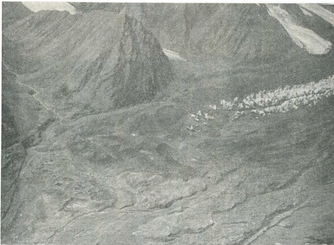
Рис. 45. Конец языка ледника Октябрьского.
