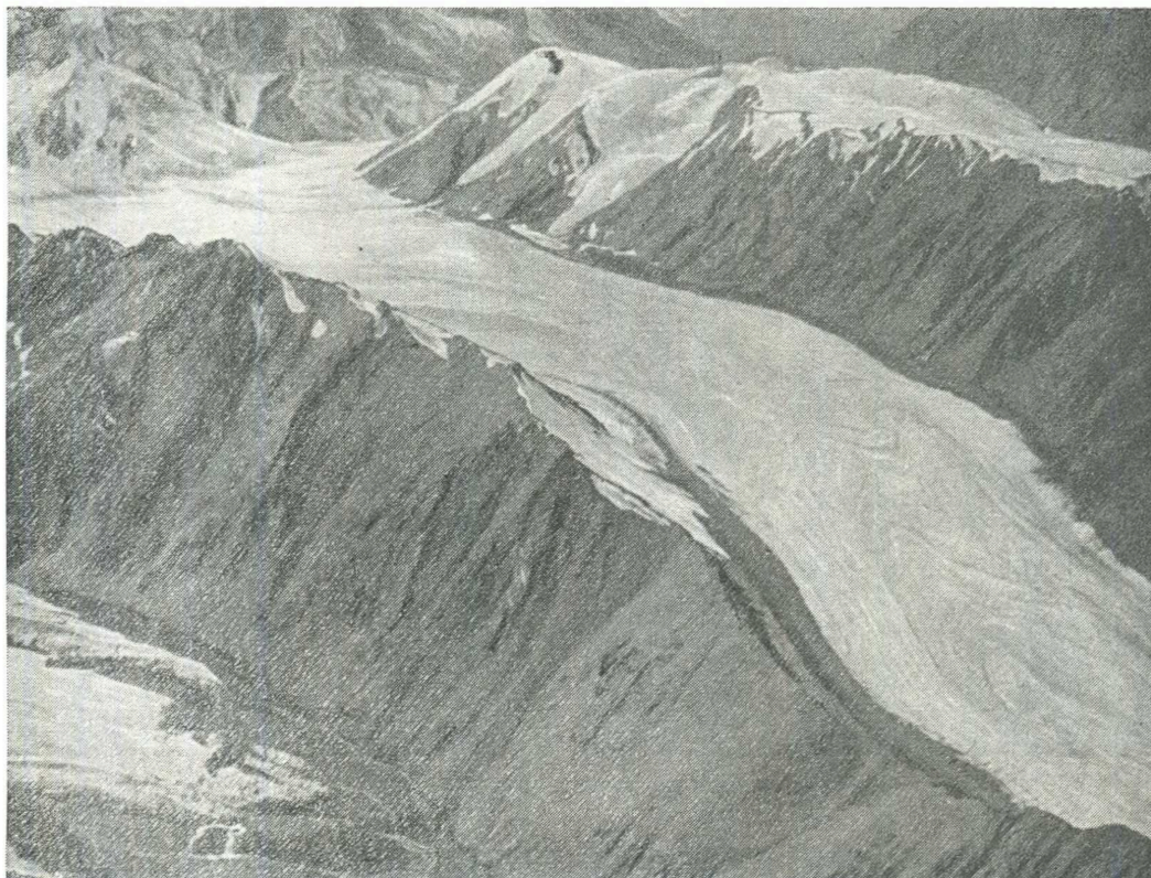
Рис. 12. Ледник Западный Октябрьский (№ 276) в среднем течении.
