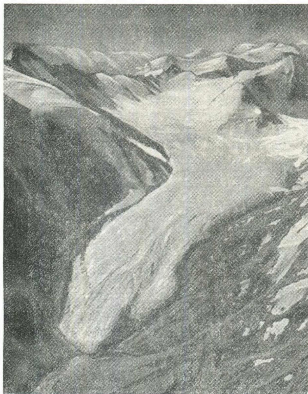
Рис. 16. Долинный ледник № 201 в верховье р. Караджилга.
