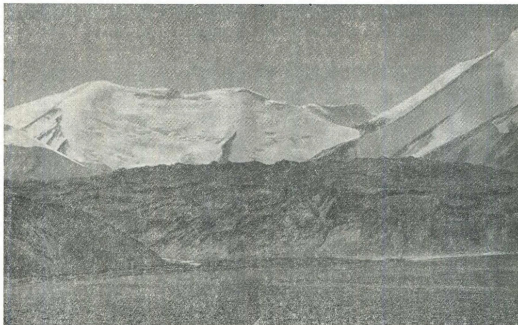
Рис. 15. Конец языка ледника Уйсу.
