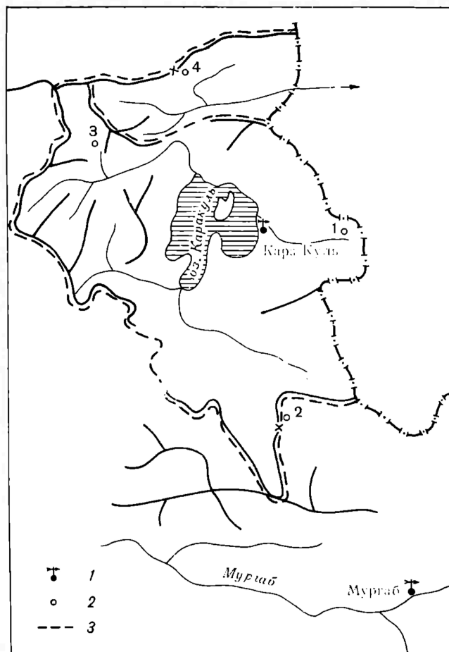
Рис. 42. Схема расположения гидрометеорологических станций и суммарных осадкомеров в районе ледников. 1 — действующие метеорологические станции, 2 — суммарные осадкомеры, 3 — границы бассейнов оз. Каракуль и р. Маркансу.
