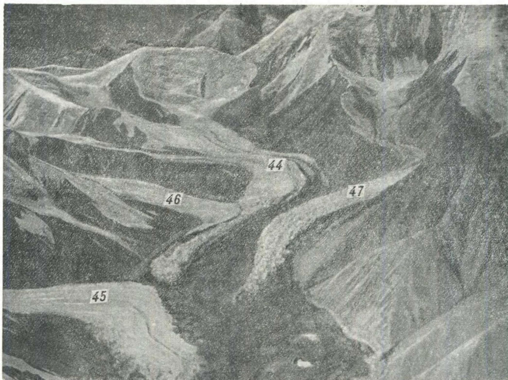
Рис. 14. Дендритовый ледник Уйсу.
