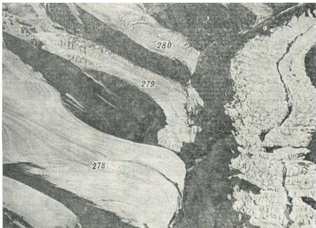
Рис. 11. Поверхность языка ледника Октябрьского (№ 275) в среднем его течении у впадения правых притоков (№ 278—280).
