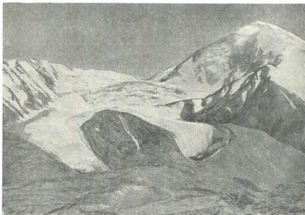
Рис. 49. Конец ледника № 42 в бассейне ледника Уйсу.
