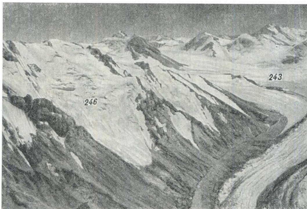
Рис. 7. Характер оледенения верховьев р. Байгашка (северный склон хр. Коммунаров) (ледники № 243, 246).
