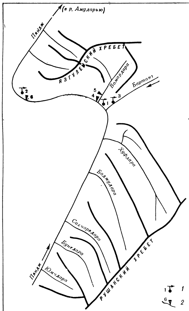
Рис. 22. Схема расположения гидрометеорологических станций и постов в районе ледников. 1 — метеорологическая станция и пост, 2 — гидрологический пост.
