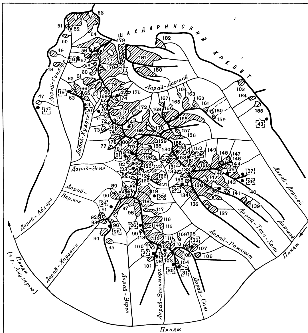
Рис. 11. Схема расположения ледников в бассейнах рек Дарай-Абхарь, Дарай-Харавык, Дарай-Зерев, Дарай-Завчмор, Дарай-Санг, Дарай-Романит, Дарай-Тока-Хана, Даршай и Дарай-Даршай. Усл. обозначения см. на рис. 10.
