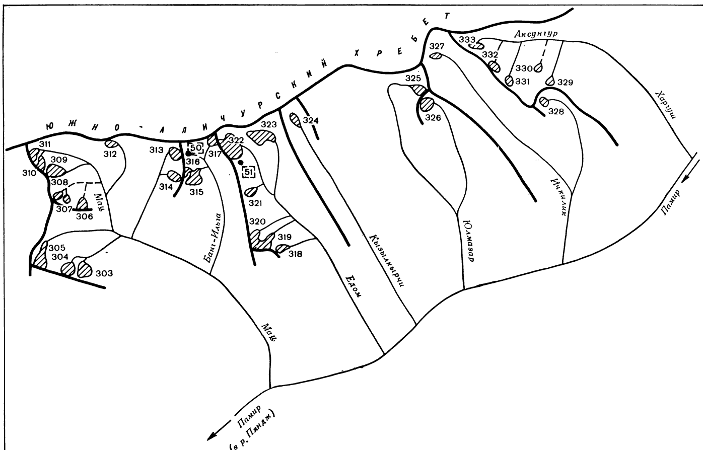
Рис. 14. Схема расположения ледников в бассейнах рек Мац, Едом, Кызылкырчи, Юлмазар, Тчкилик и Харгуш. Усл. обозначения см. на рис. 10.
