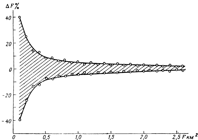
Рис. 1. Зависимость максимальной ошибки округления площади до 0,1 км² ( \Delta F\% ) от площади ледника F .
