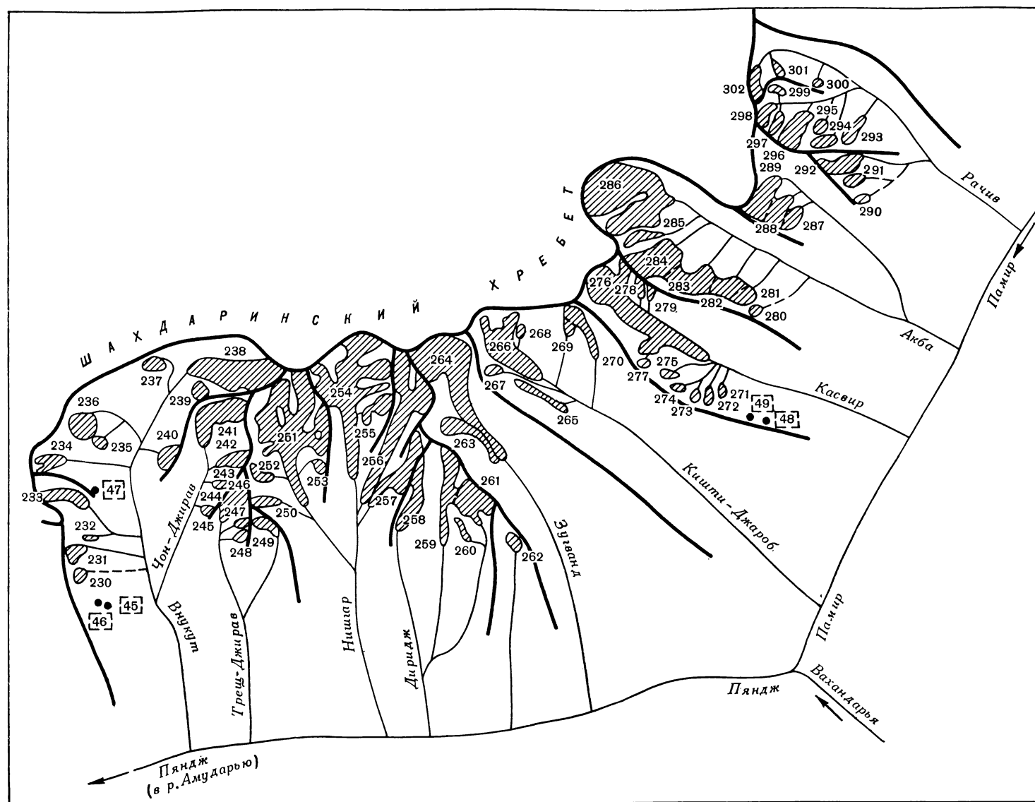
Рис. 13. Схема расположения ледников в бассейнах рек Вукут, Трещ-Джирав, Нишгар, Диридж, Зугванд, Кашти-Джароб, Касвир, Якба и Рачия. Усл. обозначения см. на рис. 10.
