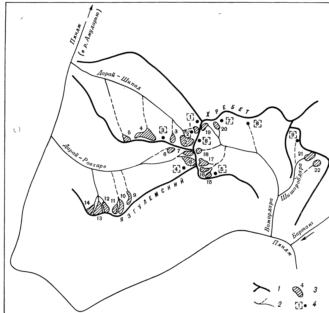
Рис. 20. Схема расположения ледников в бассейнах рек Дарай-Шипад, Дарай-Ровхарв и Вомар-дара. 1 — хребет, 2 — река, 3 — ледник и его порядковый номер по табл. 1, 4 — ледник размером менее 0,1 км² и его порядковый номер по табл. 39
