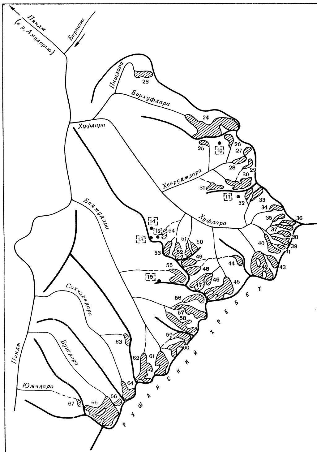
Рис. 21. Схема расположения ледников в бассейнах рек Худара, Баджудара, Сохчарвдара, Бунедара и Юмчдара. Усл. обозначения см. на рис. 20.
