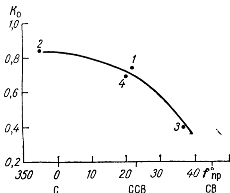
Рис. 6. Связь между коэффициентом ориентации K_0 и преобладающей ориентацией f_{пр} ледников бассейнов левых притоков Сарезского озера и р. Мургаба (1), верховьев рек Сулистый и Аксу (2), правых притоков р. Мургаба и Сарезского озера (3) и бассейна р. Мургаба в целом (4).
