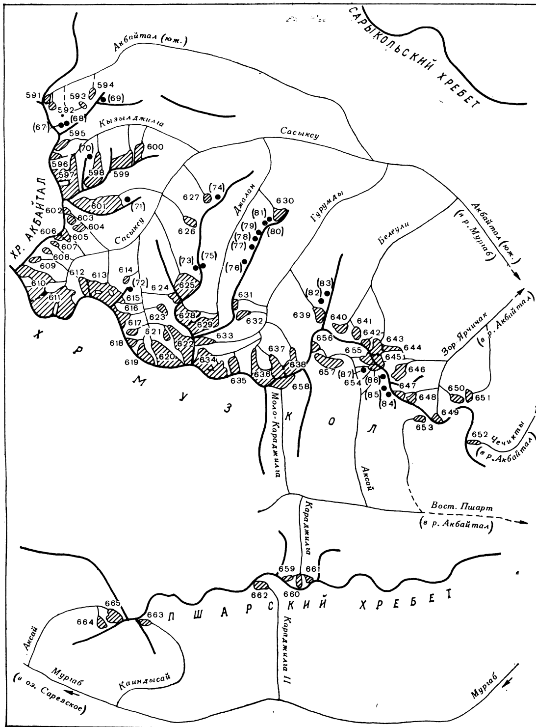
Рис. 17. Схема расположения ледников в бассейнах рек Акбайтал (юж.), Восточного Пшарта, Караджилга II, Каиндысай и Аксай.
