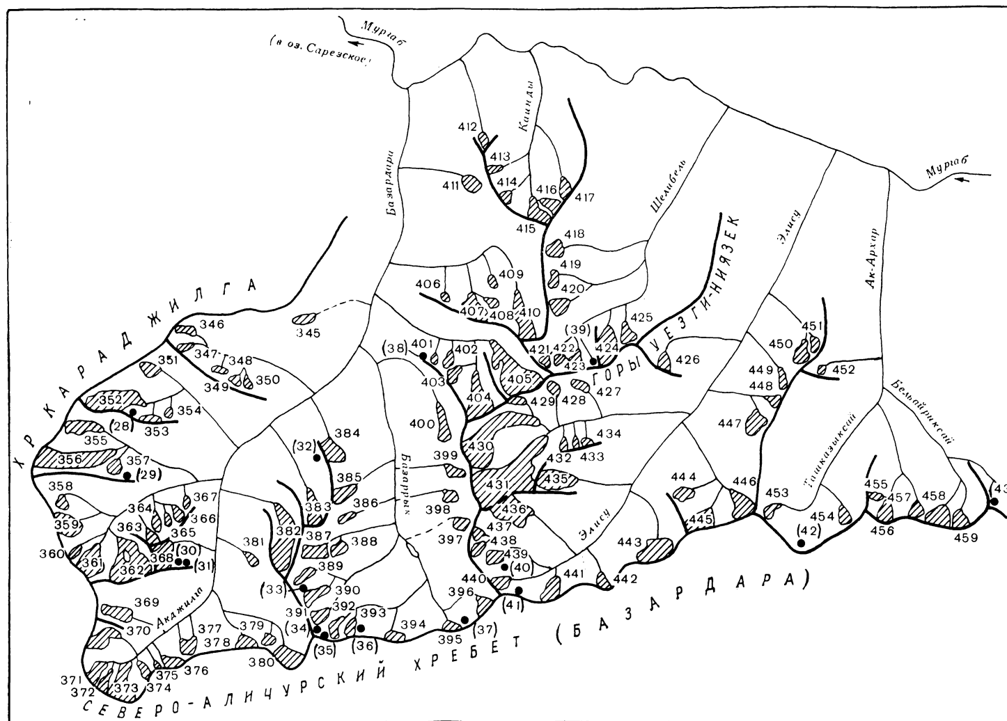
Рис. 12. Схема расположения ледников в бассейнах рек Базардара, Кайнды, Шелибель, Элису и Ак-Архар.
