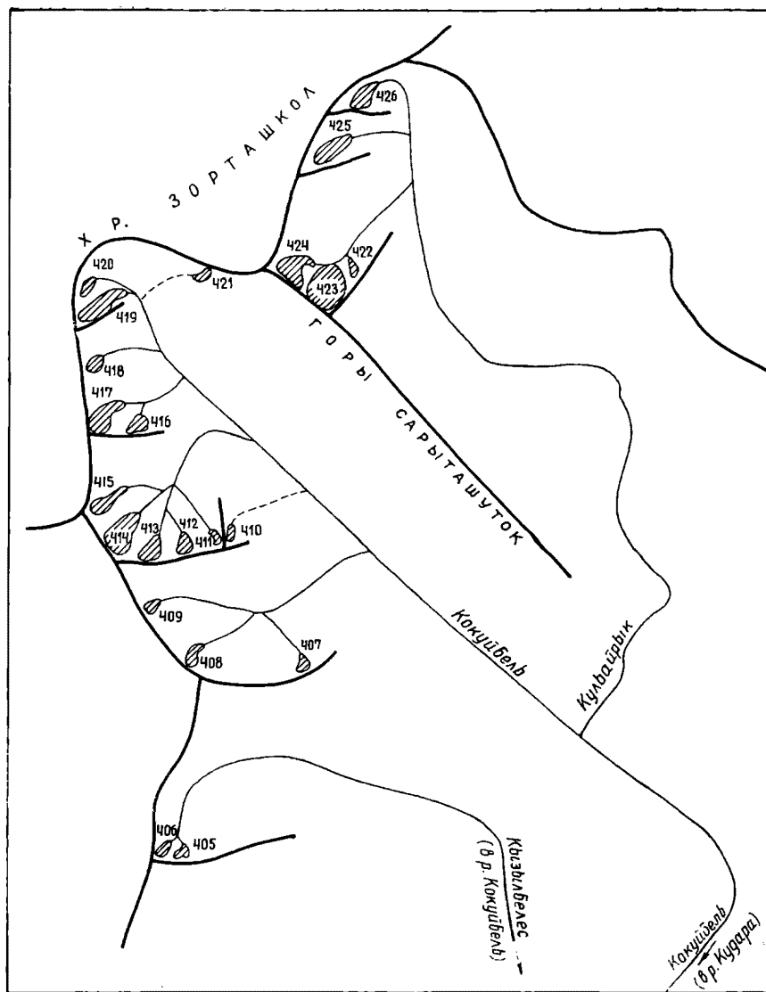
Рис. 23. Схема расположения ледников в верховьях рек Кызылбелес, Кокуйбель и Кулайрык. Усл. обозначения см. на рис. 11.
