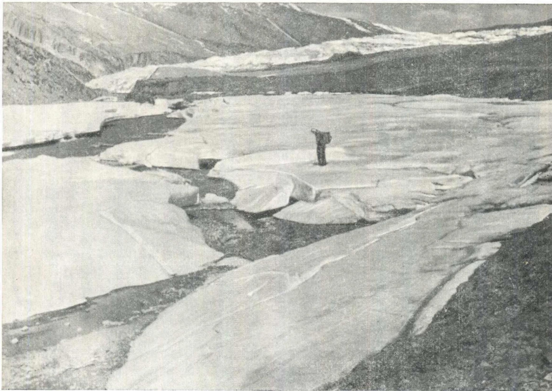
Рис. 44. Наледи в верховьях р. Танымас. Фото В. К. Ноздрюхина.
