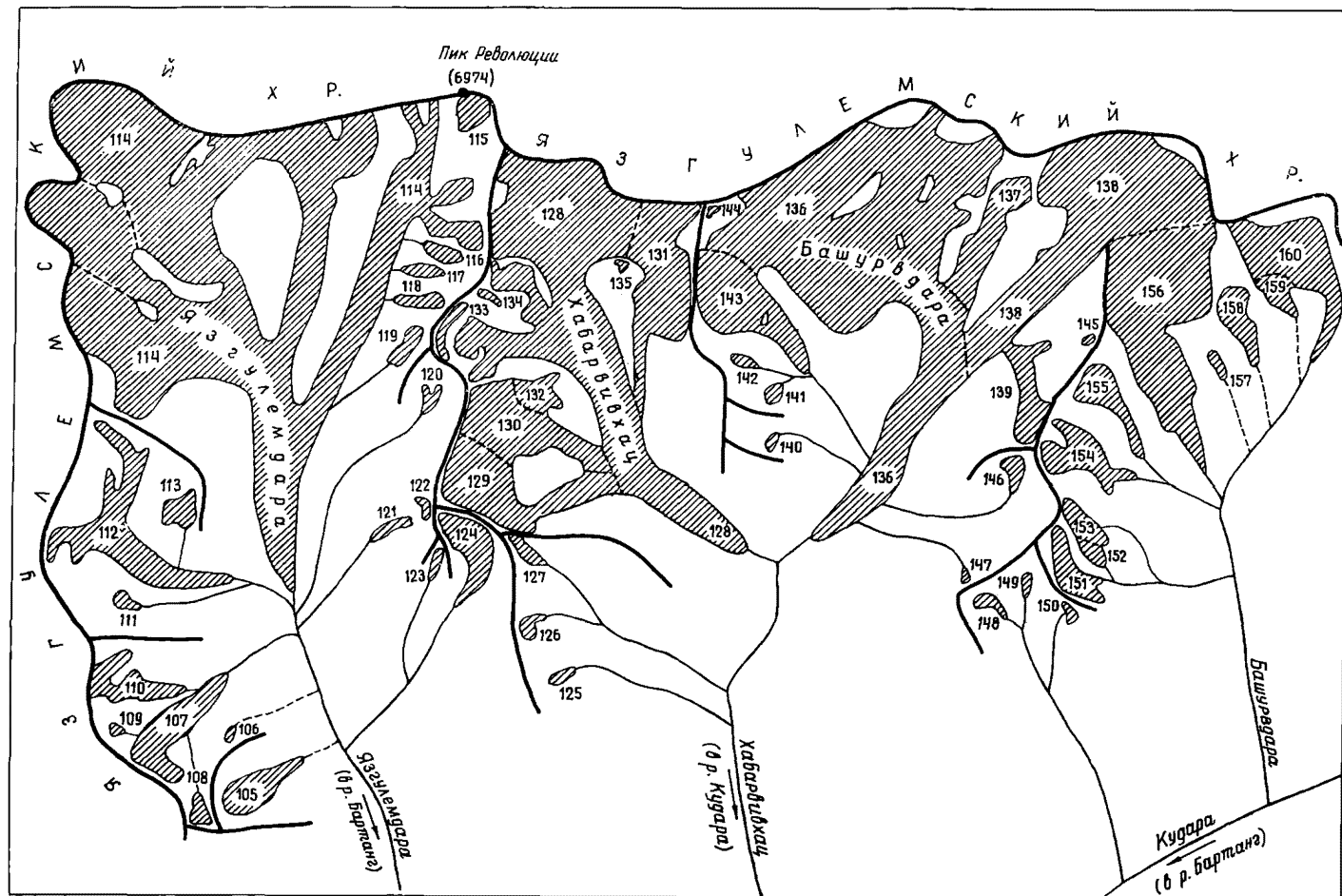
Рис. 15. Схема расположения ледников в верховьях рек Язгулемдара, Хабарвинха и Башурвдара. Усл. обозначения см. на рис. 11.
