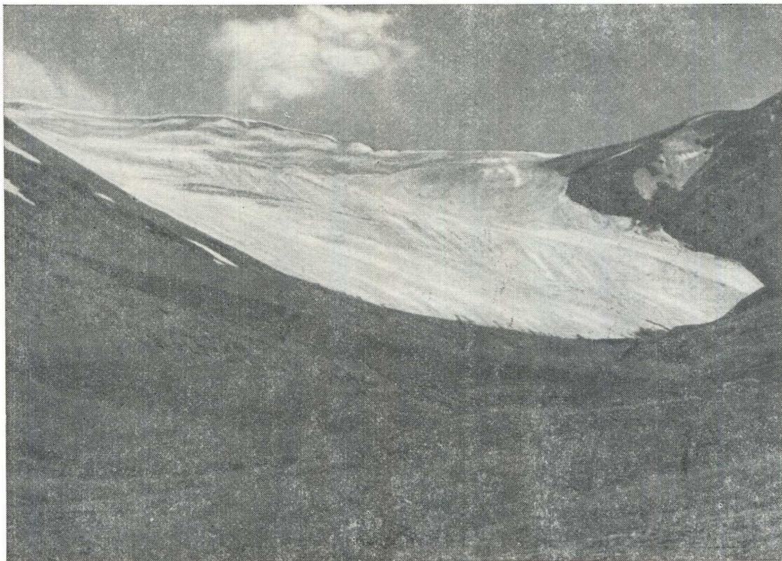
Рис. 39. Каровый ледник № 423 в бассейне р. Кульбайрык. Фото А. С. Щетинникова.
