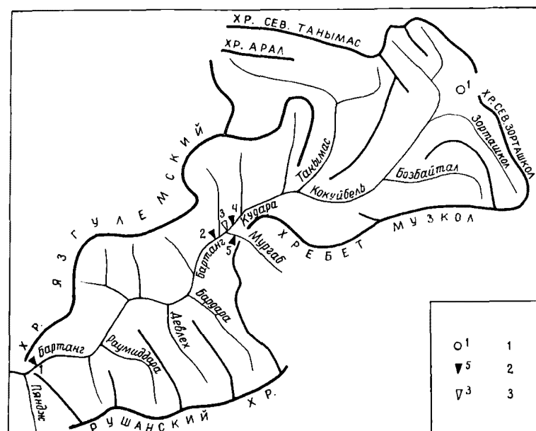
Рис. 35. Схема расположения гидрологических постов и суммарных осадкомеров.
