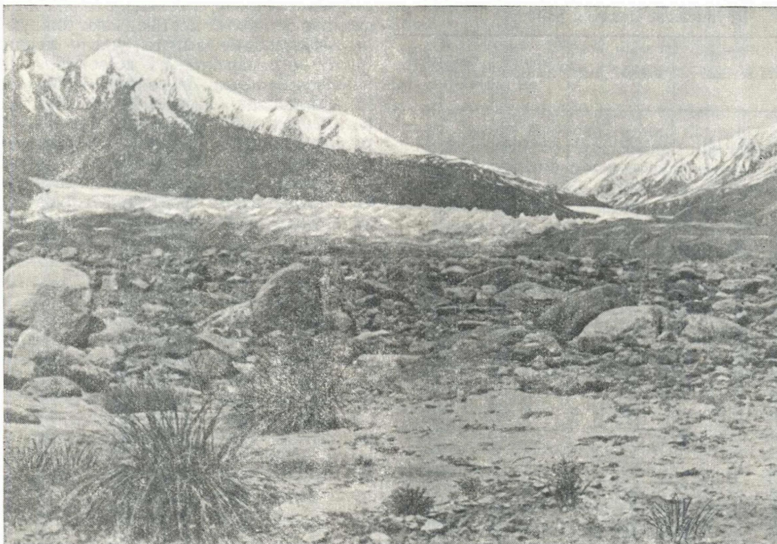
Рис. 5. Конец языка ледника Грумм-Гржимайло (№ 237). Фото В. Ф. Сулова.
