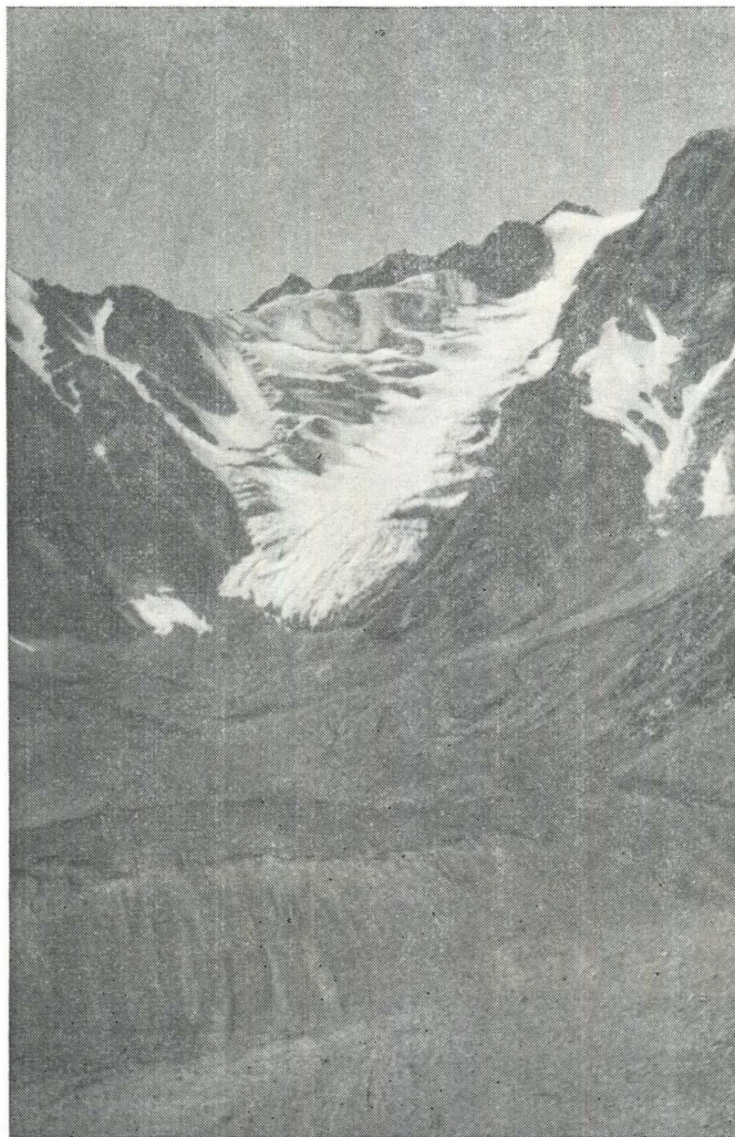
Рис. 41. Висячий ледник № 459 в бассейне р. Зорташкол. Фото А. С. Щетинникова
