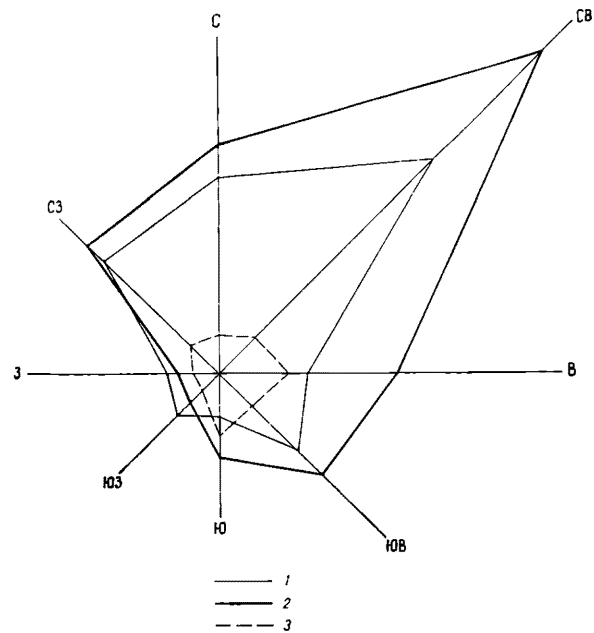
Рис. 7. Распределение числа (1), площади (2) и размеров среднего ледника (3) по экспозициям.
