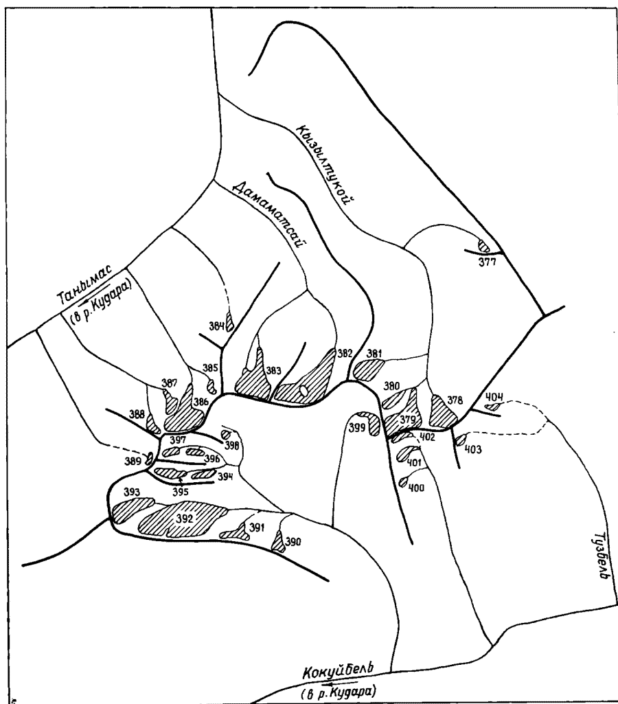
Рис. 22. Схема расположения ледников в бассейнах рек Кызылтукой, Дамаматсай, Тузбель и безымянных притоков рек Танымас и Кудара.
