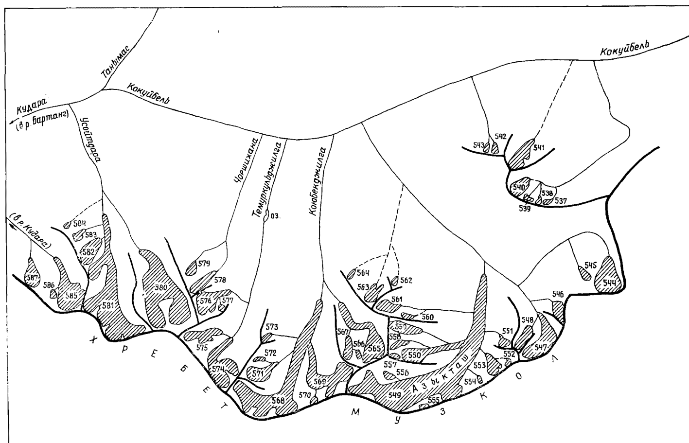
Рис. 27. Схема расположения ледников в бассейнах правых притоков рек Кокуйбелъ и Кудара. Усл. обозначения см. на рис. 11.
