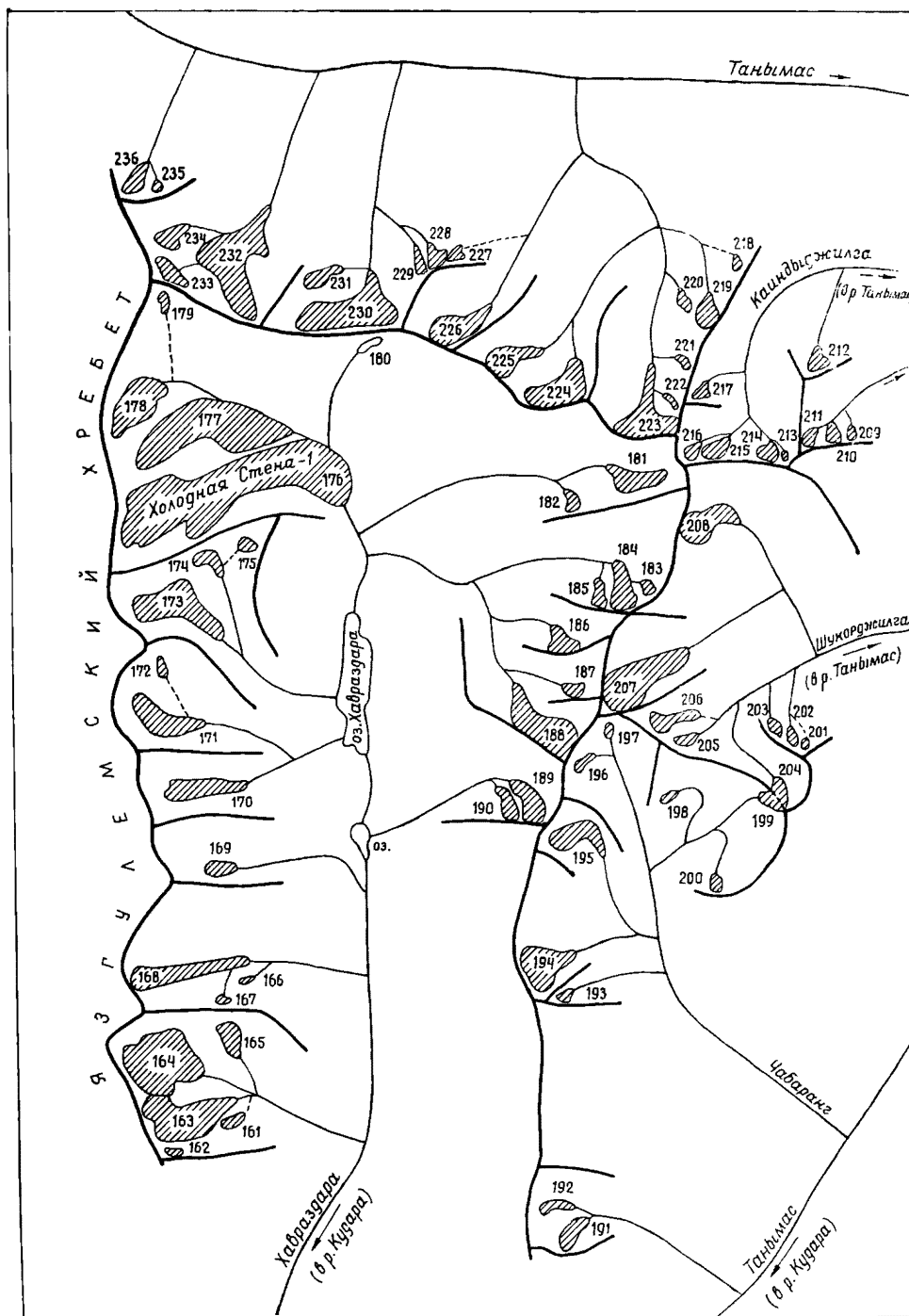
Рис. 16. Схема расположения ледников в бассейнах рек Хавраздара, Чабаранг, Шукорджилга, Кайндыжилга и правых безымянных притоков р. Танымас. Усл. обозначения см. на рис. 11.
