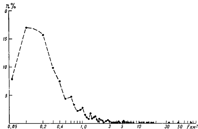
Рис. 4. Распределение числа ледников (n%) по величине их площади (F км 2 ).
