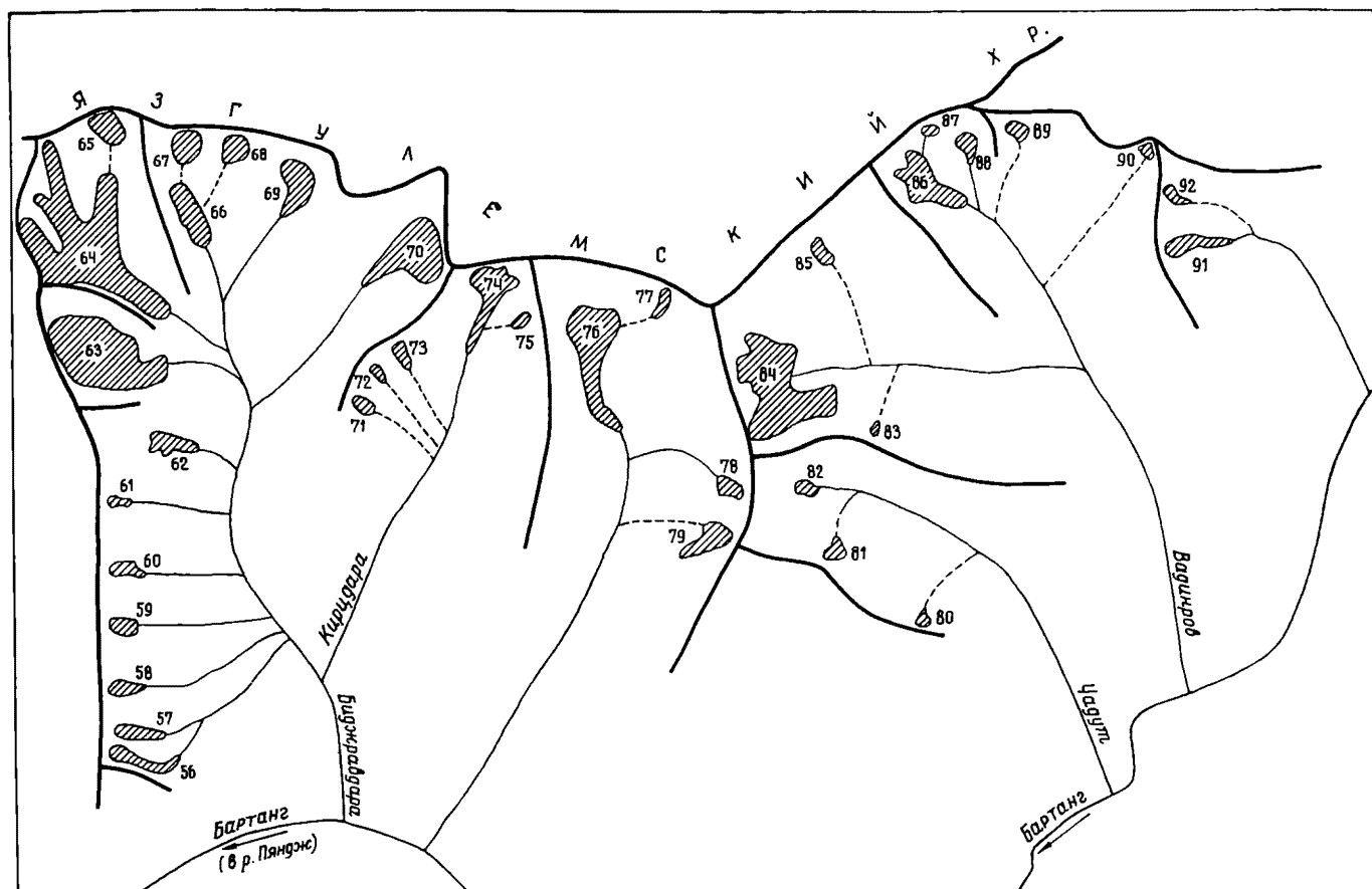
Рис. 13. Схема расположения ледников в бассейнах рек Биджравдара, Чадут, Вадинров и безымянных притоков р. Бартауга. Усл. обозначения см. на рис. 11.
