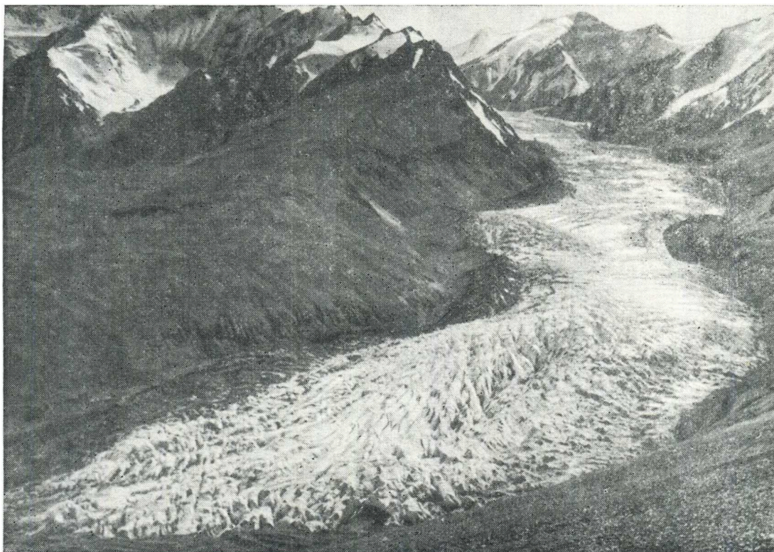
Рис. 37. Ледник Танымас-2 (№ 273). Фото В. И. Рацека.
