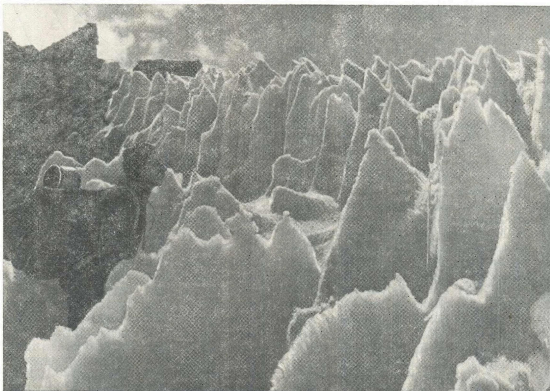
Рис. 6. Кальгаспоры на леднике Северный Танымас. Фото В. К. Ноздрюхина.
