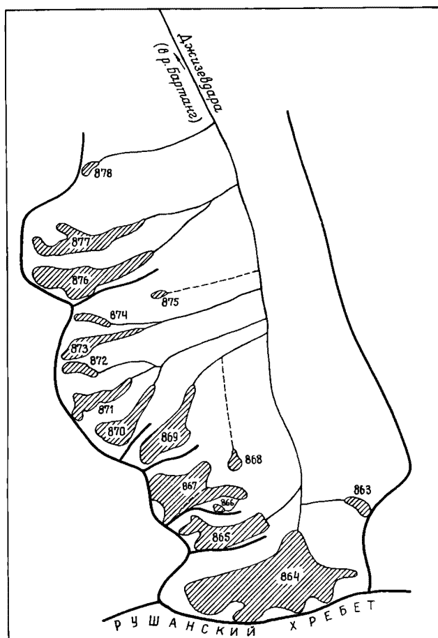
Рис. 33. Схема расположения ледников в бассейне р. Джизевдара. Усл. обозначения см. на рис. 11.
