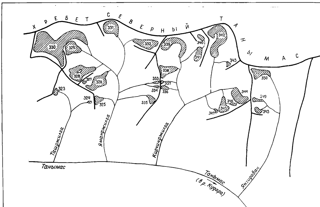
Рис. 20. Схема расположения ледников в бассейнах рек Ташджилга, Яманджилга, Кирчинджилга и Янгидаван. Усл. обозначения см. на рис. 11.
