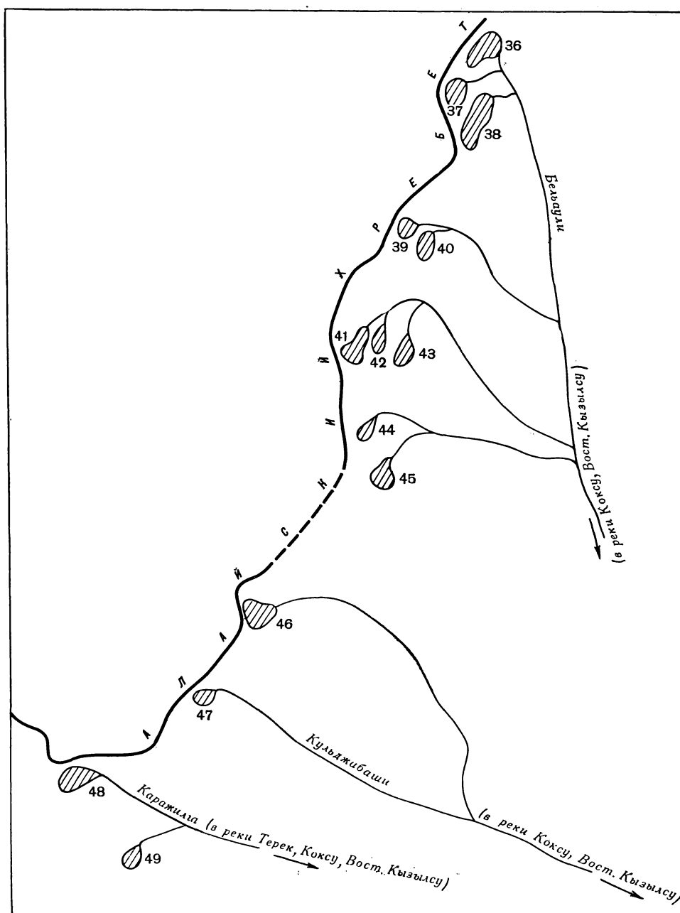
Рис. 15. Схема расположения ледников в бассейнах рек Бельяули, Кульджабаш, Каражилга. Усл. обозначения см. на рис. 6.
