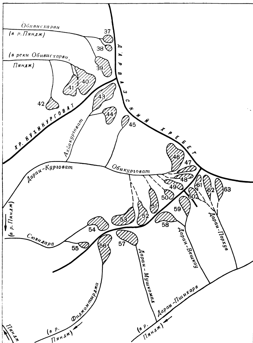
Рис. 9. Схема расположения ледников в бассейнах рек Обвиссарви, Дарай-Курговат, Фиджомтырджа и Дарай-Пшихарв. Усл. обозначения см. на рис. 6.
