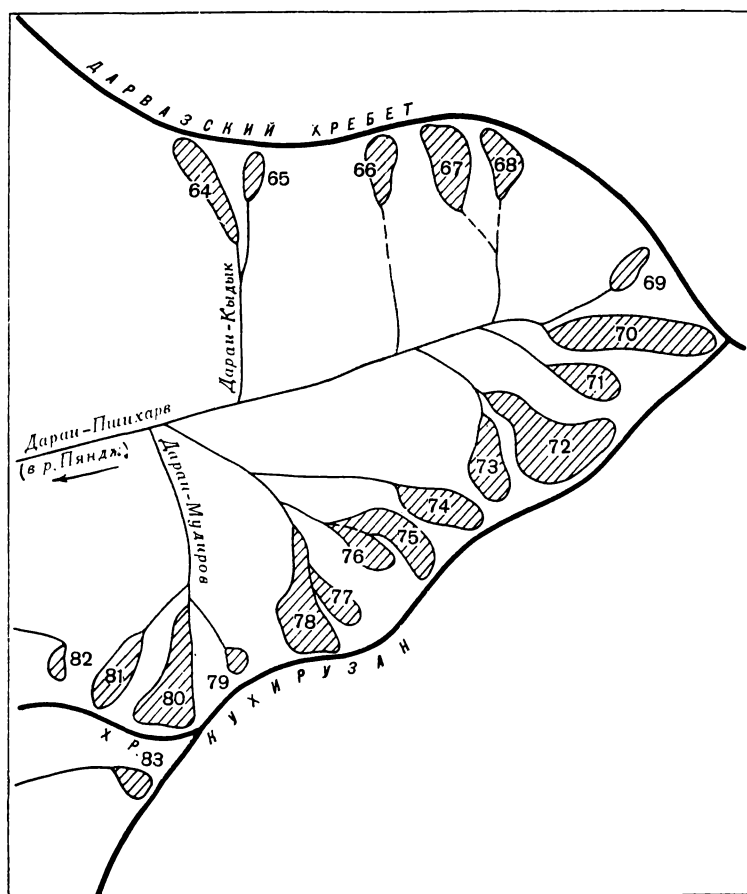
Рис. 10. Схема расположения ледников в бассейнах рек Даран-Пшихарв и Даран-Вурауз. Усл. обозначения см. на рис. 6.
