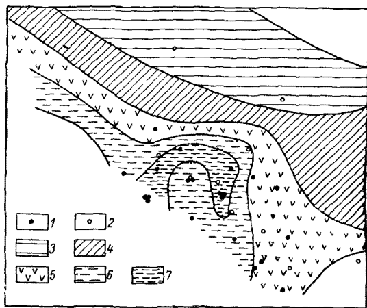
Рис 58. Схема снижения уровня подземных вод на участке водозабора Алтыябского конуса выноса
