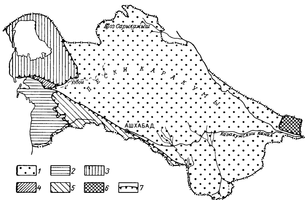
Рис. 16. Схема гидрогеологического районирования территории Туркменской ССР
