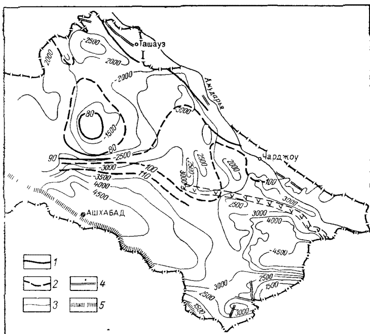
рис. 40. Схематическая карта геизотерм Каракумского артезианского бассейна по кровле водоносного комплекса юрских отложений
