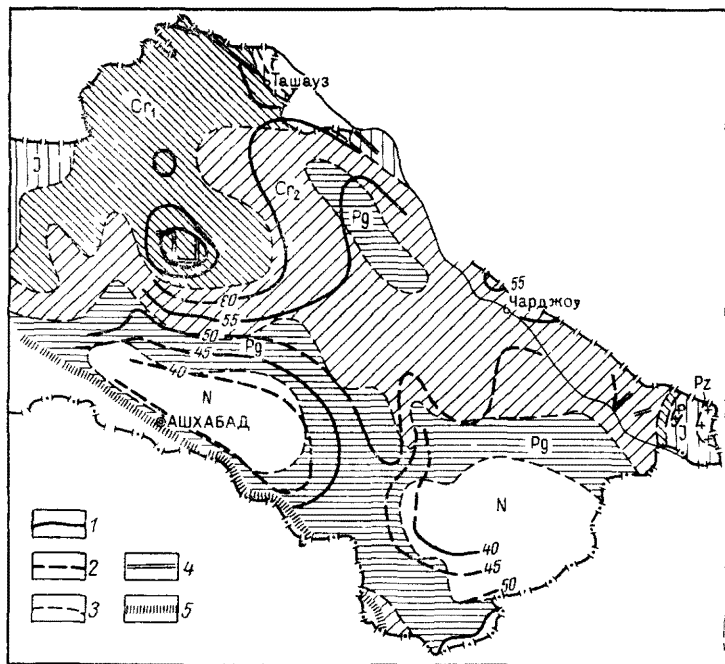
Рис. 38. Схематическая карта геотерм Каракумского артезианского бассейна на глубине 1000 м
