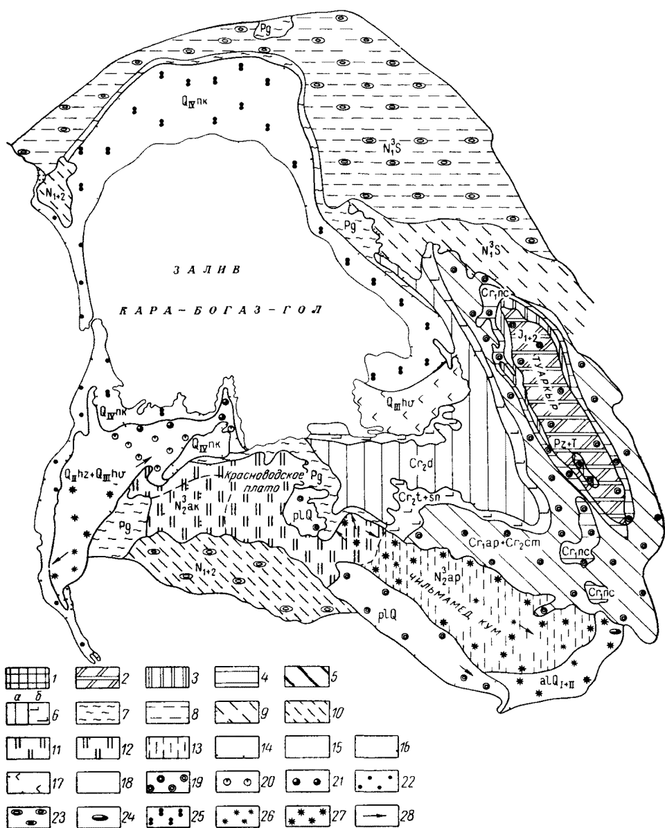
Рис 17 Схематическая гидрогеологическая карта восточной части Среднекаспийского артезианского бассейна
