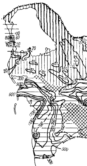
Рис. 13. Схема распределения мощностей четвертичных отложений (по Г. Бердыеву, 1965)
