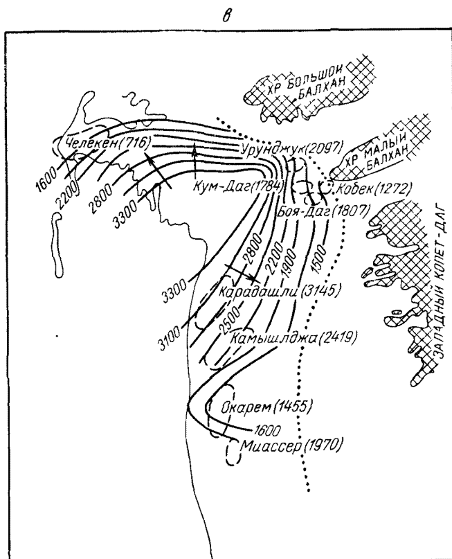
Рис. 25. Схемы гидродинамической обстановки нижней части разреза среднеплиоценовых отложений на начало акачгыльского (а), апшеронского (б) и бакинского (в) времени
