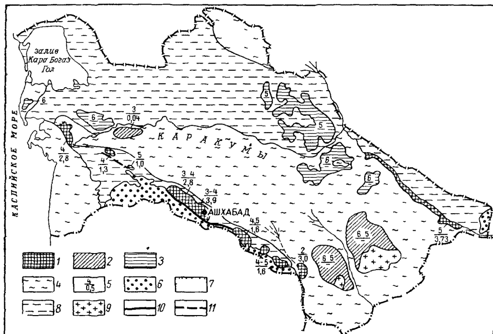
Рис. 53. Схематическая карта прогнозных эксплуатационных запасов пресных и слабосоленоватых подземных вод Туркменской ССР (составила Р. Н. Клышников)
