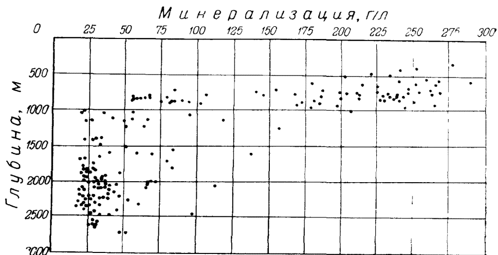
Рис. 21. Зависимость минерализации подземных вод Челекема от глубины залегания
