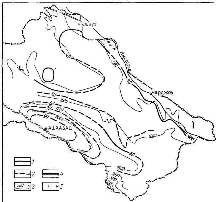
Рис. 39. Схематическая карта геизотерм Каракумского артезианского бассейна по кровле водоносного комплекса верхнемеловых отложений 1 — геизотермы достоверные, 2 — геизотермы предполагаемые; 3 — стратонизогипсы кровли водоносного комплекса, 4 — тектонические нарушения, 5 — граница альпийской геосинклинальной области
