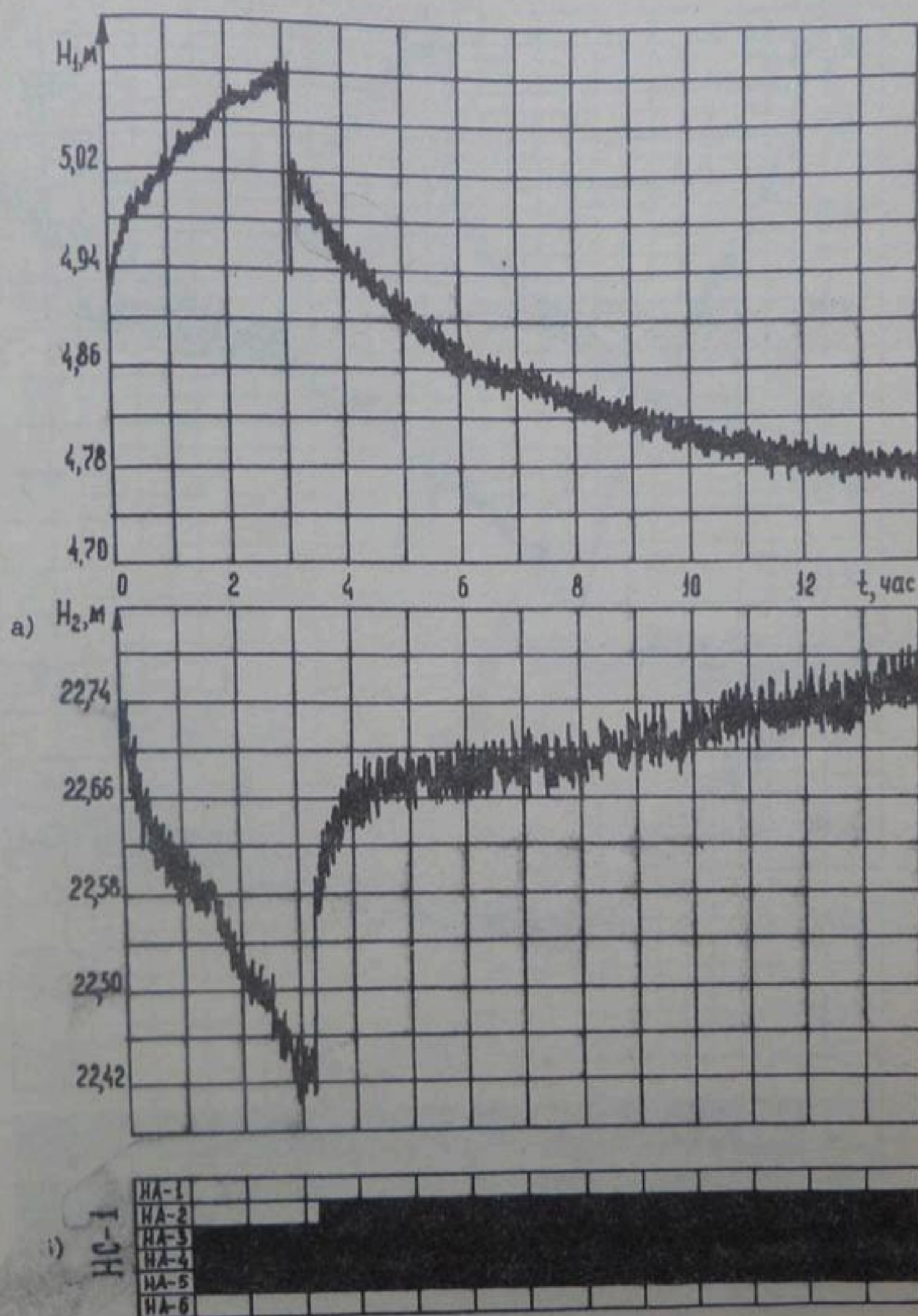
Рис. 2. Изменение режима работы НС-І в первом эксперименте.
