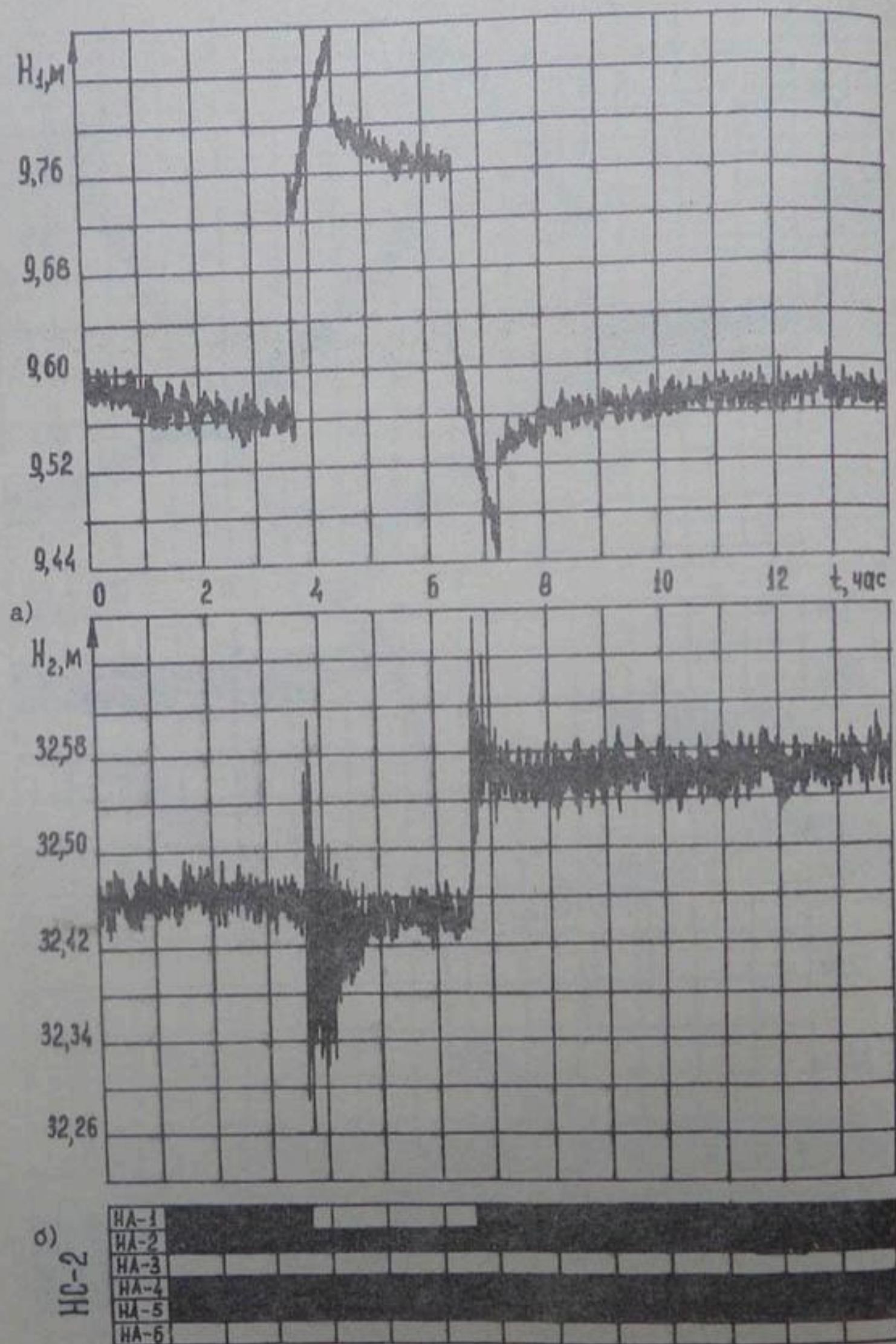
Рис. 5. Изменение режима работы НС-2 во втором эксперименте.
