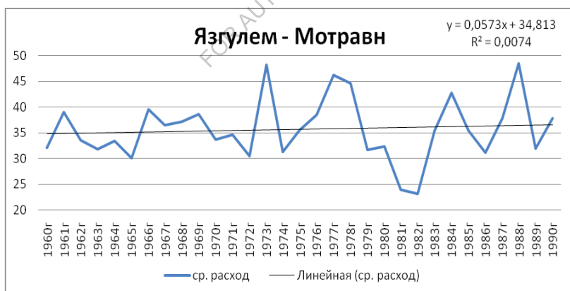
Рис. 4.6. Изменение расходов воды ( \text{м}^3/\text{с} ) на р. Язгулем пост Мотравн за базовый период.
