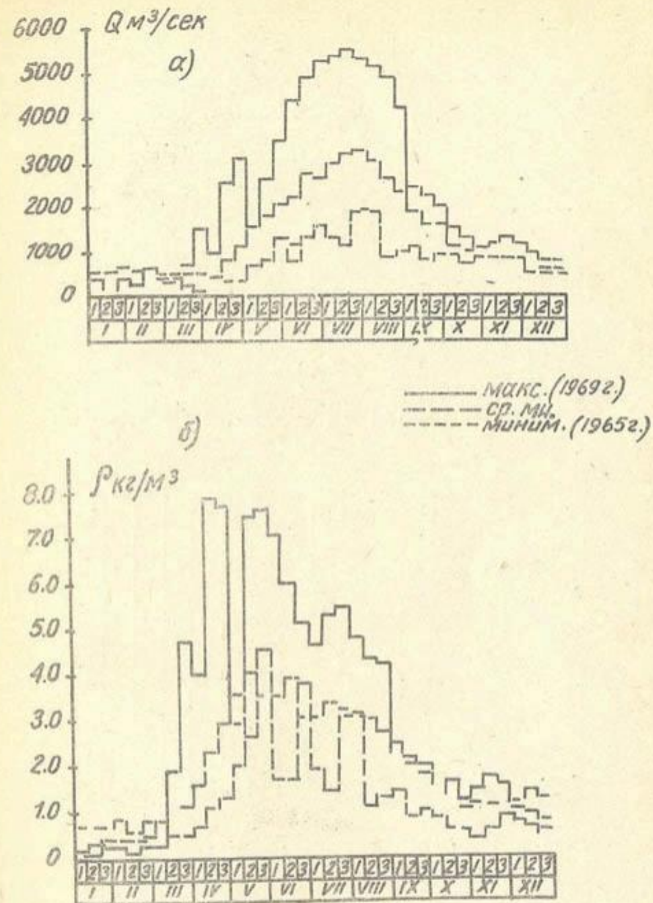
Рис. 3. Гидрографы среднедекадных расходов (а) и мутности (б) воды по створу Чатлы.
