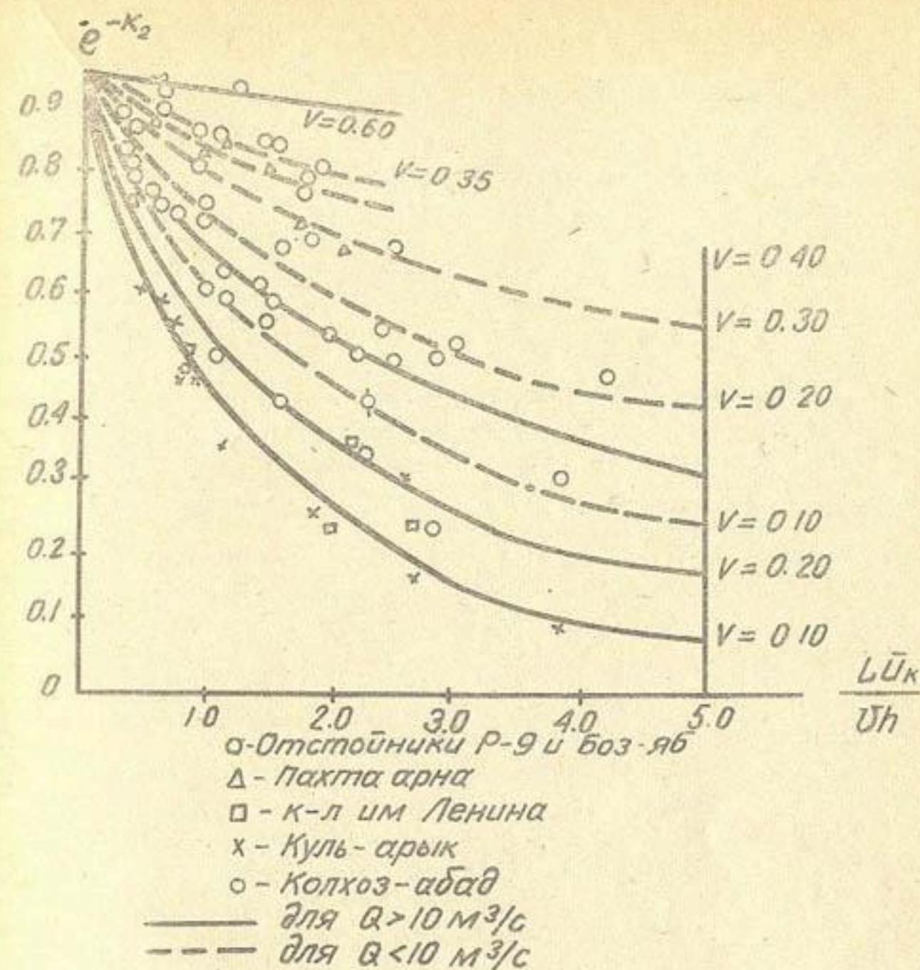
Рис. 17. Зависимость e^{-K_2} = f\left(\frac{lu_k}{vh_{cp}}\right) для фракции наносов (2—0,02) мм/сек.
