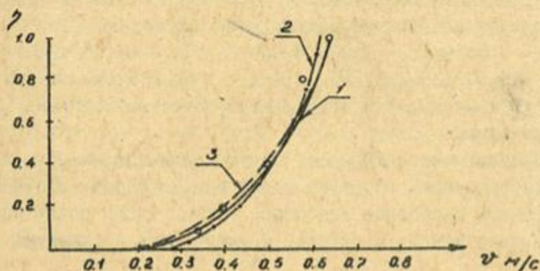
Рис.1. Распределение скорости движения потока по вертикали: о – натурные значения. Расчетные кривые: 1 – по эллиптическому закону; 2 – по логарифмическому закону; 3 – по показательному закону.
