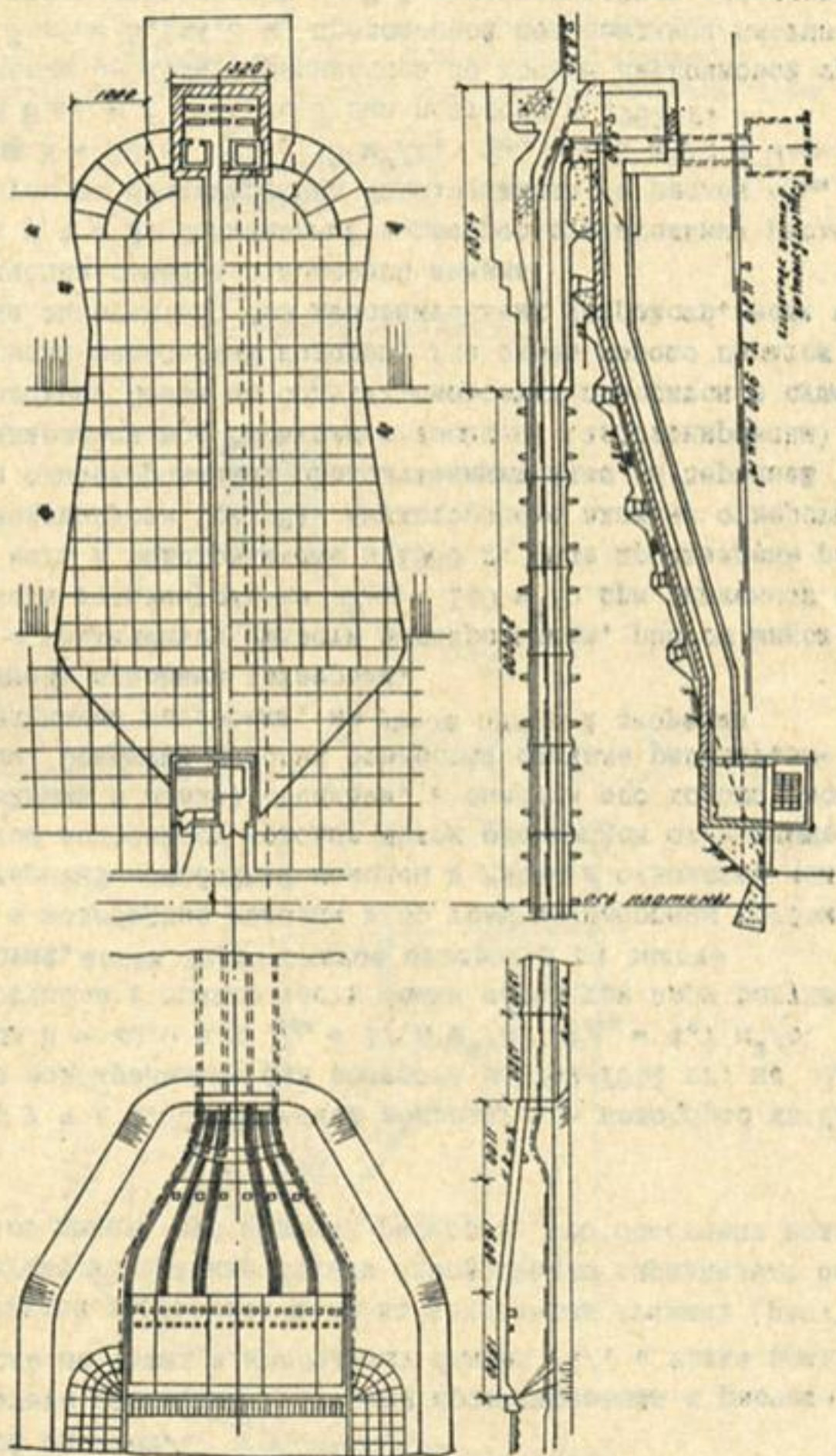
Рис. 8. Реконструкция входной части водопуска-водосброса Каттекур- танского водохранилища. Пунктиром показана удаленная башня управления, а заштрихованное - изменения при рекон- струкции сооружения.
