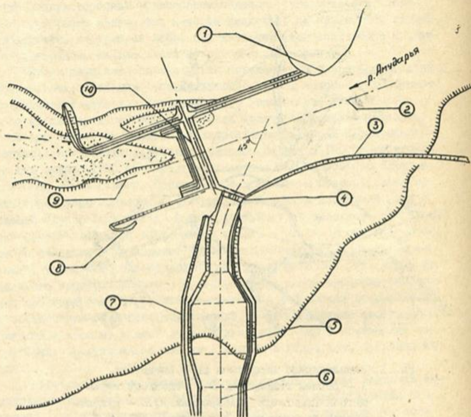
Рис.2. Компоновка речного гидроузла: 1 – скальный мыс; 2 – ось подводющего канала; 3 – струенаправляющая дамба; 4 – водозаборное сооружение; 5 – земляная плотина; 6 – соединительный канал; 7 – отстойник; 8 – дамба отводящего канала; 9 – отводящий канал; 10 – водосборная плотина.
