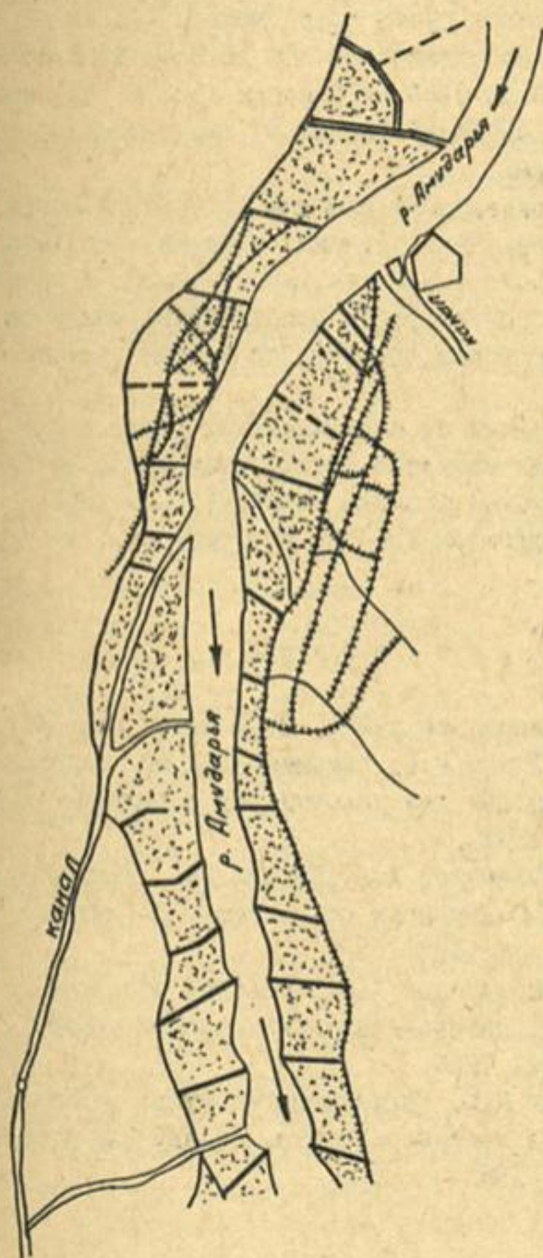
Рис. I. План участка р. Амударья в районе каналов Ташсак - Пактаврна, за-регулированного траверсными дам-бами.
