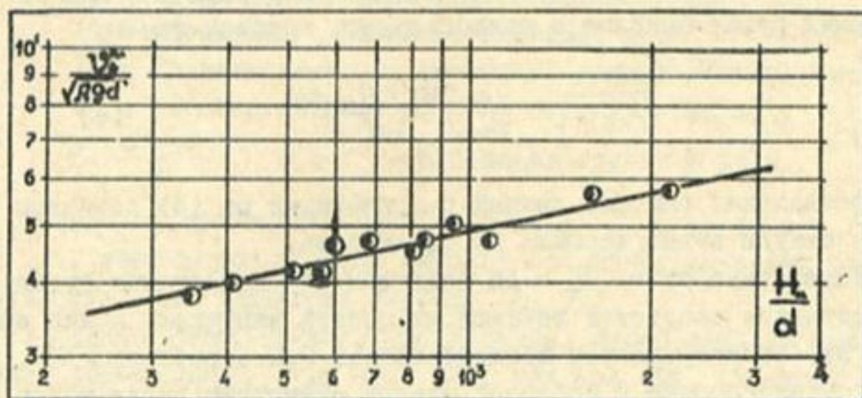
Рис.2. Сопоставление расчетных значений неразмывающей скорости по формуле (5) с опытными данными в условиях плоской задачи.
