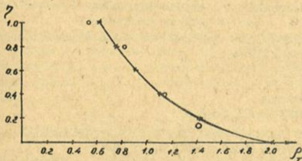
Рис.2. Распределение мутности потока по вертикали: о – натурные значения; х – расчетные значения по формуле (6).
