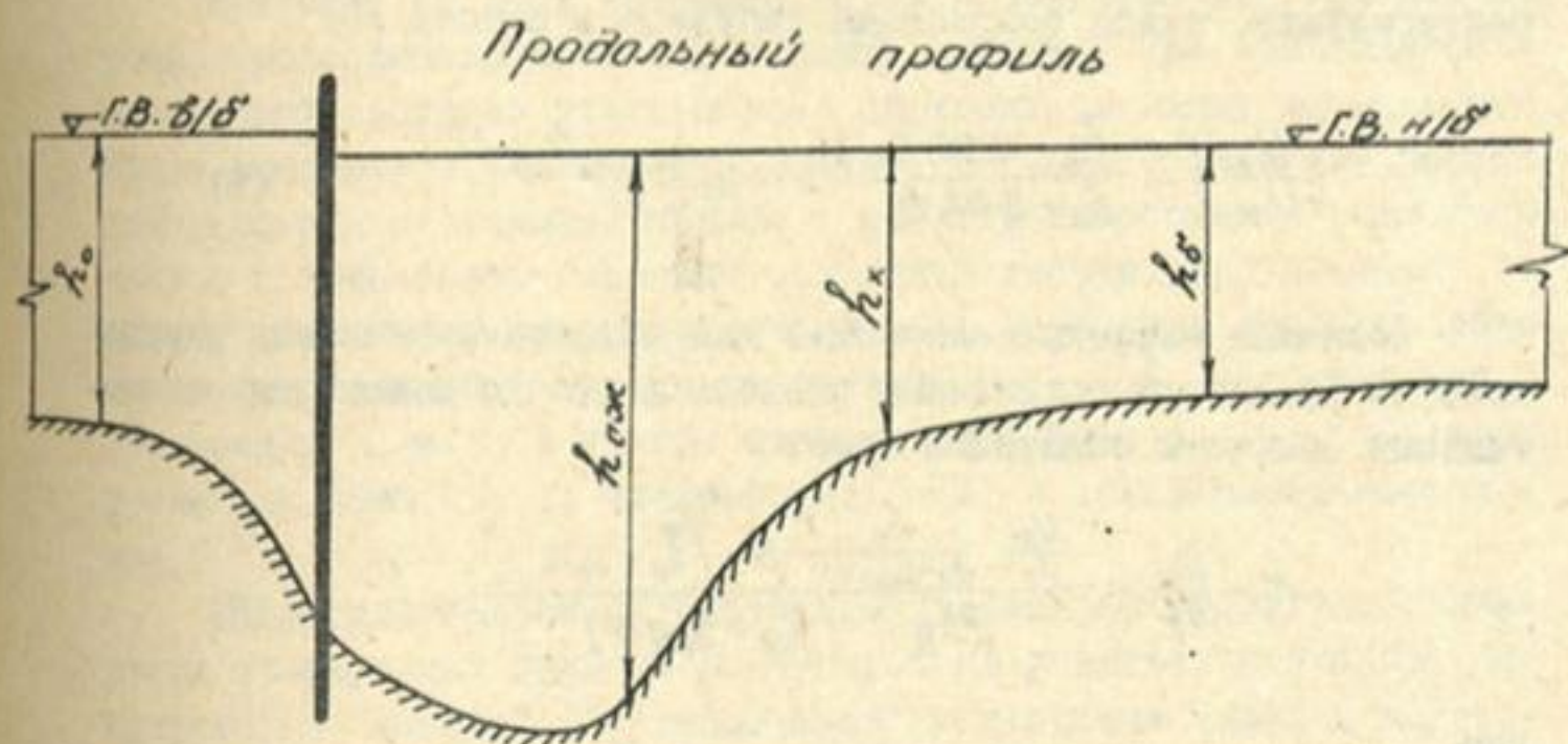
Расчетная схема растекания потока за дамбами.
