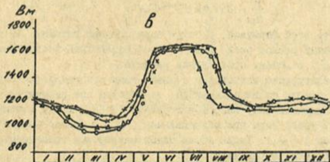
Рис.2. Графики зависимости уровня воды (а), глубины (б), ширины (в) потока от времени р.Оби с.Белогорье и р.Иртыша с.Ханты-Мансийск: .... - 1971, -о-о- 1972; + + - 1973; Δ-Δ - 1974, п-п-п- 1973 и 1974 р.Иртыш.
