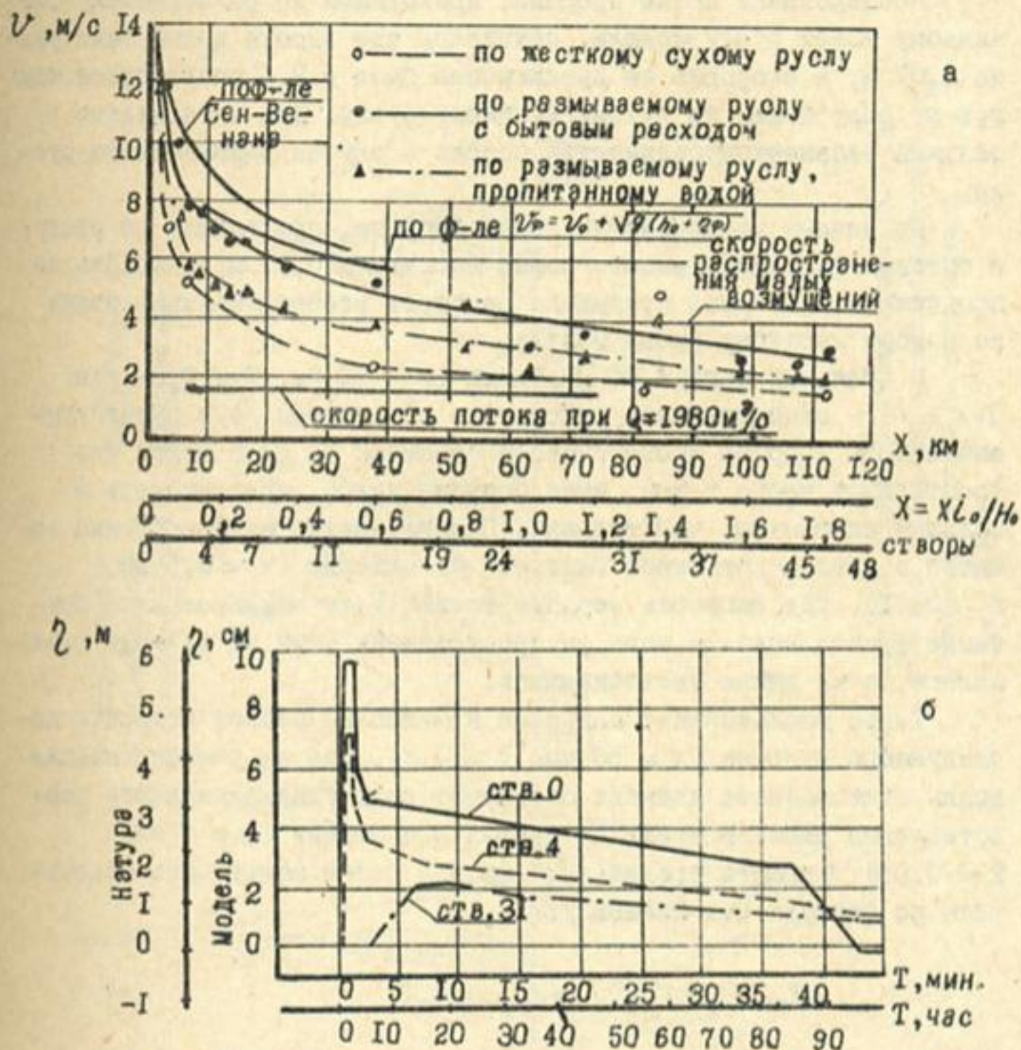
Рис. 1. Трансформация волны прорыва вдоль участка исследований ( B_{\text{пр}} = 250 \text{ м} ): а — изменение скорости распространения фронта волны (пересчет на натуру); б — изменение приращений уровней воды при прохождении волны над бытовыми по времени в различных створах (при прохождении волны по размываемому руслу с бытовым расходом).
