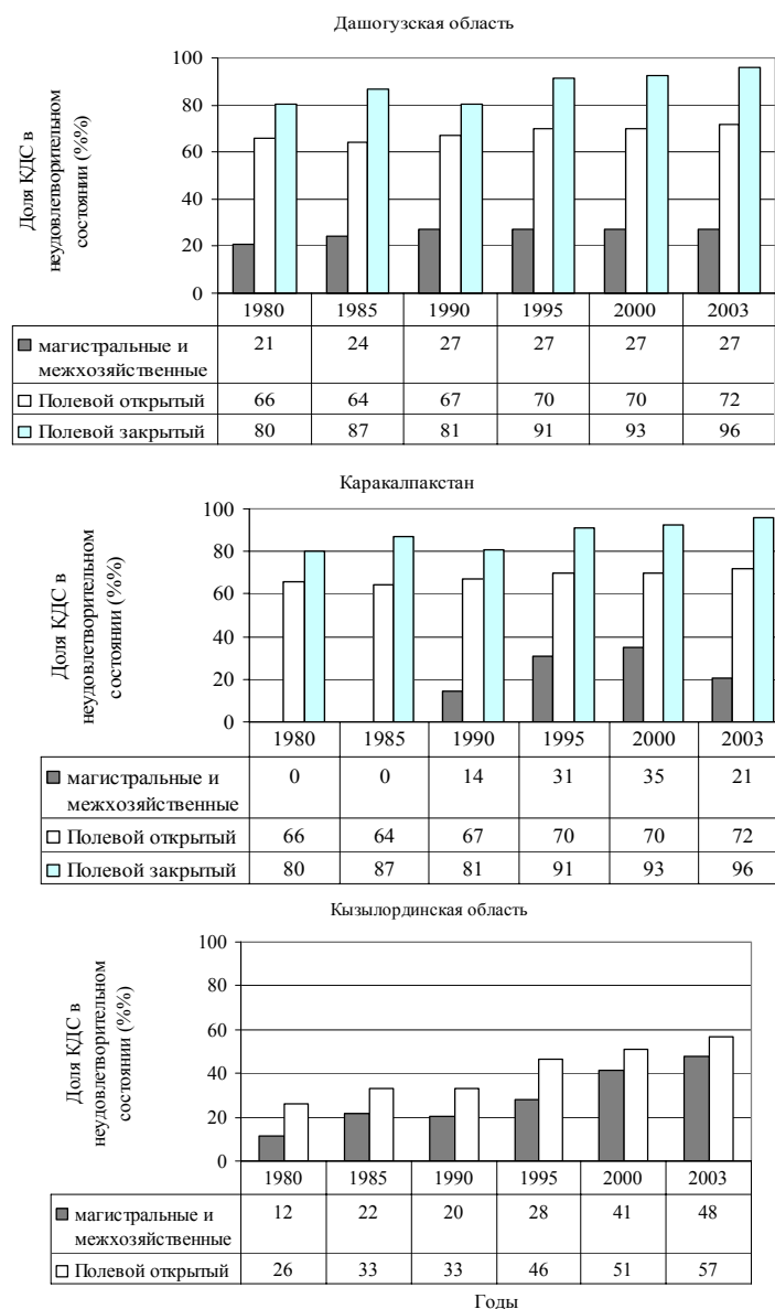
Рис.1.6.5. Состояние дренажа
