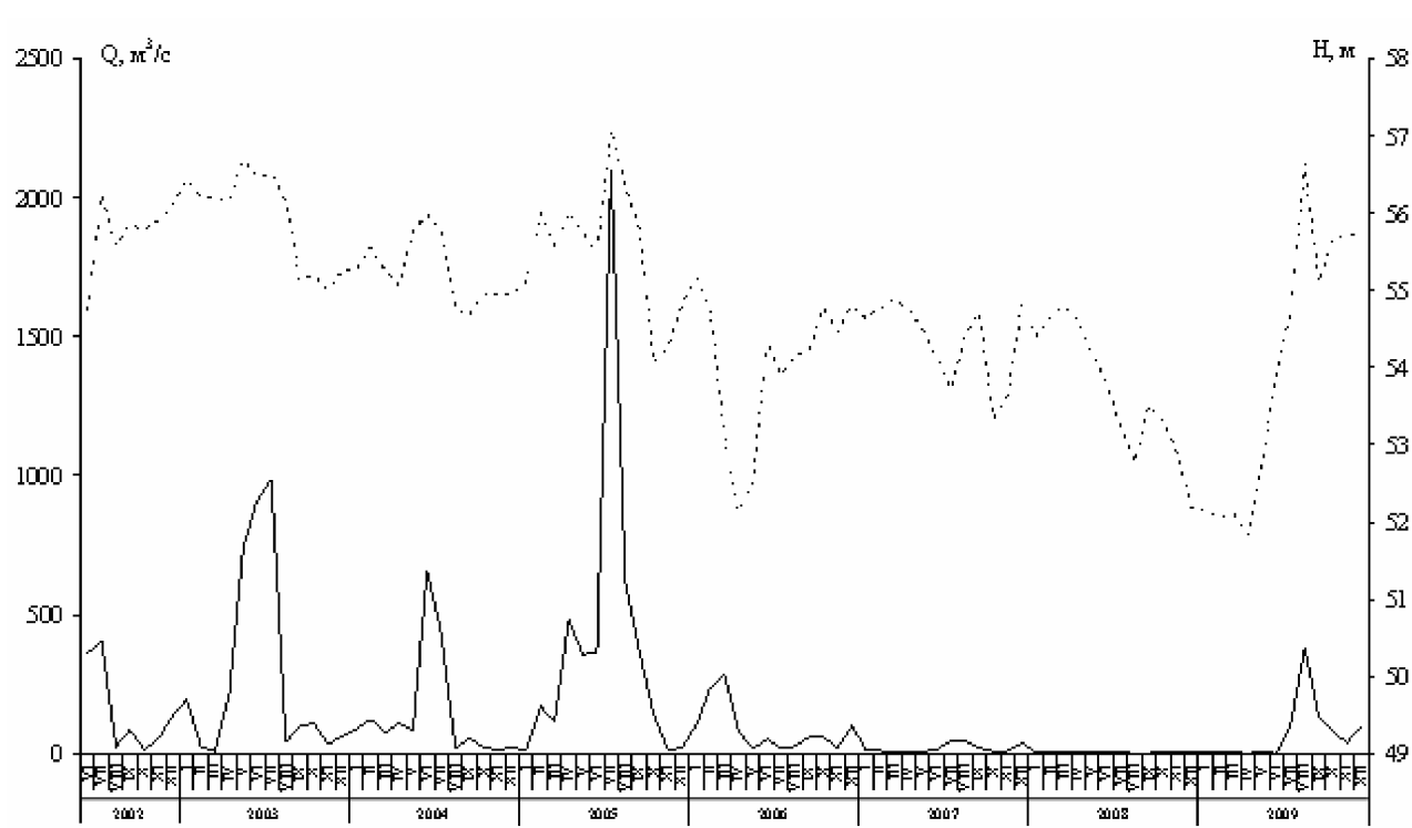
Рисунок 5.18 - Совмещенные графики расхода воды по ств. Кызылджар и уровня воды Междуреченского водохранилища за период с 2002 по 2009 гг. — Q , — H
