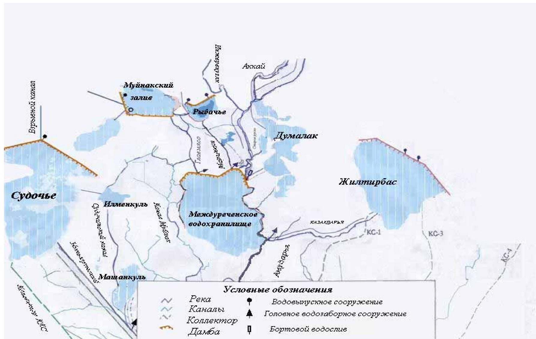
Рисунок 5.6 Карта расположения гидротехнических сооружений в дельте реки Амударьи
