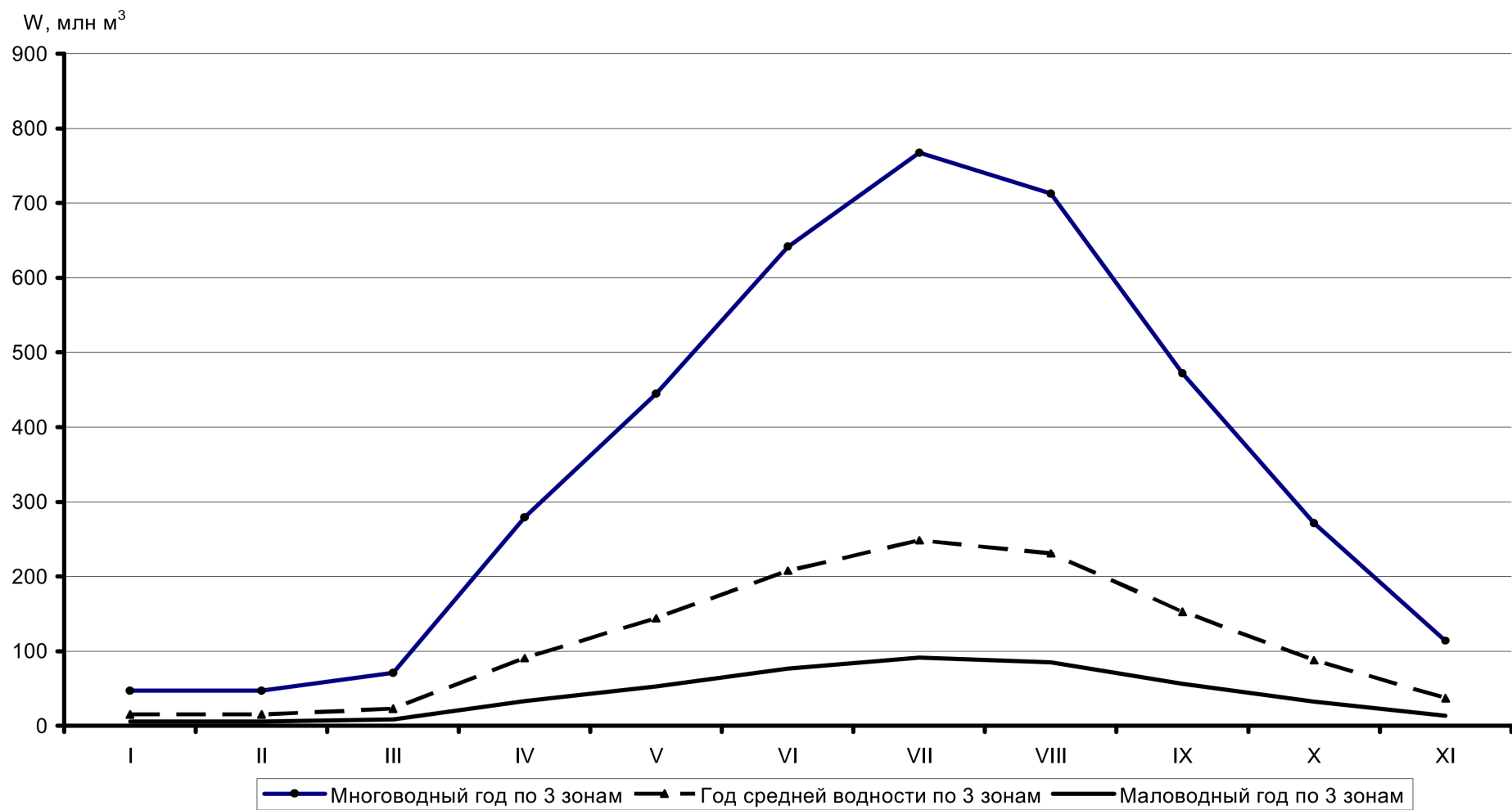
Рисунок 5.5 График объема водоподачи для обводнения дельтовых озер в годы различной обеспеченности
