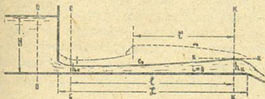
Рис. I. Формы кривых свободной поверхности потока в лотке за щитовым отверстием перед перепадом.
