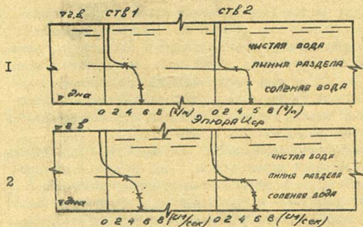
Рис. 2. 1-Эпюры минерализации и 2-средней скорости по сечению (по вертикали) плотного потока расход минерализованной воды Q=1,5 л/с концентрация M=5 г/л)
