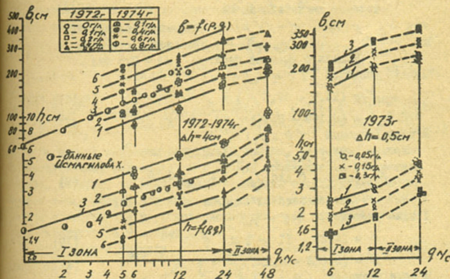
Рис. График сопоставления результатов расчета по зависимостям (6)+(12) с лабораторными данными.
