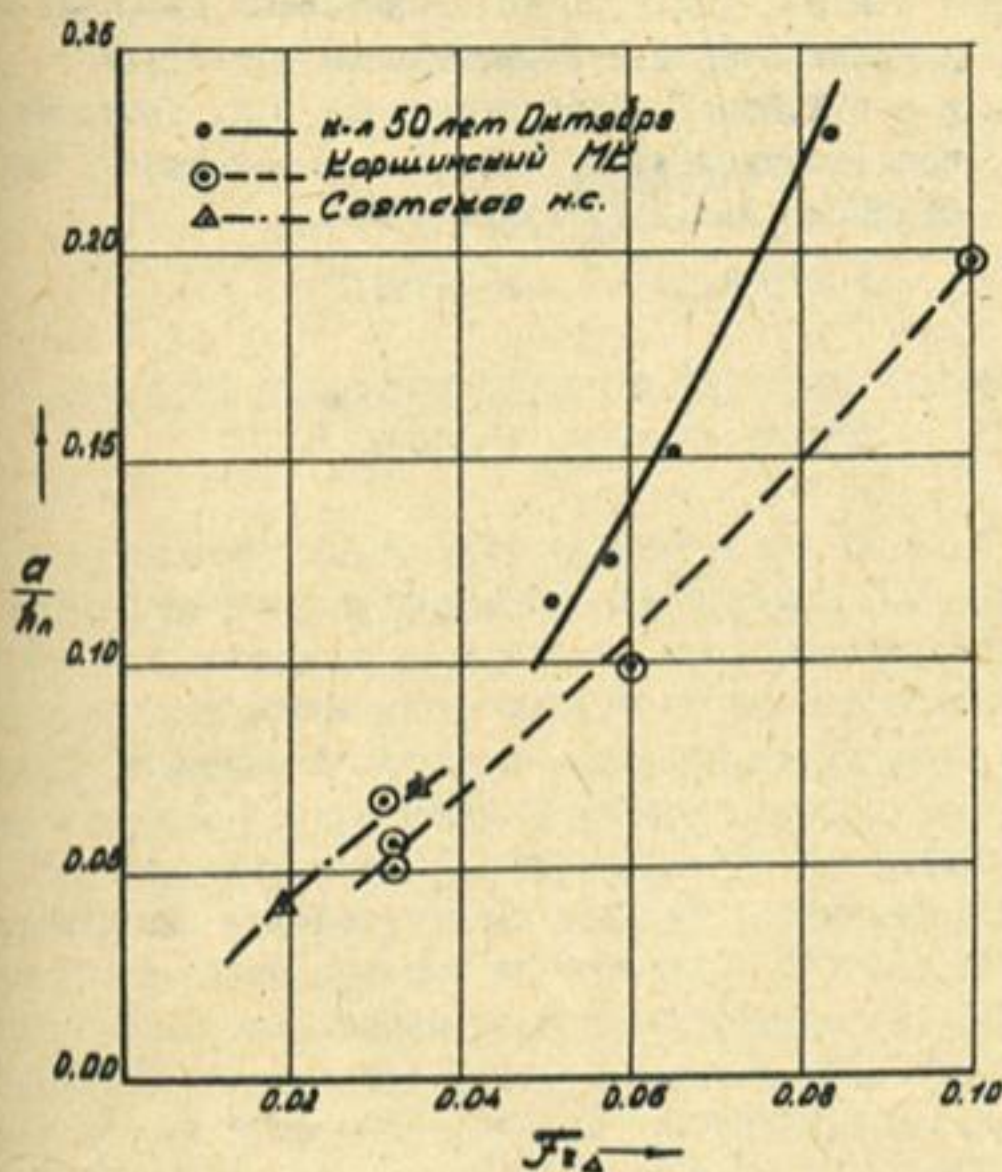
График зависимости a_1/h_n = f(Fr_{\Delta}) для каналов ( a — высота максимального гребня волны).
