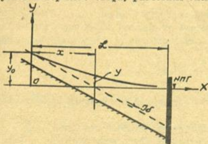
Рис.1. Схема к расчету кривой подпора в заносимых верхних бьефах гидроузлов.
