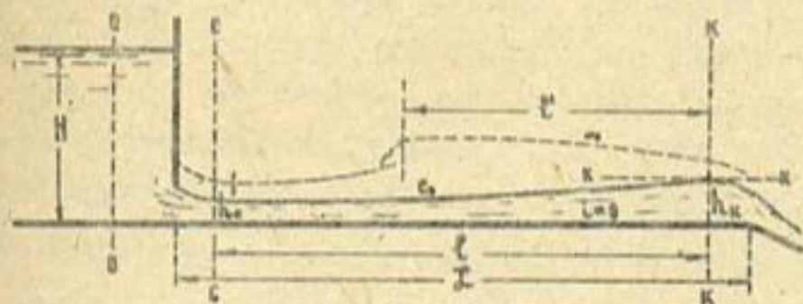
Рис. I. Формы кривых свободной поверхности потока в лотке за щитовым отверстием перед перепадом.
