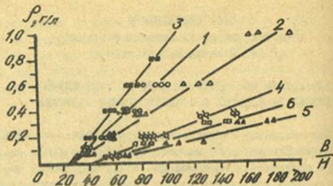
Рис. 2. График изменения относительной ширины русла по данным лабораторных исследований моделей с мелкопесчаными наносами 1972 г. ( \Delta h = 4 см): 1—6, 12 л/с; 2—24 л/с; 3—48 л/с; 1973 г. ( \Delta h = 0,5 см): 4—6 л/с; 5—12 л/с; 6—24 л/с.
