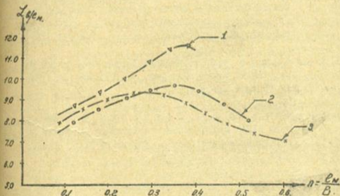
Рис. 2. График Z/\epsilon_n = f(\eta) : 1 — по Бакиеву М.Р. и др.; 2 — по автору (метод ЭГДА); 3 — по Баланину В.В. и др.
