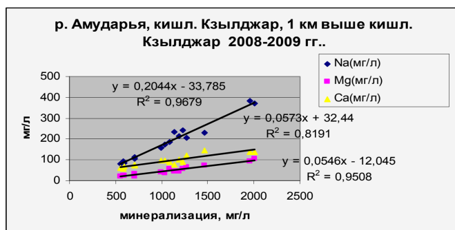
Рисунок 4.6 -Графики зависимости содержания главных ионов (Ca, Mg, Na, HCO 3 , Cl, SO 4 ) от величины минерализации на различных створах р. Амударьи.
