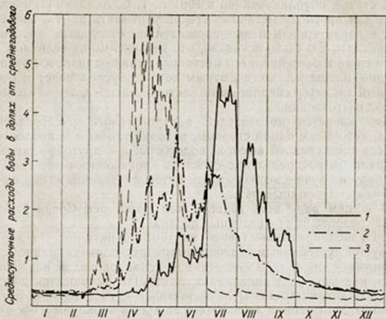
Рис. 56. Гидрографы рек за 1956 г. 1 — Сух, 2 — Чирчик, 3 — Ангрен.
