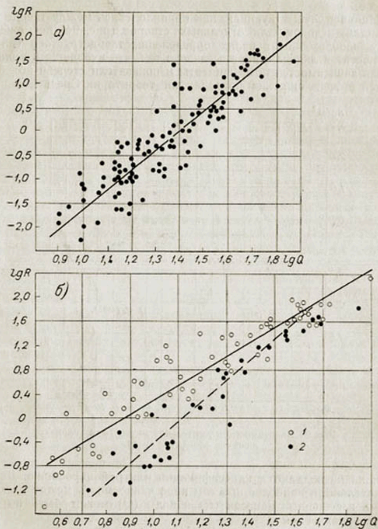
Рис. 94. Зависимость между расходами взвешенных наносов ( R ) и расходами воды ( Q ). а — р. Исфайрам — ст. Учкурган, б — р. Исфара — ст. Ташкурған. 1 — апрель—июль, 2 — август—сентябрь.
