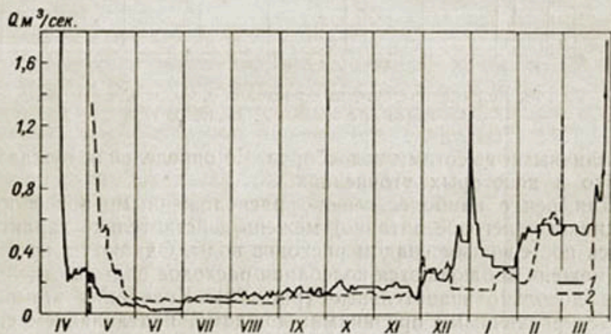
Рис. 81. Ход средних суточных расходов воды р. Кичик-Уру в межень.
