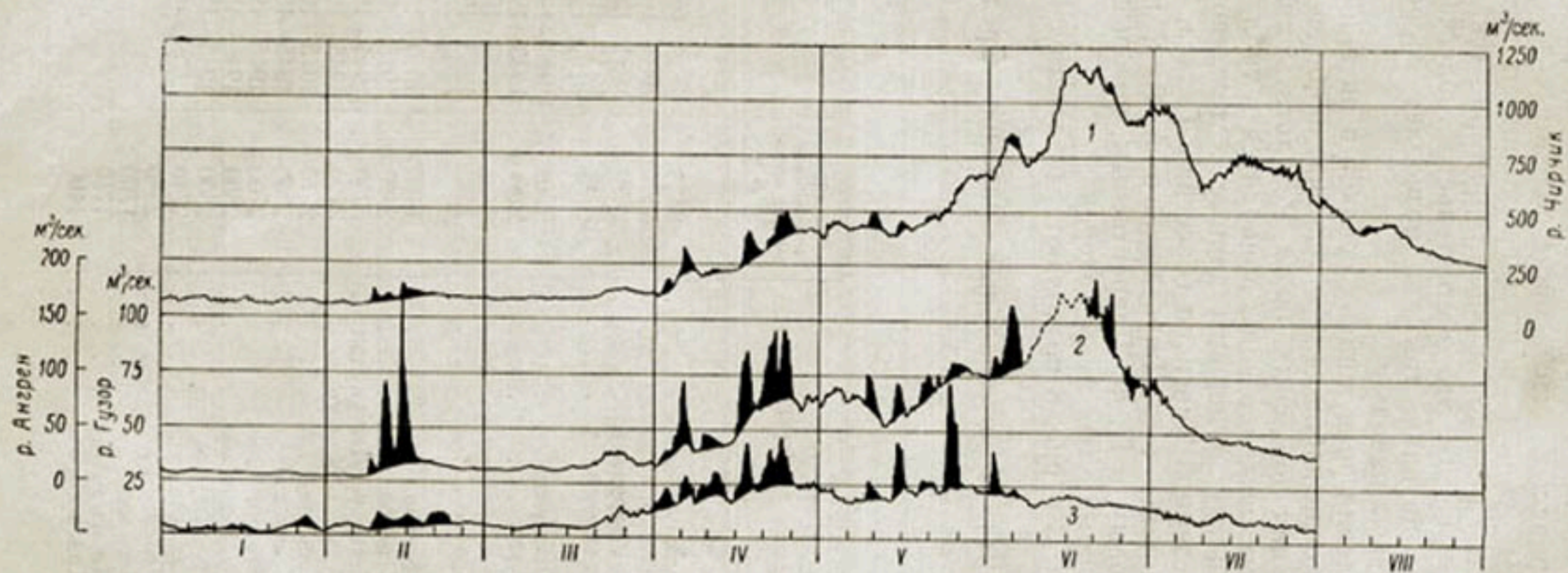
Рис. 8. Ход срочных расходов воды за 1933-34 г. с выделением дождевого питания. 1 — р. Чирчик — ст. Ходжикент, 2 — р. Ангрен — ст. Турк, 3 — р. Гузар — ст. Яркен.
