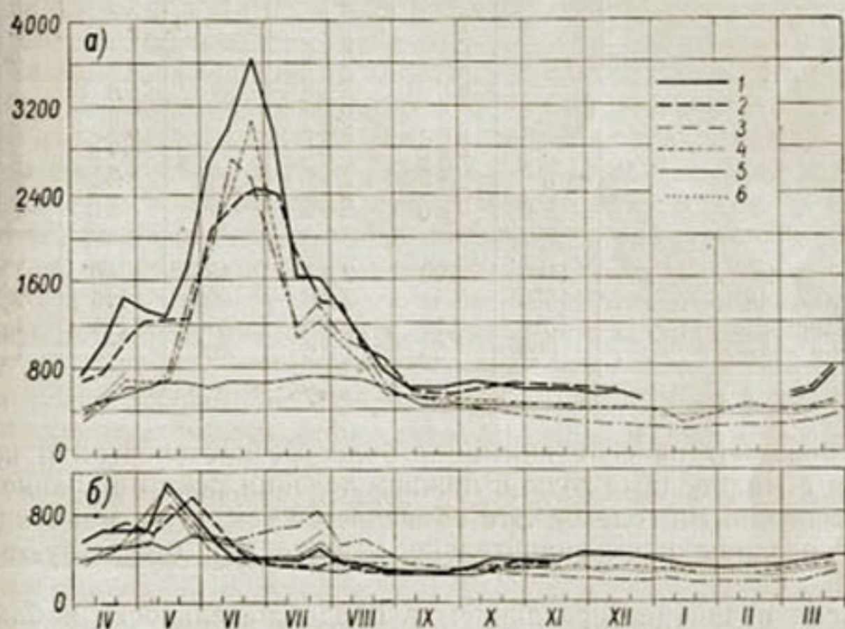
Рис. 147. Ход средних декадных расходов воды Сыр-Дарьи. а — 1934-35 г., б — 1938-39 г. 1 — Кокбулак, 2 — Тюменьарык, 3 — Учкуртан и Кампыррават (суммарные), 4 — Беговат, 5 — Казалинск, 6 — Каль.
