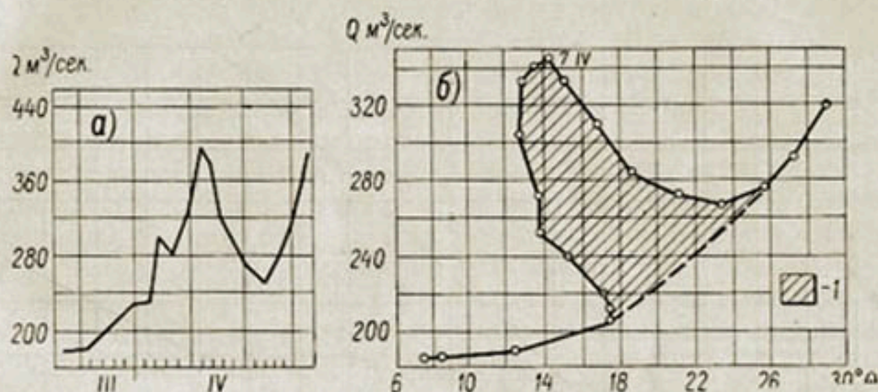
Рис. 13. Гидрограф средних суточных расходов р. Нарын — ст. Учкур- гун (а) и зависимость средних суточных расходов от температу- ры воздуха за 13 час. по ст. Андижан для скользящих пентад (б). Март—апрель 1936 г. I — дождевой сток.
