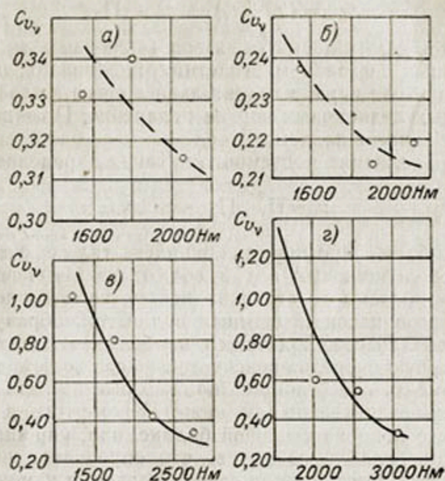
Рис. 27. Зависимость изменчивости водности снежного покрова ( C_{v_v} ) от высоты местности ( H ). а — р. Чаткал, б — Падшаата, в — р. Қарадарья, г — Исфайрам.
