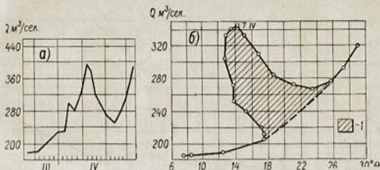
Рис. 13. Гидрограф средних суточных расходов р. Нарын — ст. Учкурган (а) и зависимость средних суточных расходов от температуры воздуха за 13 час. по ст. Андижан для скользящих пентад (б). Март—апрель 1936 г.
