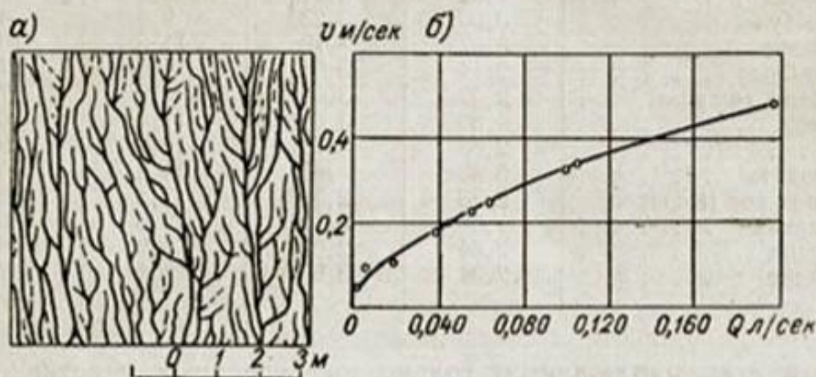
Рис. 76. Густота микроручейковой сети (а) и зависимость скоростей стекания (б) от величины расходов на эродированном склоне крутизной 32^\circ .
