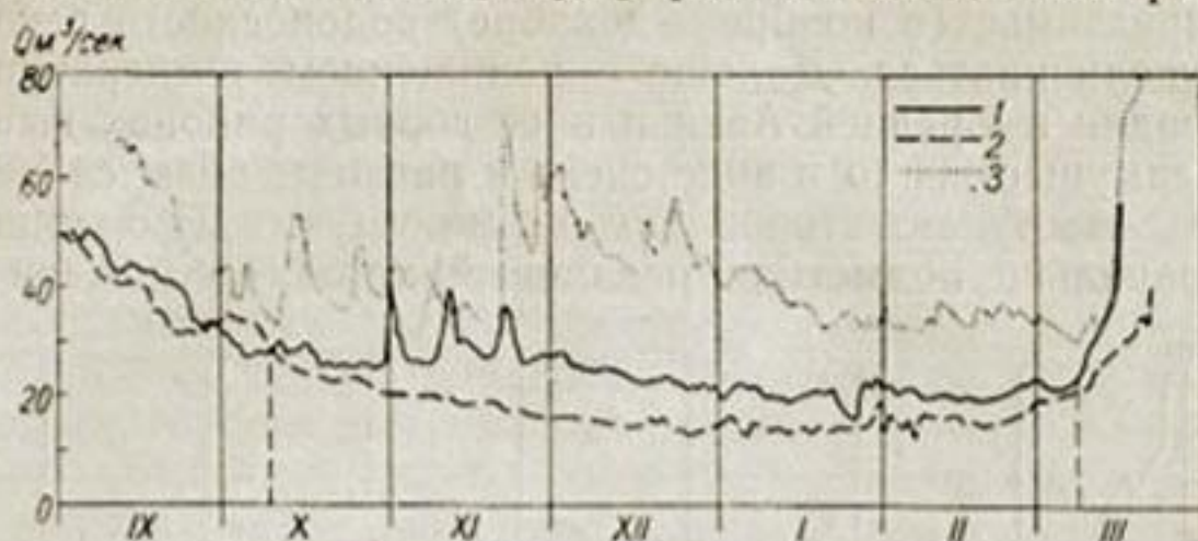
Рис. 80. Ход средних суточных расходов воды р. Кафирниган в межень.
