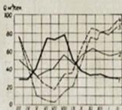
Рис. 161. Ход средних месячных расходов воды р. Чу в 1940-41 г. 1 — с. Джильярык, 2 — с. Чумыш, 3 — с. Ташуткул, 4 — с. Фурмановка.
