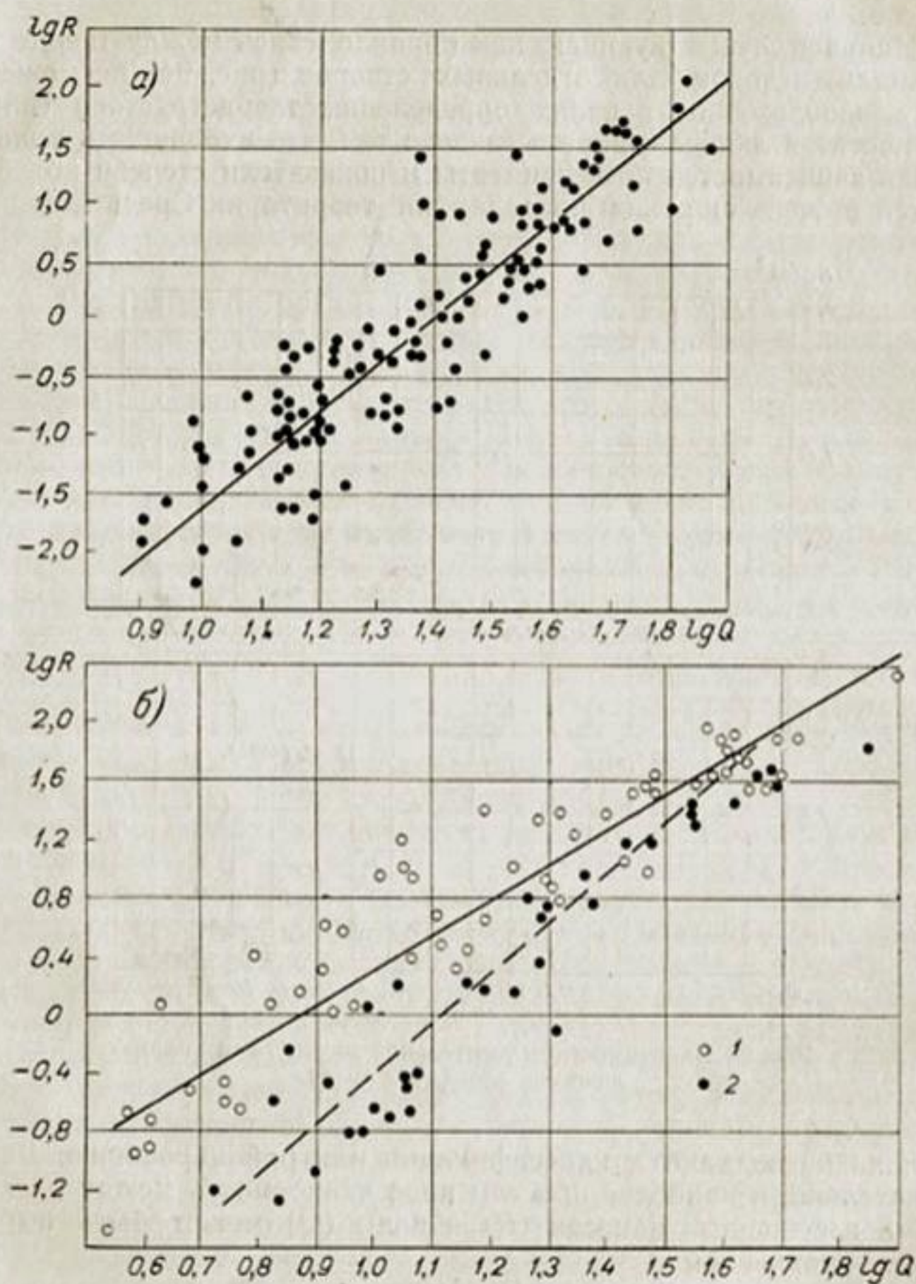
Рис. 94. Зависимость между расходами взвешенных наносов ( R ) и расходами воды ( Q ). а — р. Исфайрам — ст. Учкурган, б — р. Исфара — ст. Ташкуртан. 1 — апрель-июль, 2 — август-сентябрь.
