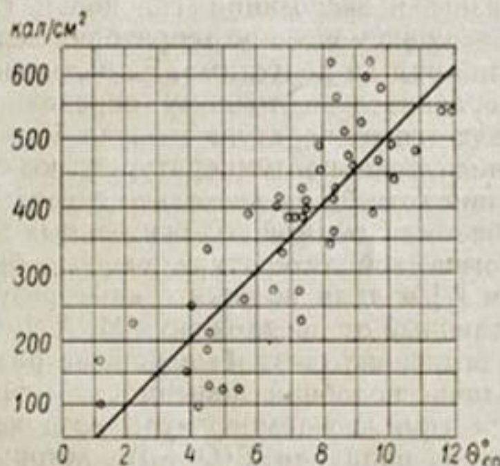
Рис. 43. Зависимость между приходом тепла и средними суточными температурами воздуха ( \theta ).
