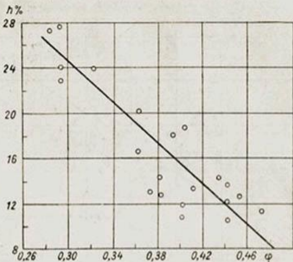
Рис. 84. Зависимость долей межени в годовом ( h ) от коэффициента внутригодовой неравномерности стока ( \phi ) для южного района Средней Азии.
