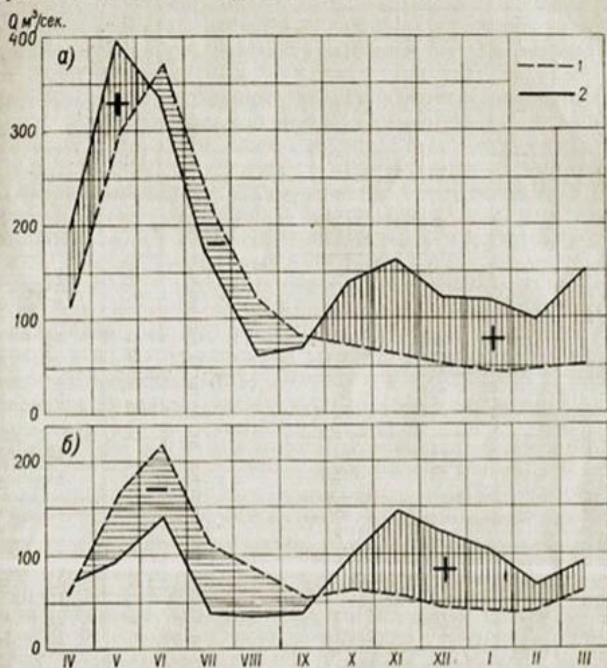
Рис. 143. Ход средних месячных расходов воды р. Карадарья в створах Кампырраватской (1) и Балыкчинской (2) станций. а — многоводный 1937-38 г., б — маловодный 1940-41 г.
