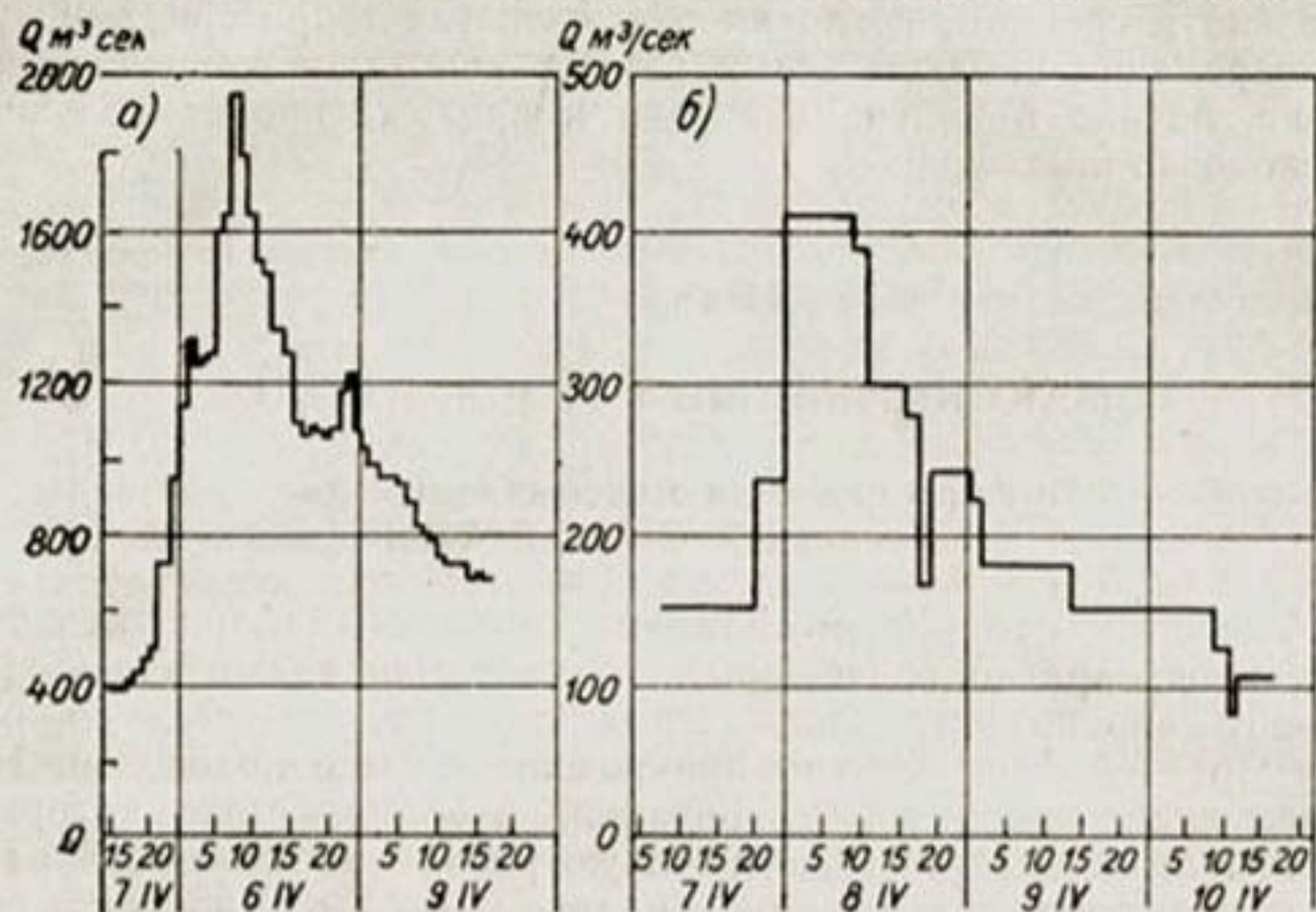
Рис. 71. Гидрографы паводков, прошедших в апреле 1959 г. а — р. Чирчик, б — р. Ангрен.
